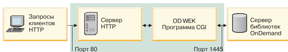
Рисунок 2. Один экземпляр с интерфейсом CGI
