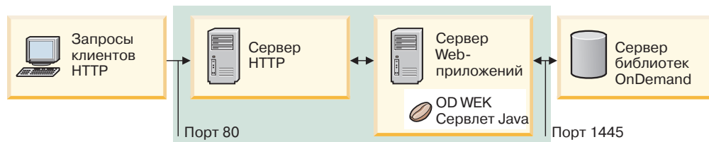
Рисунок 3. Один экземпляр с интерфейсом Java
