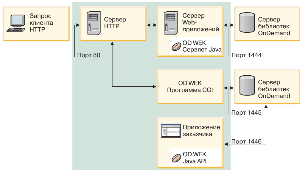
Рисунок 5. Топология с несколькими экземплярами
