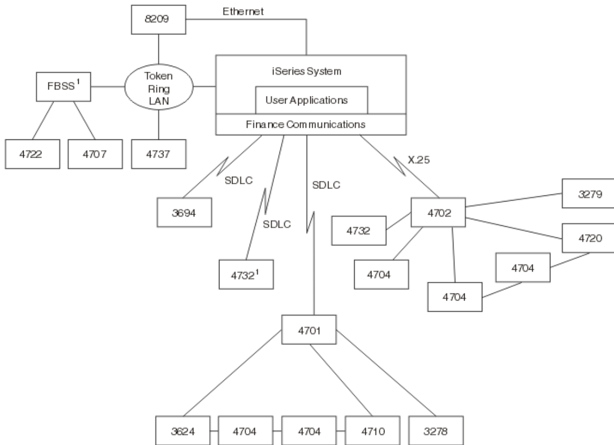
Figuur 10. Een iSeries-server met een Finance-netwerk
