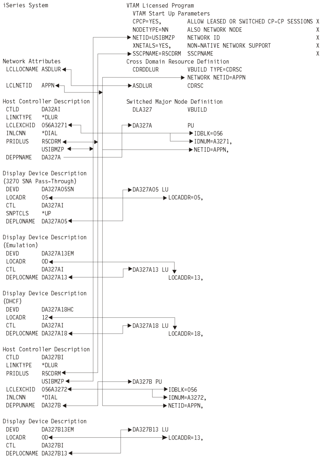
Figuur 4. iSeries-server via APPN-verbinding met VTAM
