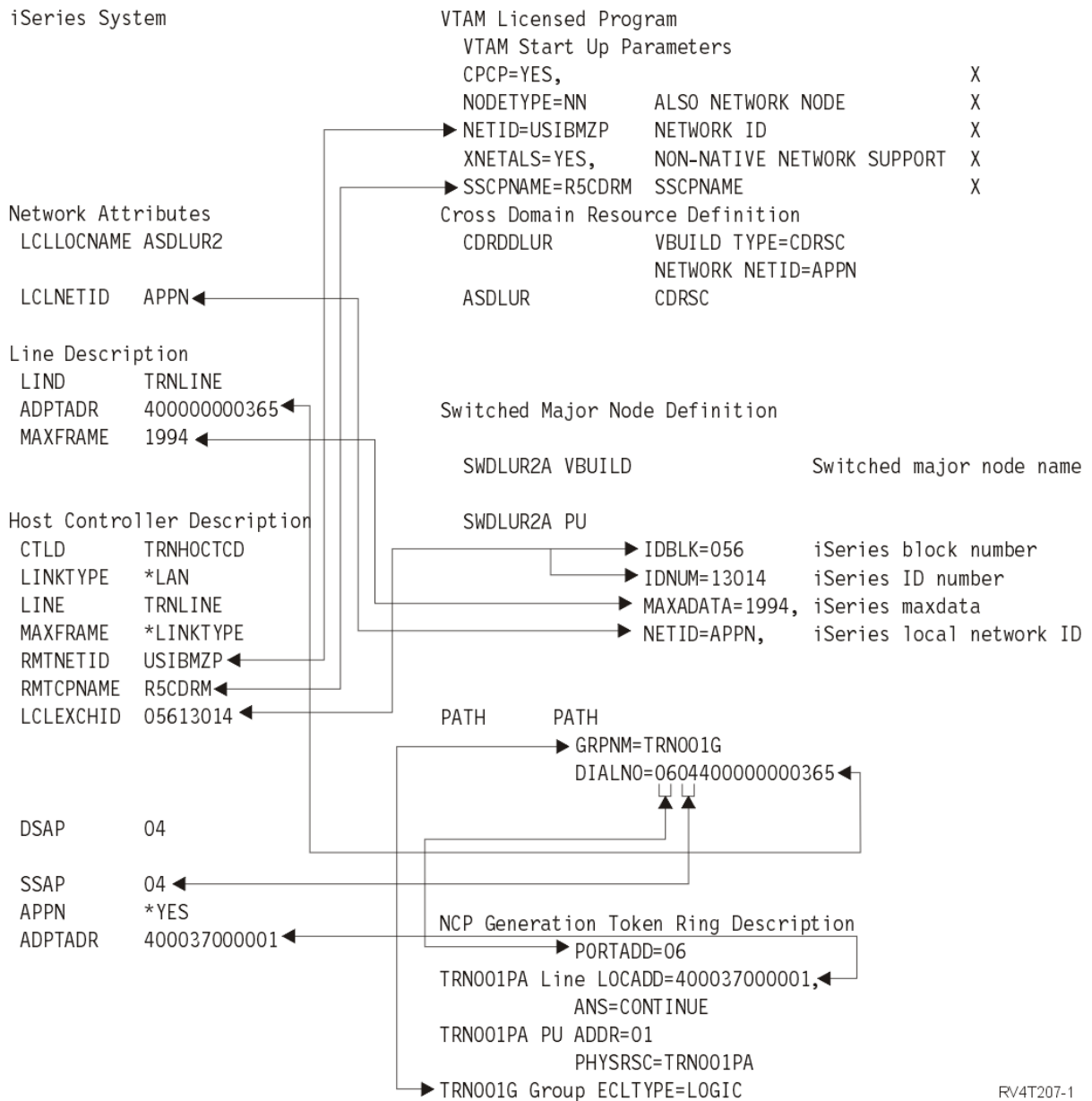
Figuur 3. iSeries-systeem met DLUR-ondersteuning verbinden met een hostsysteem
