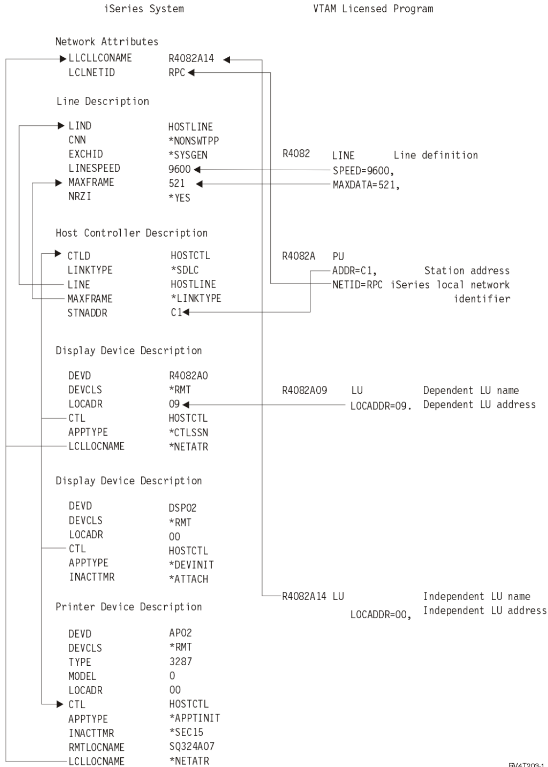
Figuur 1. iSeries-systeem verbinden met een hostsysteem via een vaste SDLC-lijn
