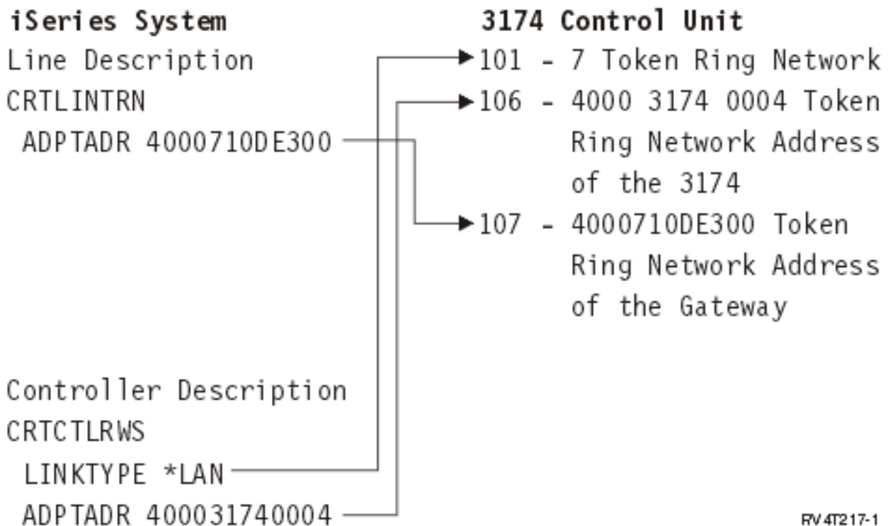
Figuur 9. Een iSeries-server met een 3174-controller
