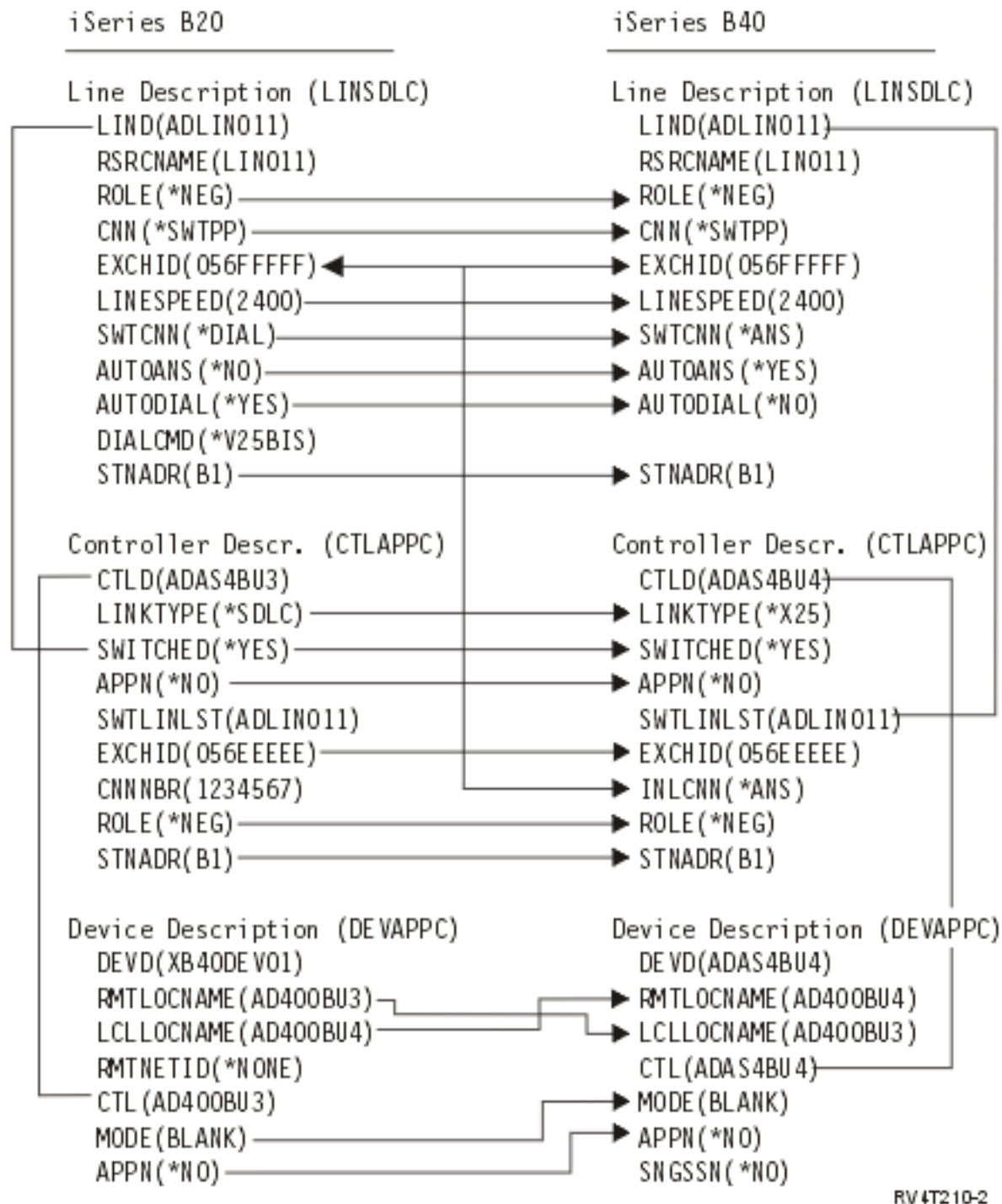
Figuur 7. Series-server met iSeries-server met automatisch kiezen in één richting
