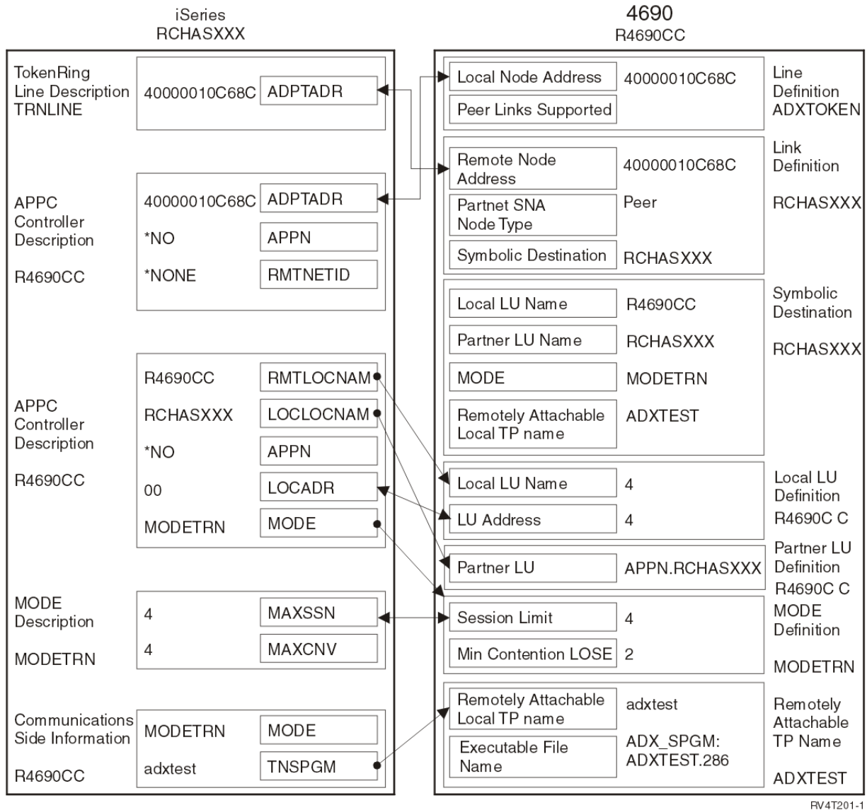
Figuur 12. iSeries-server met 4690-peer via een token-ring-netwerk
