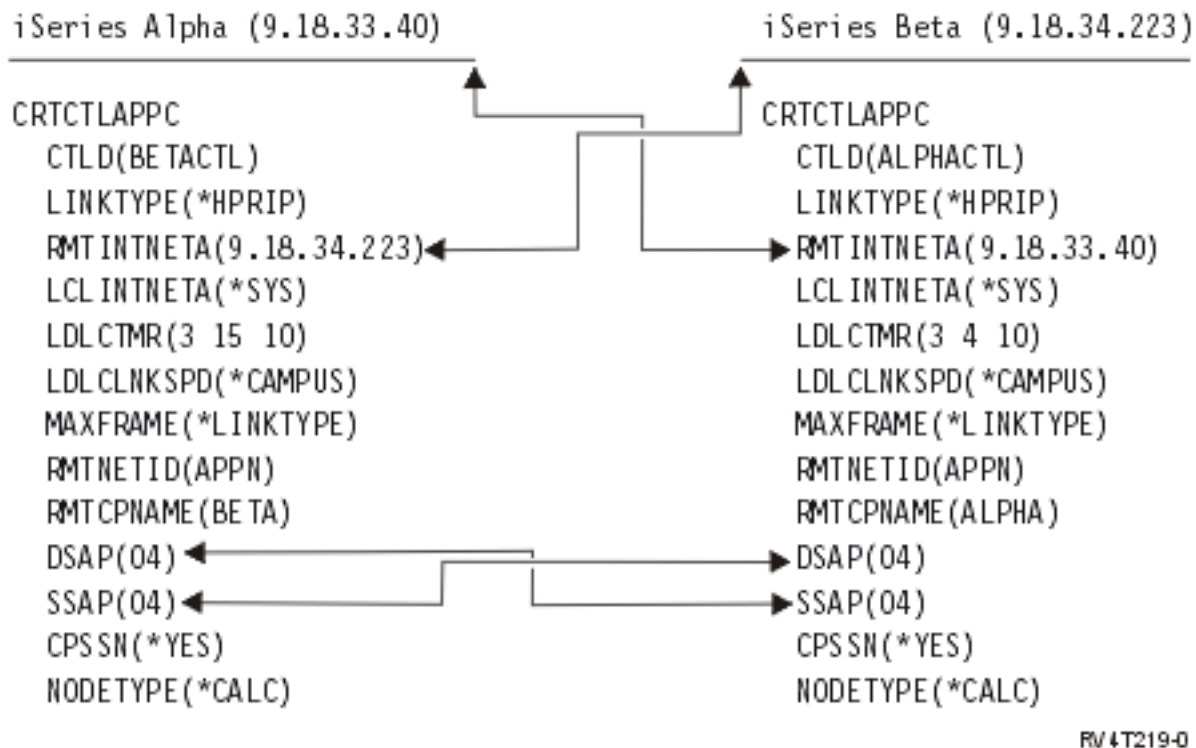
Figuur 8. iSeries-server met iSeries-server met Enterprise Extender (HPRIP)
