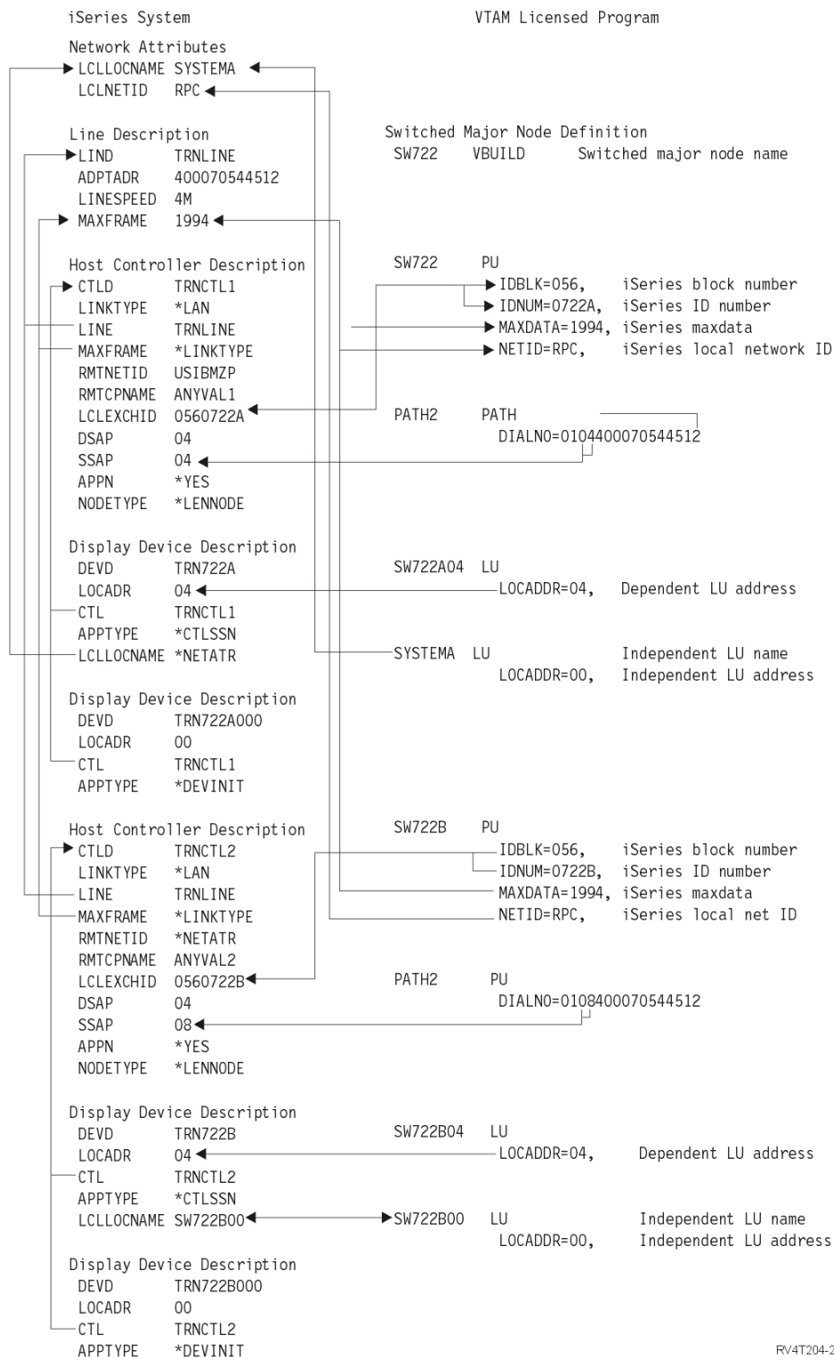
Figuur 2. iSeries-systeem verbinden met een hostsysteem via een token-ring-lijn
