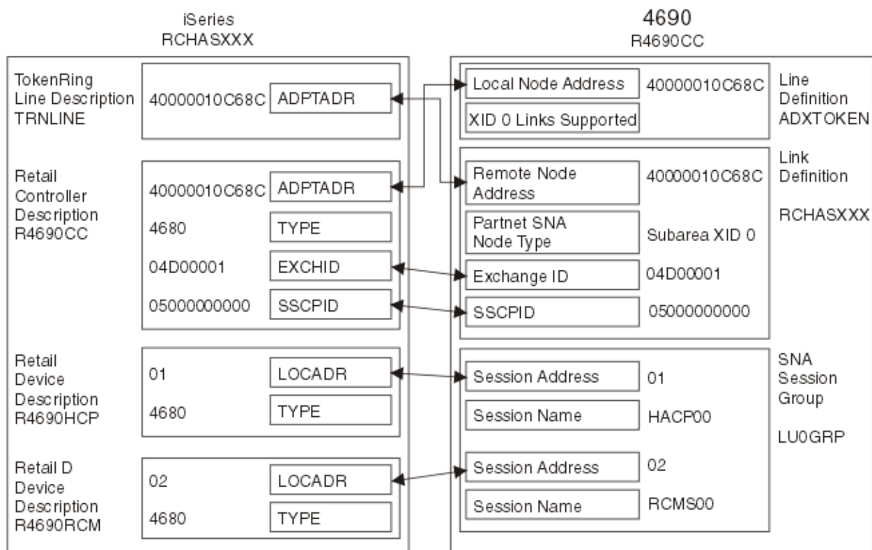
Figuur 11. iSeries-server met 4690 LU0 via een token-ring-netwerk
