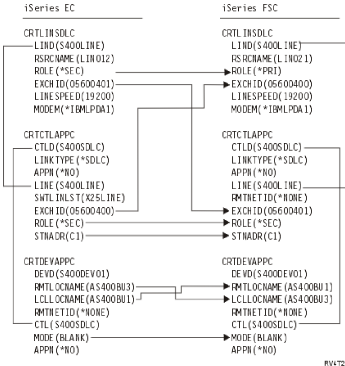
Figuur 6. iSeries-server met iSeries-server met SDLC
