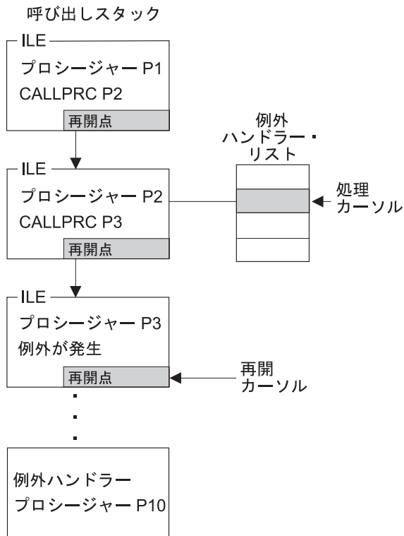
図 45. 処理カーソルおよび再開カーソルの例
