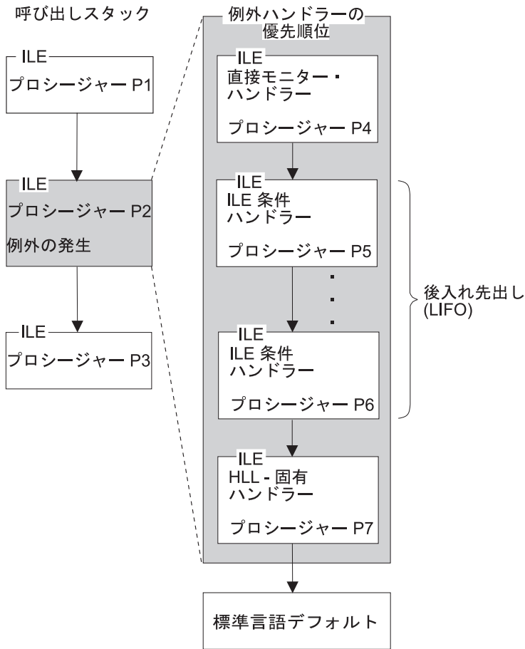
図 26. 例外ハンドラーの優先順位
