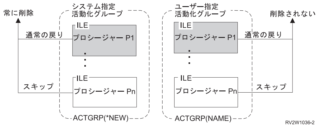
図 19. ユーザー指定活動化グループとシステム指定活動化グループの存続
