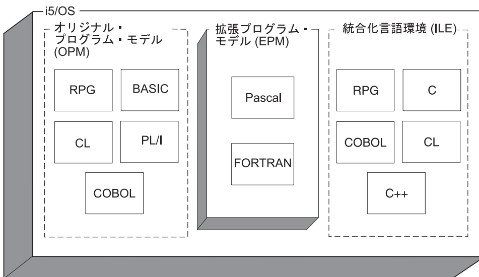
図 5. OPM、EPM、および ILE と i5/OS の関係
