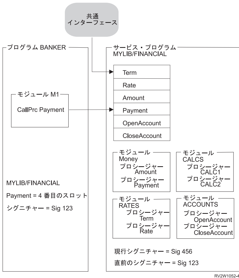
図 36. バインド・プログラム言語の使用によるサービス・プログラムの更新
