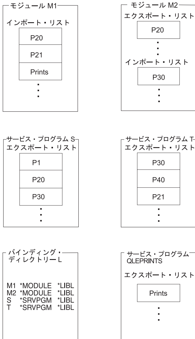
図 30. モジュール、サービス・プログラム、およびバインディング・ディレクトリー
