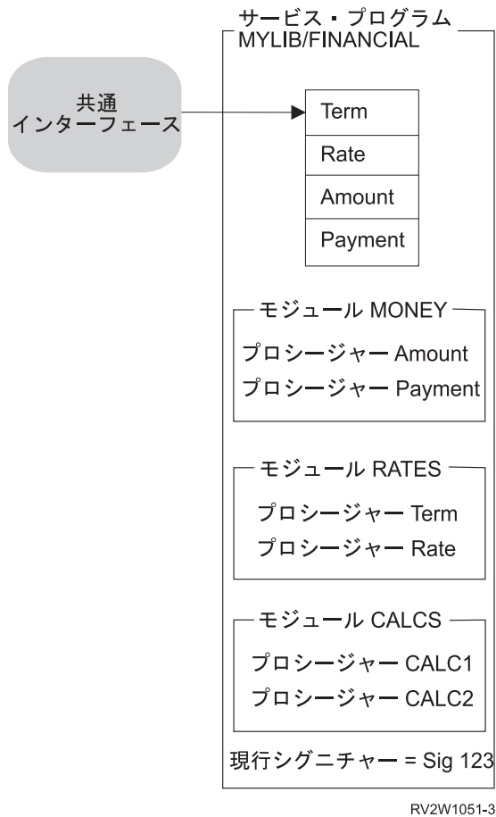
図 34. バインド・プログラム言語の使用によるサービス・プログラムの作成
