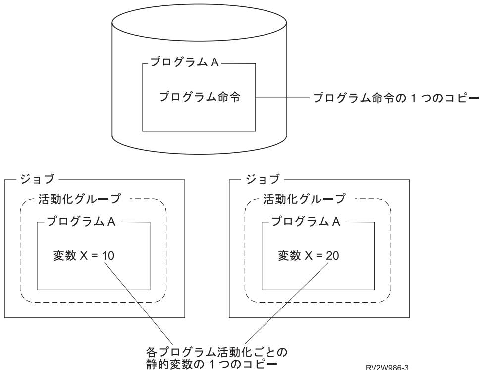
図 15. 各プログラム活動化ごとの静的変数の 1 つのコピー
