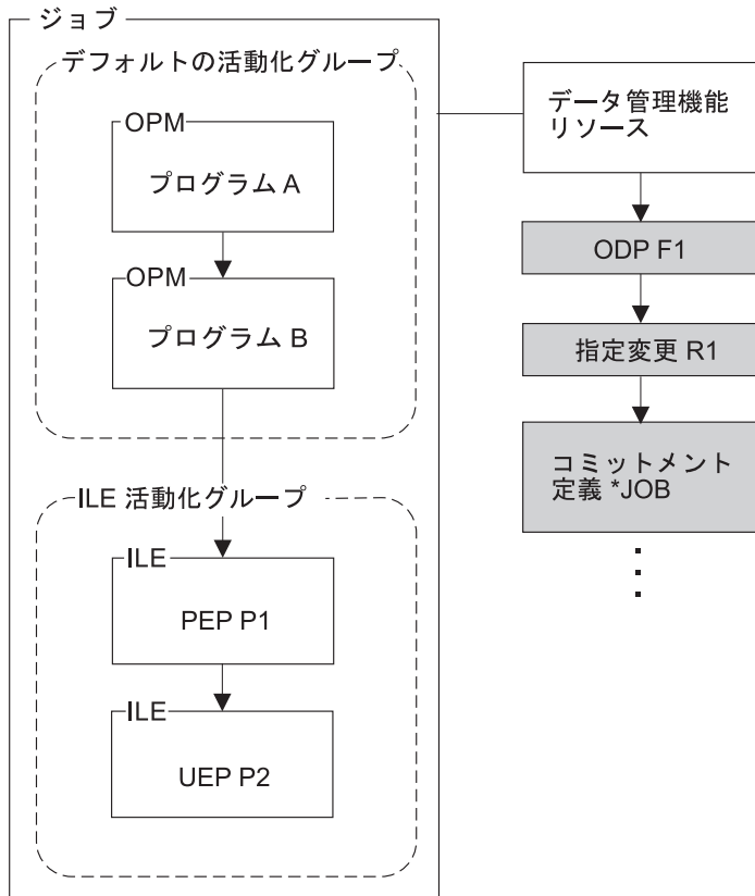
図 29. ジョブ・レベルの有効範囲指定：(ODP、指定変更、およびコミットメント定義の有効範囲はジョブ・レベルにすることができます。)
