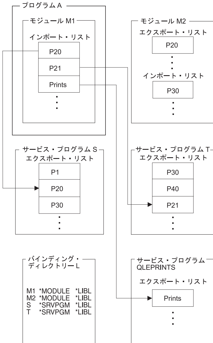
図 31. 記号の解決とプログラムの作成: 例 1
