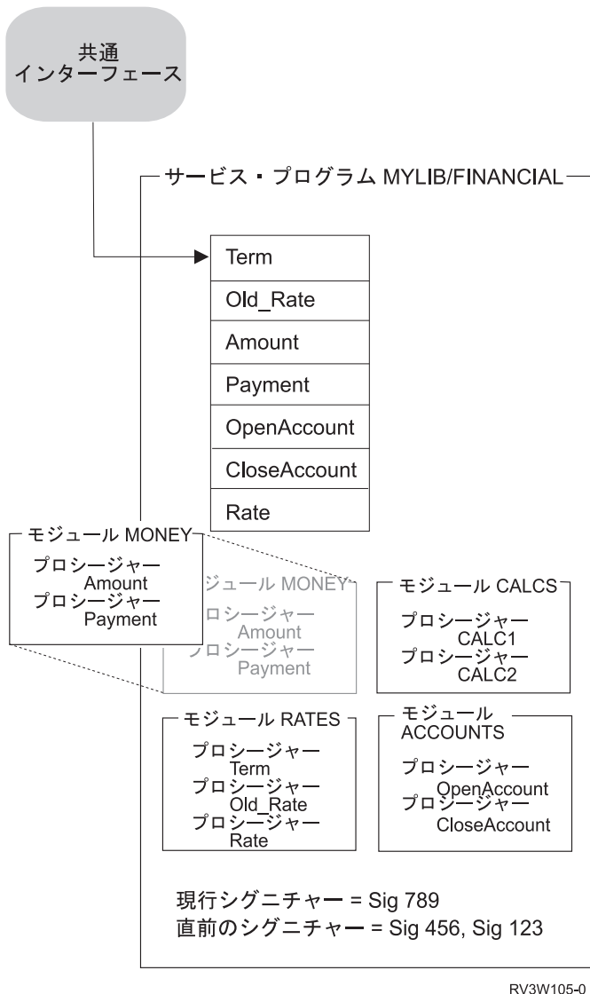
図 38. サービス・プログラムでのモジュールの置き換え
