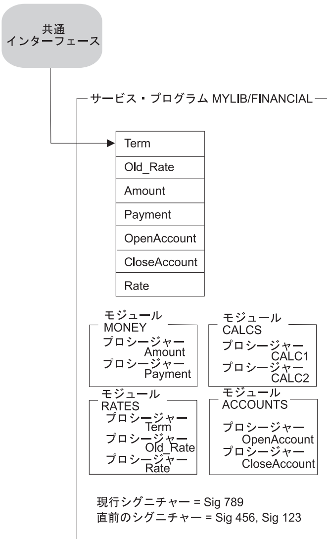
図 37. バインド・プログラム言語の使用によるサービス・プログラムの更新
