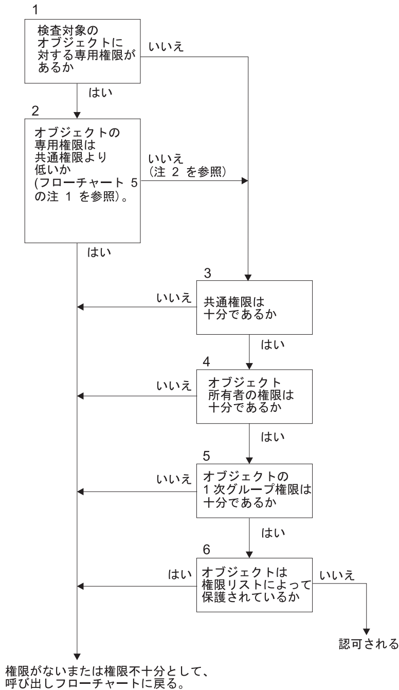
図 15. フローチャート 5: ユーザー権限の高速パス
