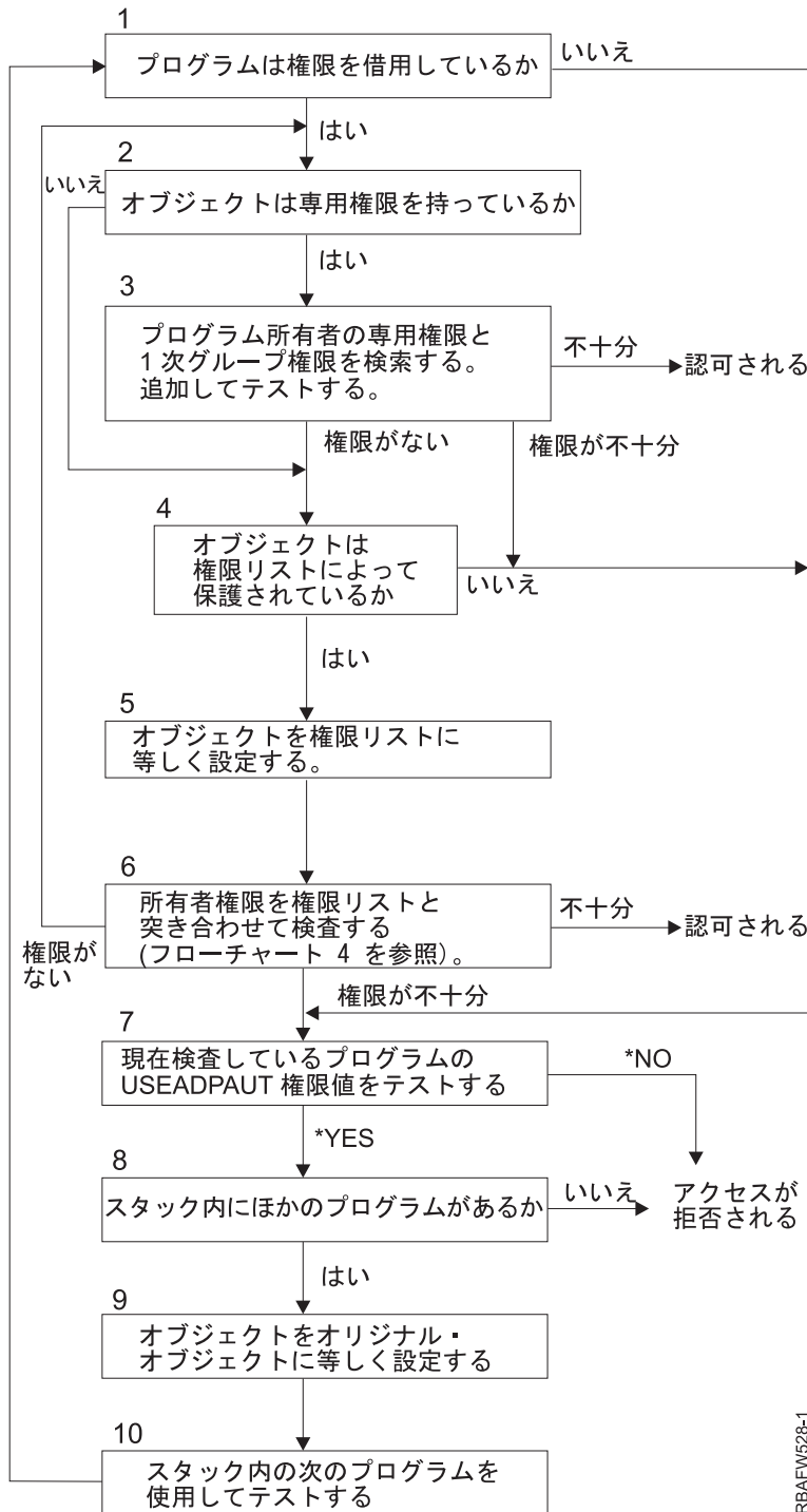
図 19. フローチャート 8B: 専用権限を使用する借用権限の検査
