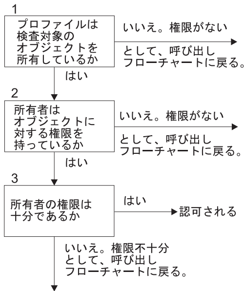
図 14. フローチャート 6: 所有者権限の検査
