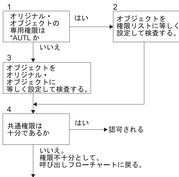
図 17. フローチャート 7: 共通権限の検査
