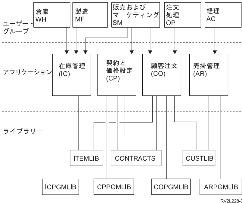
図 31. アプリケーション例
