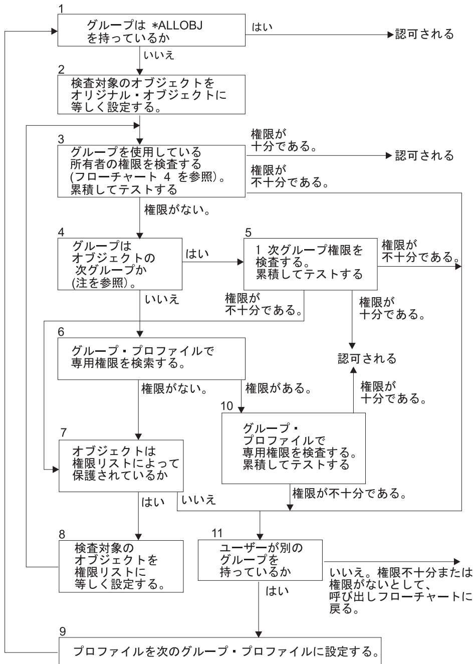
図 16. フローチャート 6: グループ権限検査
