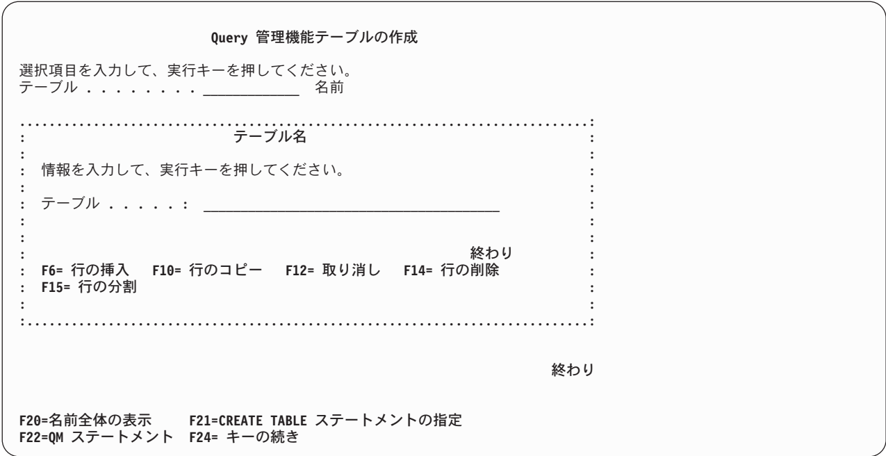
図 113. チュートリアル: テーブルの名前全体を表示するための画面
