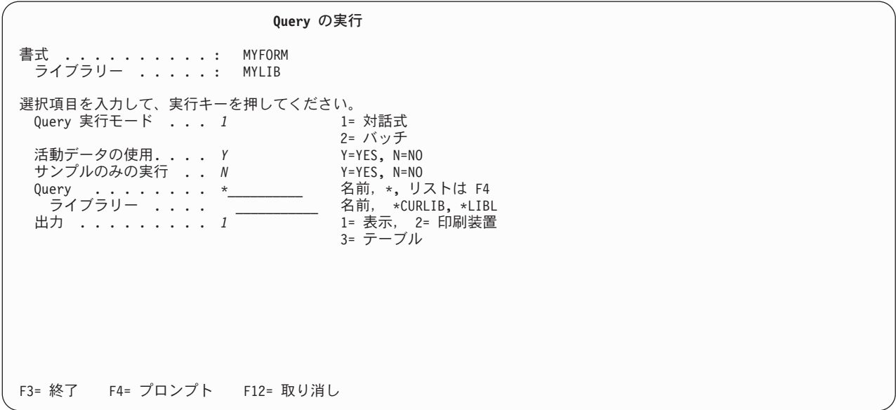
図 79. 報告書のための「Query の実行」画面
