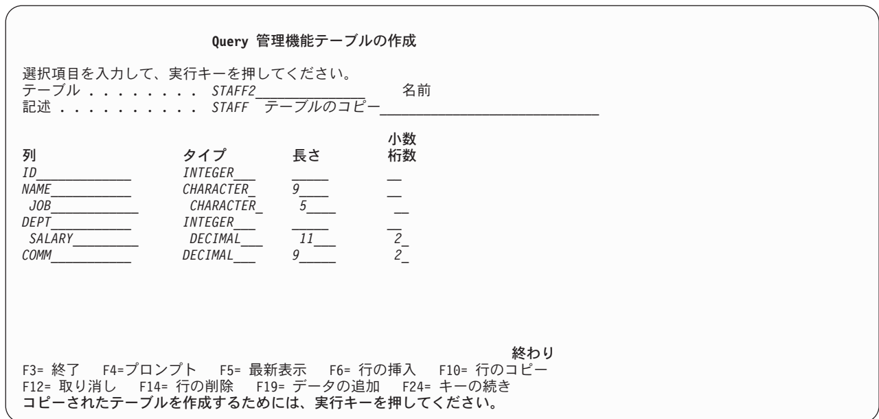
図 122. チュートリアル: テーブルをコピーするための画面
