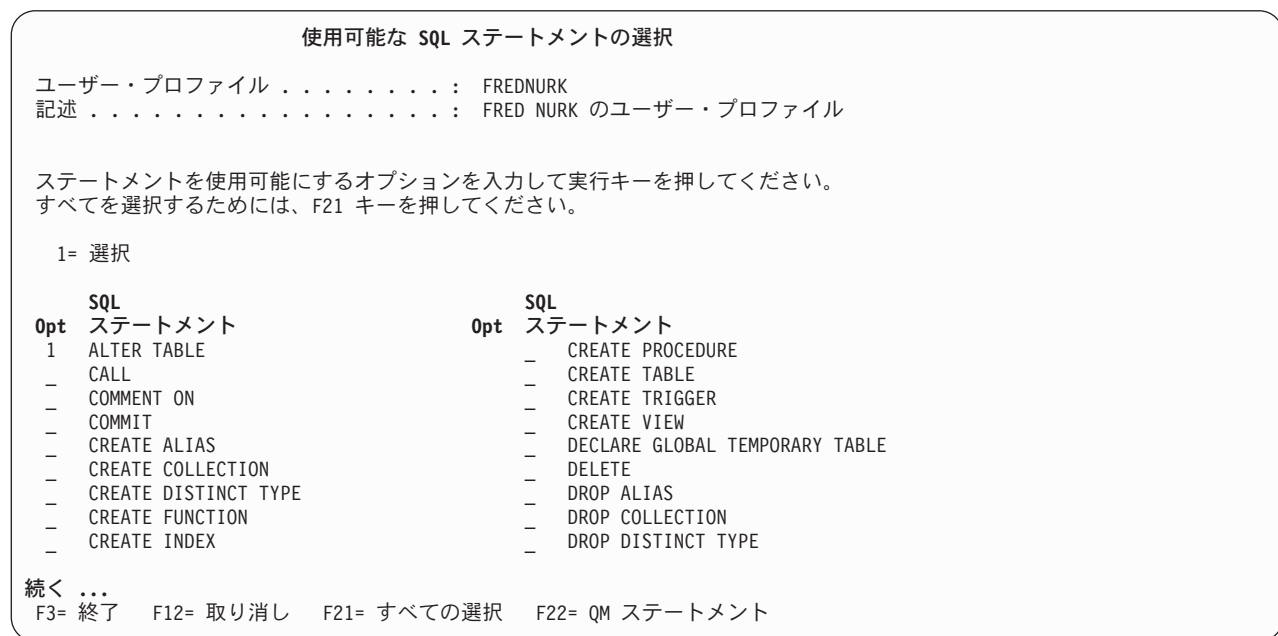
図 20. 「使用可能な SQL ステートメントの選択」画面
