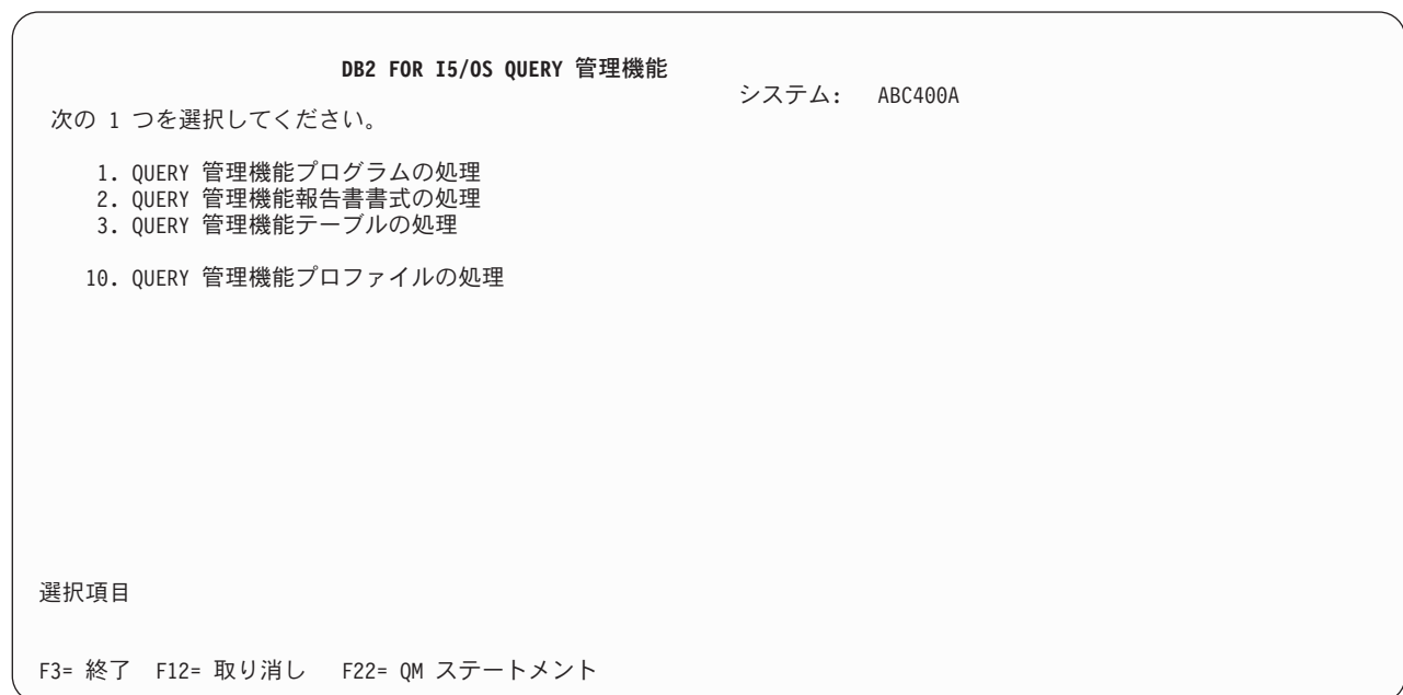
図 4. メイン・メニュー画面
