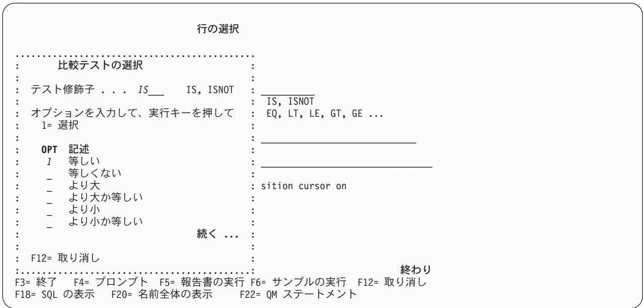
図 138. チュートリアル: プロンプト Query を作成するための画面
