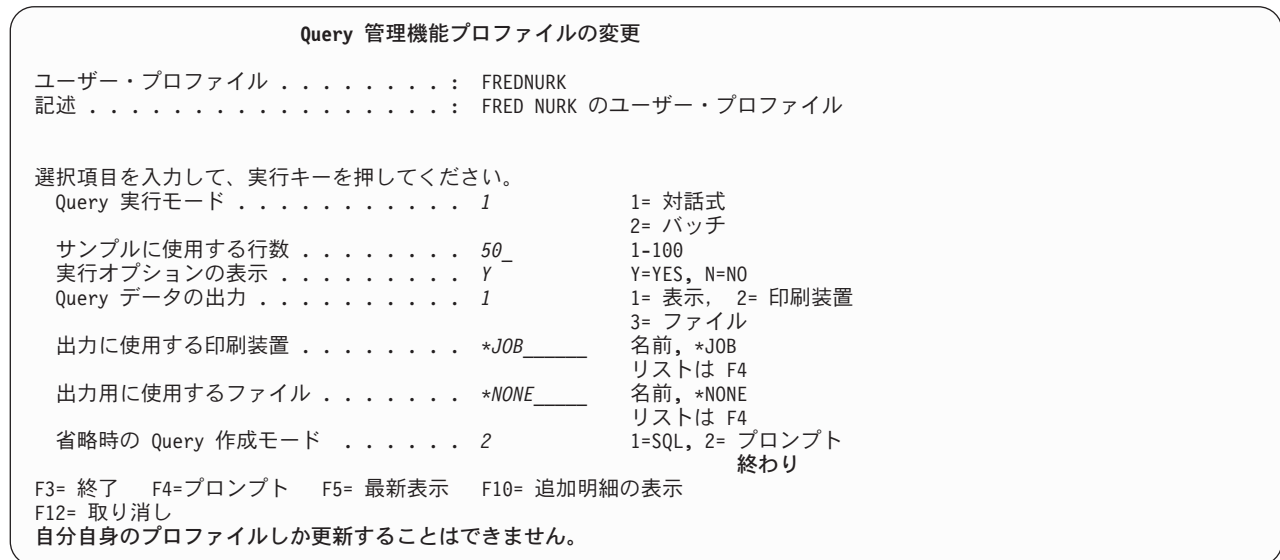
図 14. アクセス・レベル基本のユーザー用の「Query 管理機能プロファイルの変更」画面
