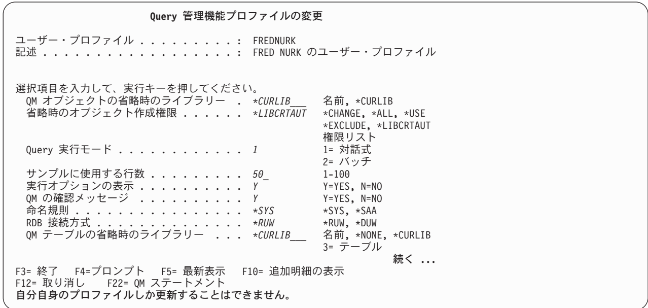
図 15. アクセス・レベル "すべて" のユーザー用の「Query 管理機能プロファイルの変更」画面
