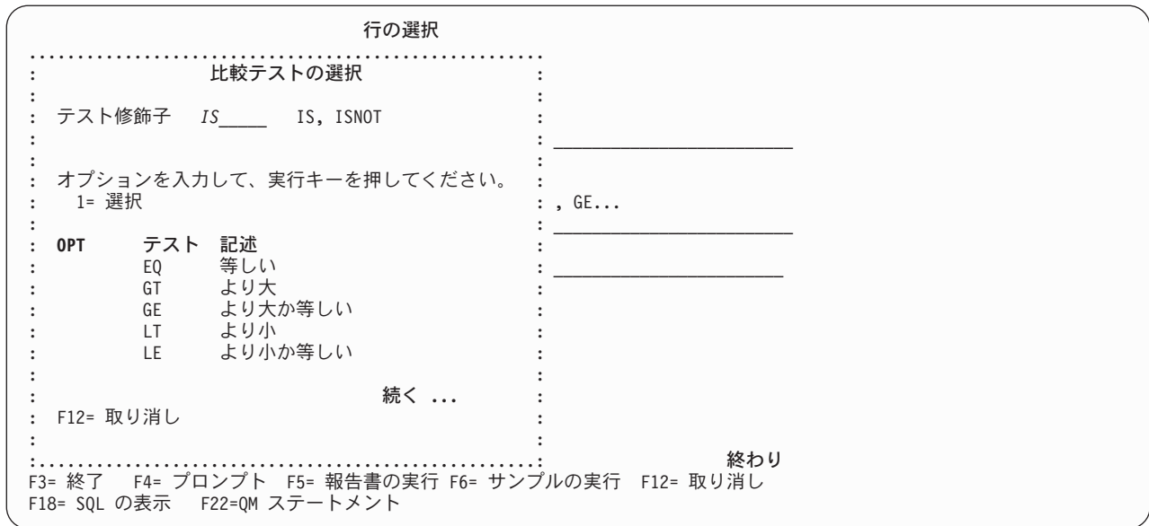
図 49. 「比較テストの選択」ウィンドウ
