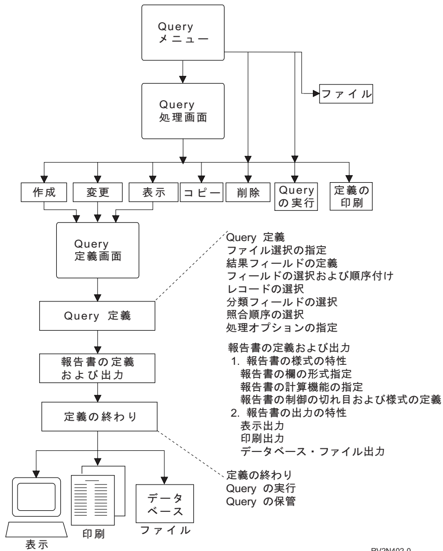
図3. Query メニューと「Query 処理」画面における主要な作業
