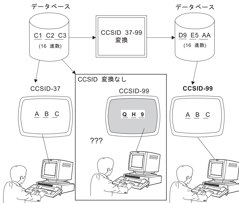
図 7. CCSID 変換を行う場合と行わない場合の処理：変換が必要で、しかも可能な場合には、システムにより自動的に行われます。
