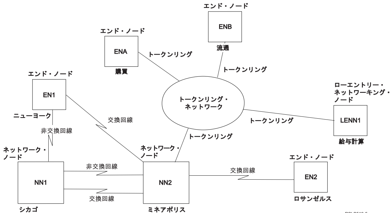
図 8. APPN を使用する複数の iSeries システム
