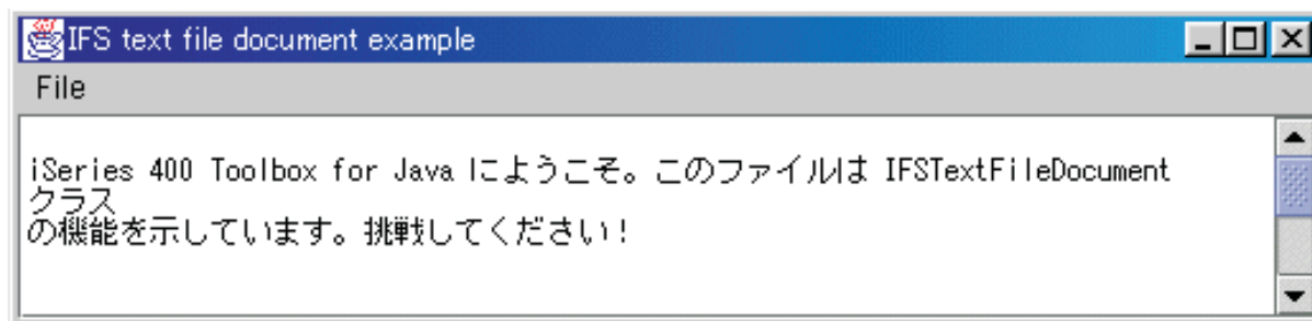
図 1: IFSTextFileDocument の例
