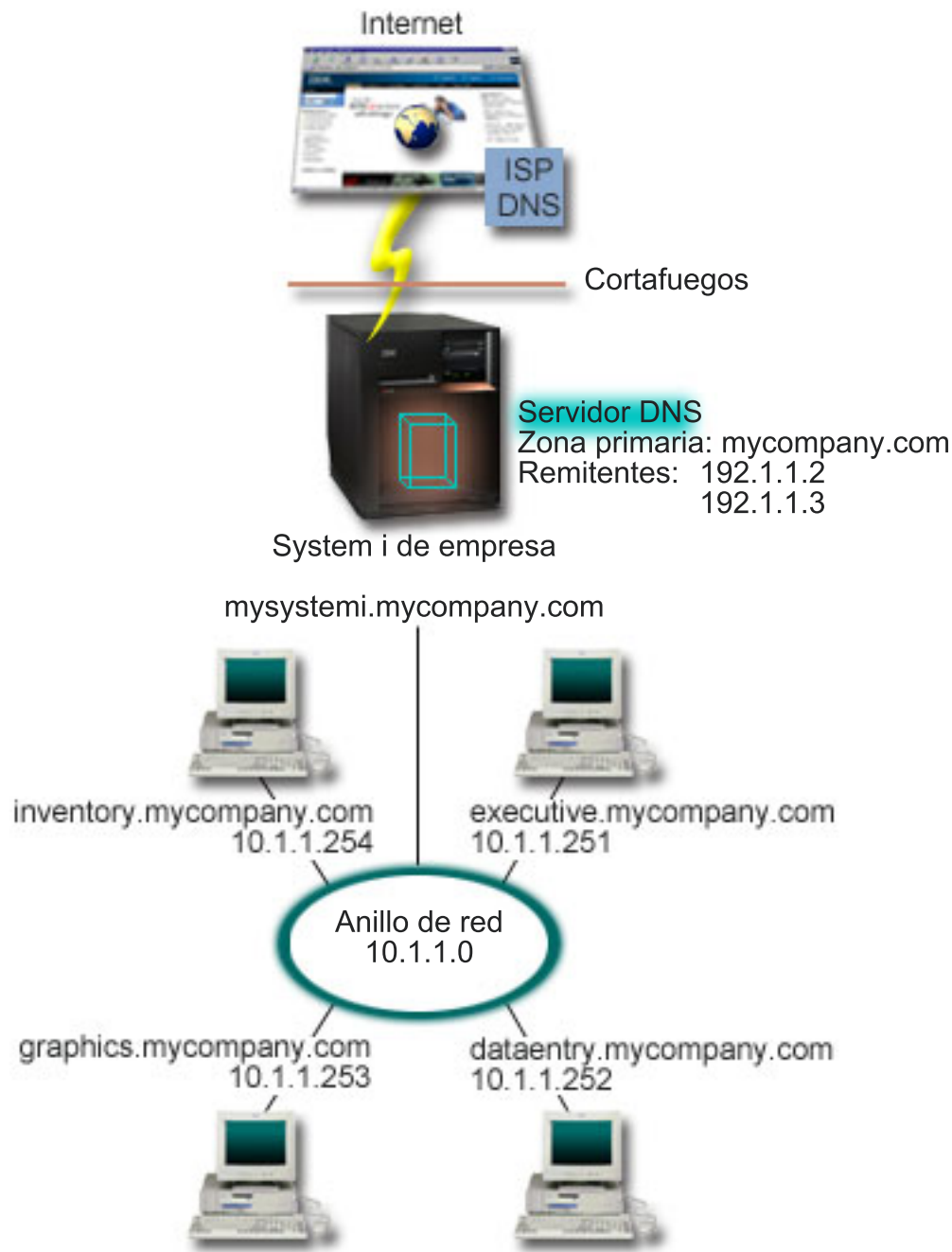
Figura 1. Un único servidor DNS con acceso a Internet
