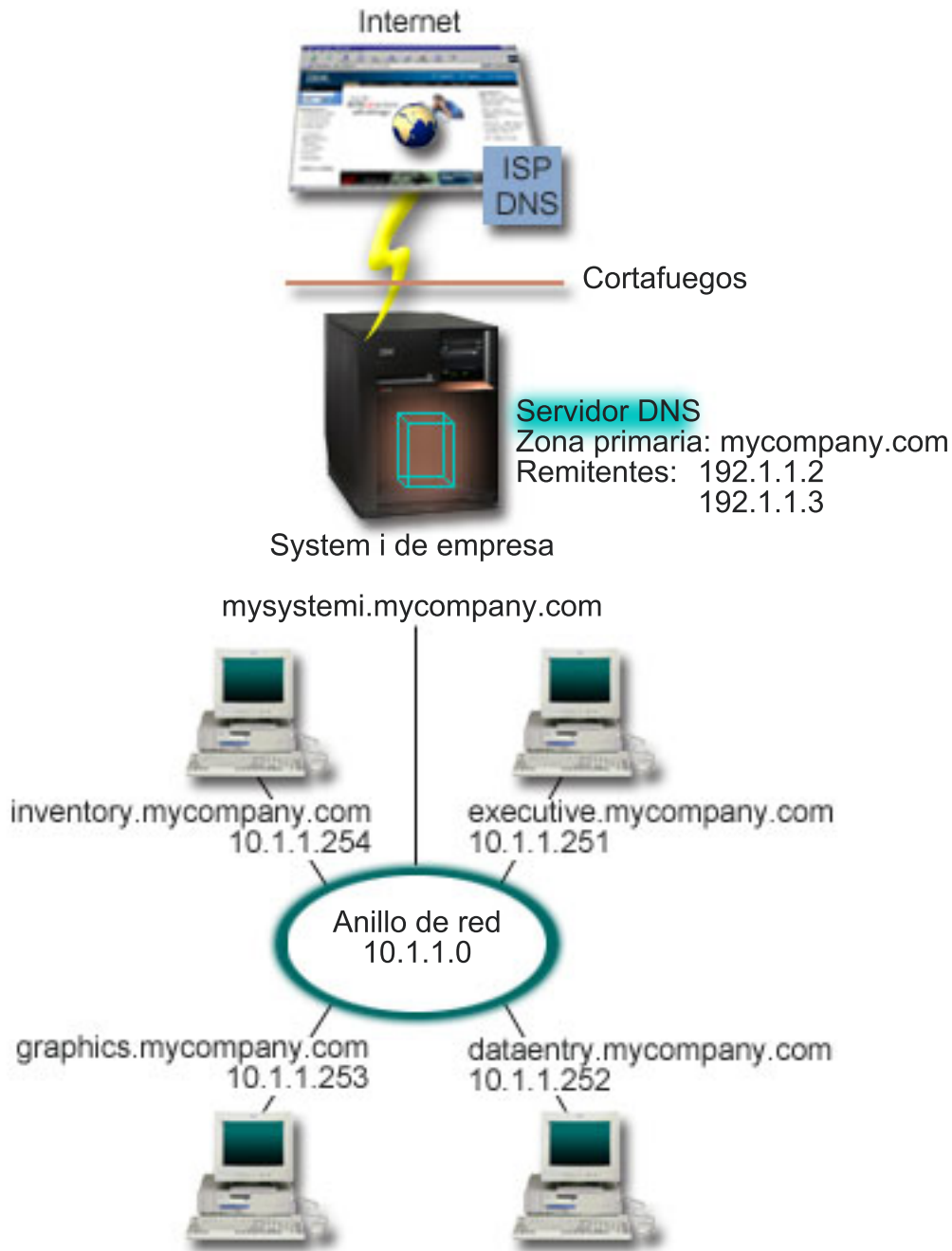
Figura 3. Un único servidor DNS con acceso a Internet
