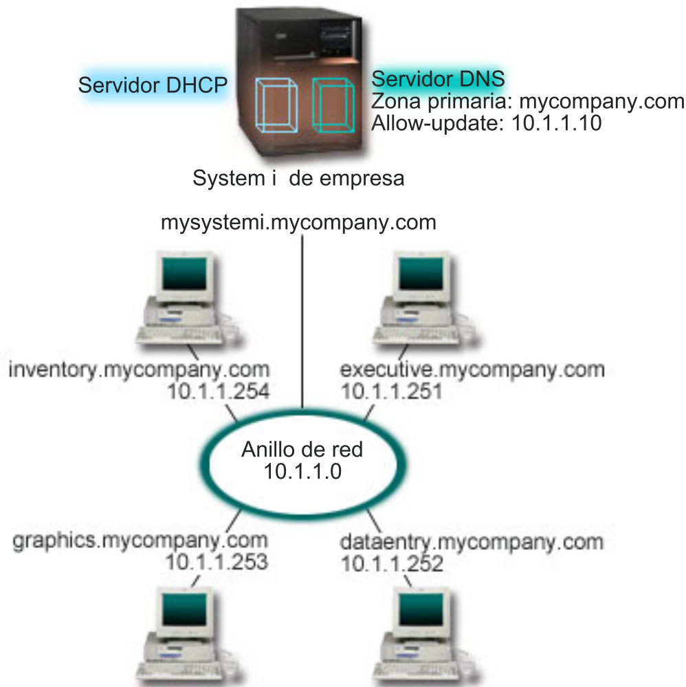
Figura 4. DNS y DHCP en la misma plataforma System i
