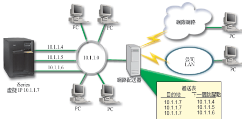
圖 2. 具有本端用戶端的配接卡錯誤後移轉
