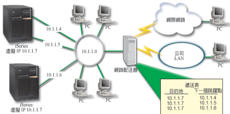
圖 3. 具有多部 iSeries 及本端用戶端的配接卡錯誤後移轉
