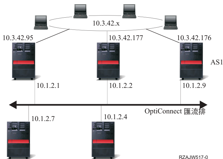
模擬 OptiConnect 的 LAN 配置
