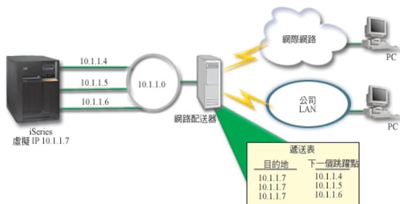
圖 1. 沒有本端用戶端的配接卡錯誤後移轉
