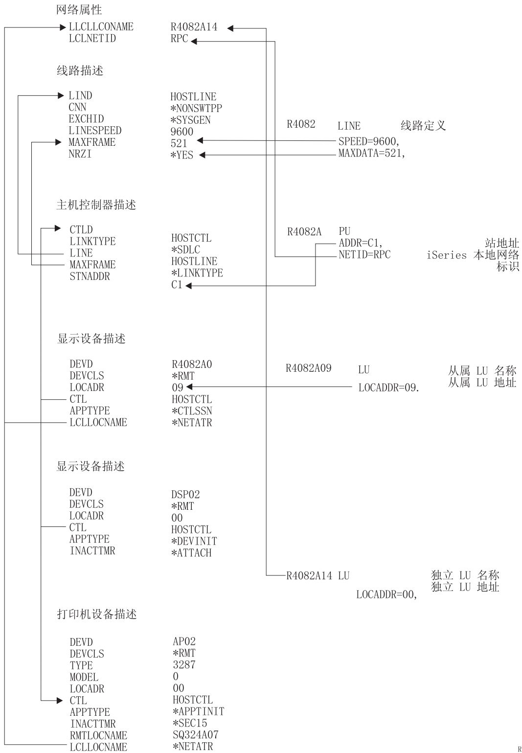
图 1. 显示配置参数如何相关和配置的图。有关更多信息，请访问以上链接以获得详细描述。
