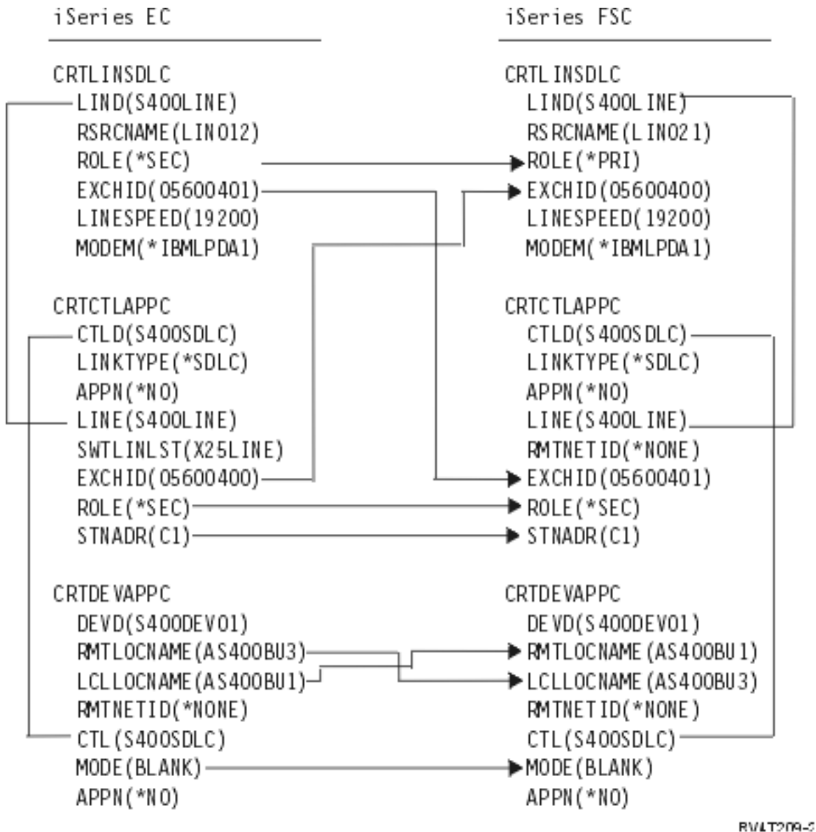
图 6. 显示配置参数如何相关和配置的图。有关更多信息，请访问以上链接以获得详细描述。
