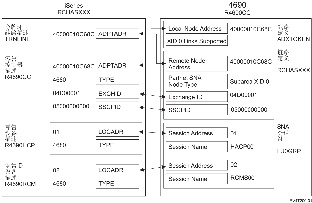
图 11. 显示配置参数如何相关和配置的图。有关更多信息，请访问以上链接以获得详细描述。
