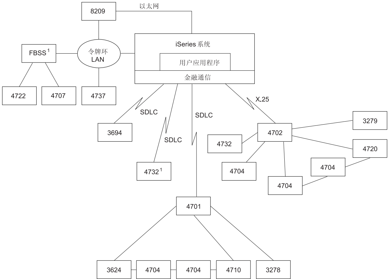
图 10. 显示 iSeries 服务器和金融控制器之间通信结构的图
