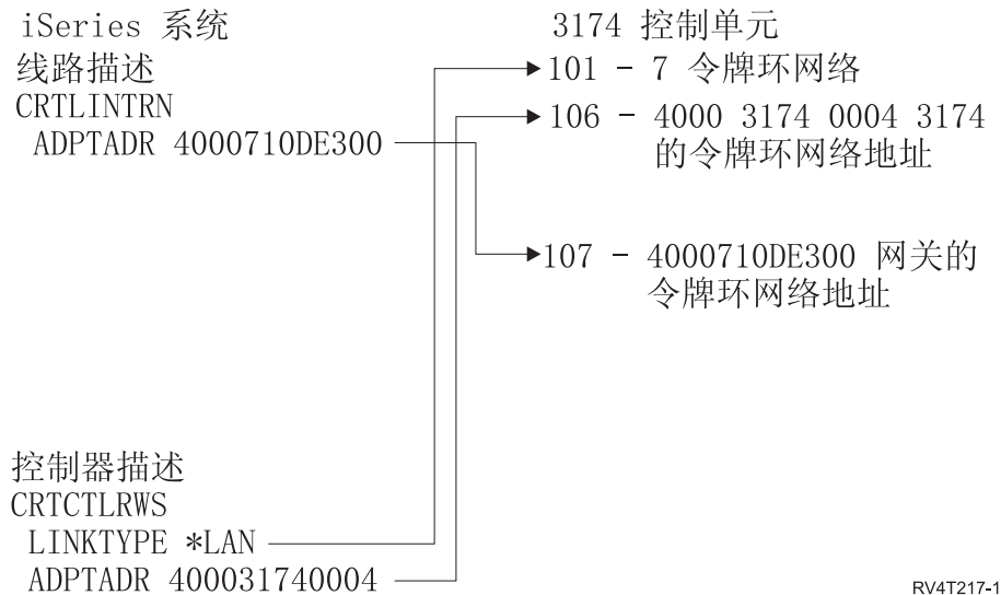
图 9. 显示在使用令牌环时，需要相互匹配的 iSeries 系统参数和 3174 参数的图
