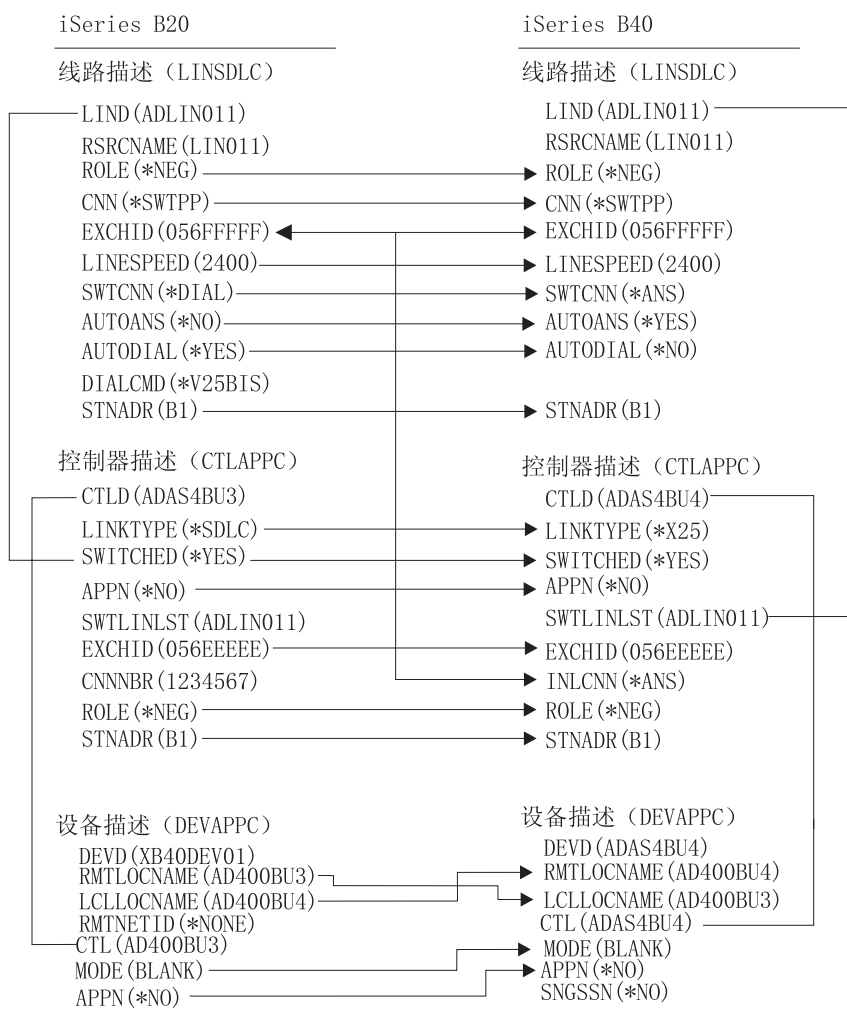
图 7. 显示配置参数如何相关和配置的图。有关更多信息，请访问以上链接以获得详细描述。
