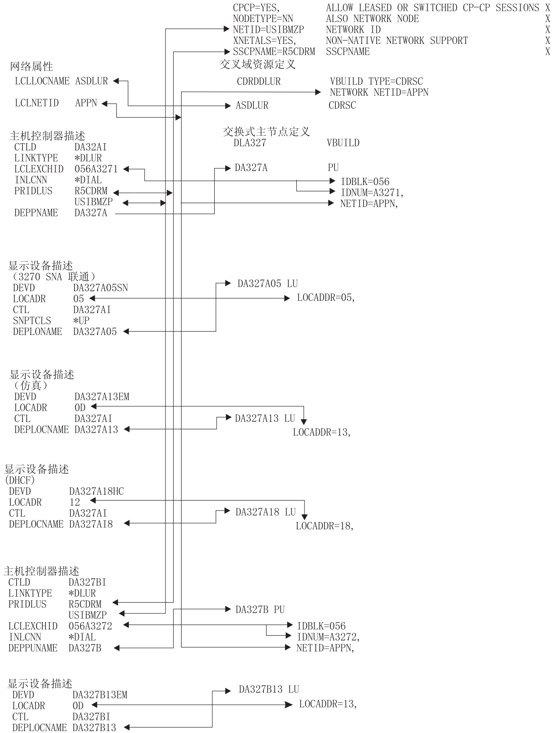
图 4. 显示配置参数如何相关和配置的图。有关更多信息，请访问以上链接以获得详细描述。
