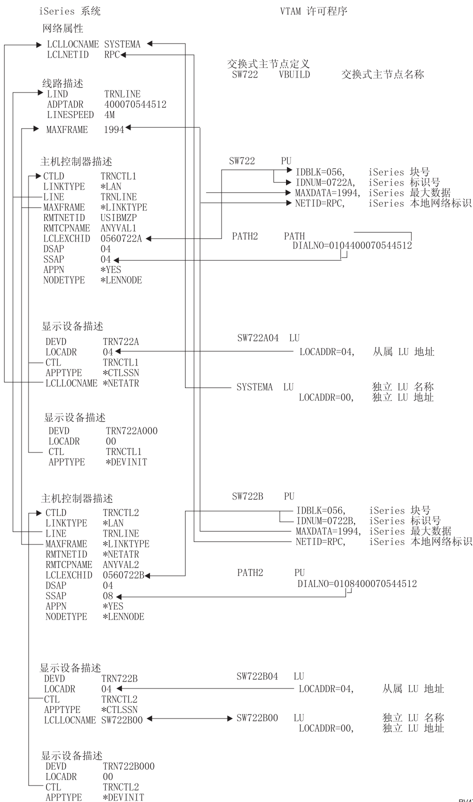
图 2. 显示配置参数如何相关和配置的图。有关更多信息，请访问以上链接以获得详细描述。
