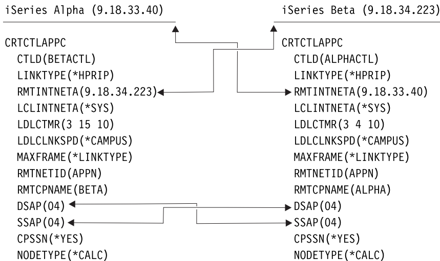
图 8. 显示配置参数如何相关和配置的图。有关更多信息，请访问以上链接以获得详细描述。
