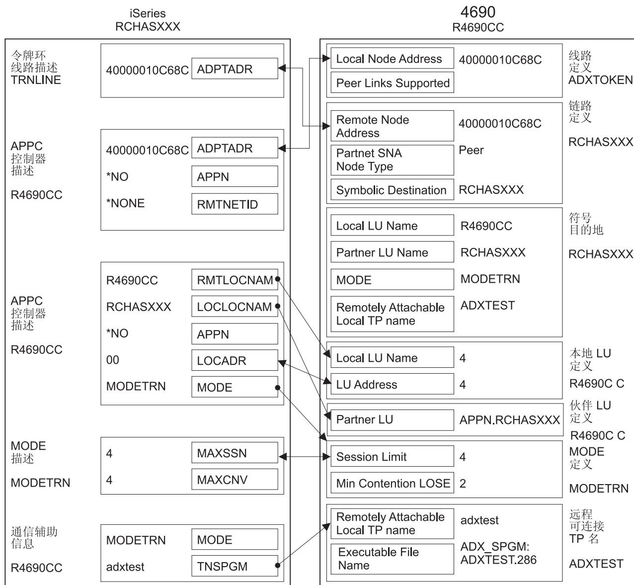
图 12. 显示配置参数如何相关和配置的图。有关更多信息，请访问以上链接以获得详细描述。
