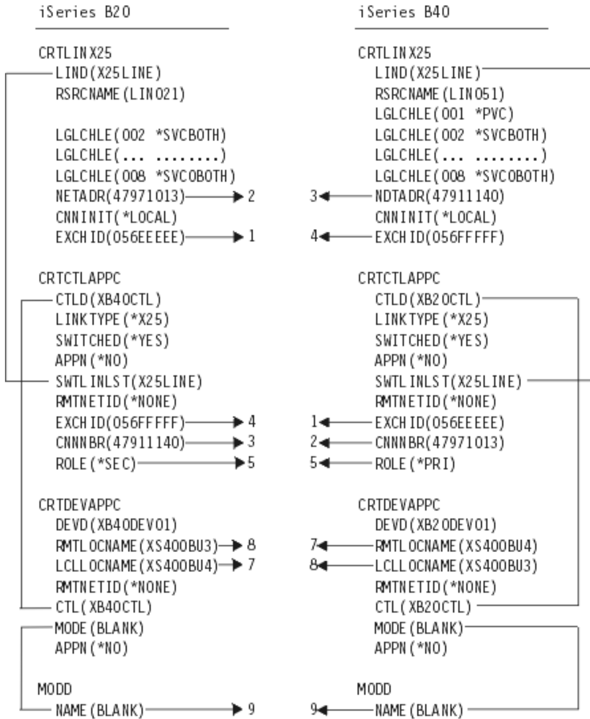
图 5. 显示配置参数如何相关和配置的图。有关更多信息，请访问以上链接以获得详细描述。
