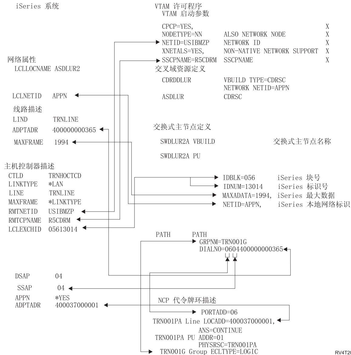
图 3. 显示配置参数如何相关和配置的图。有关更多信息, 请访问以上链接以获得详细描述。
