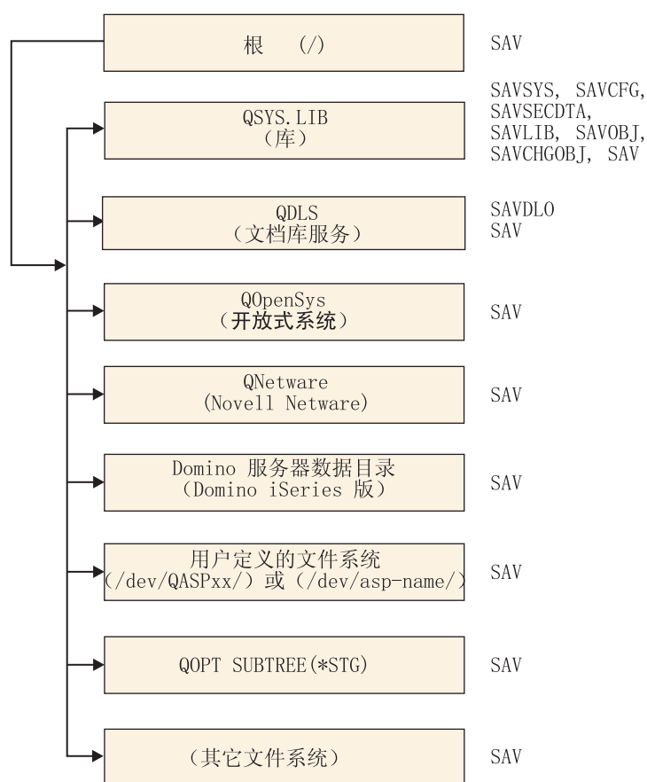
图 5. 文件系统 - 保存命令
