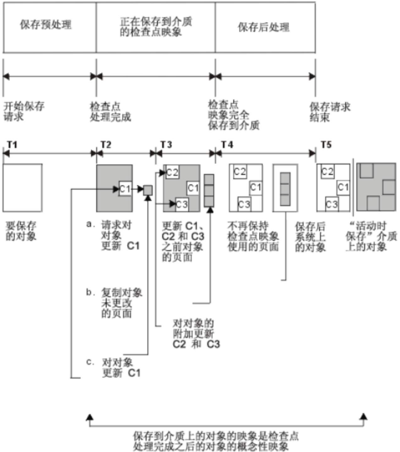
图 6. 检查点处理完成之后对象更新的服务器管理
