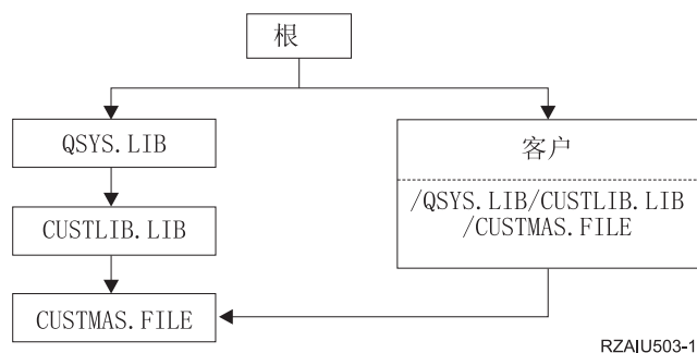
图 4. 具有符号链接的对象 - 示例
