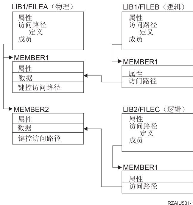
图 2. 保存访问路径
