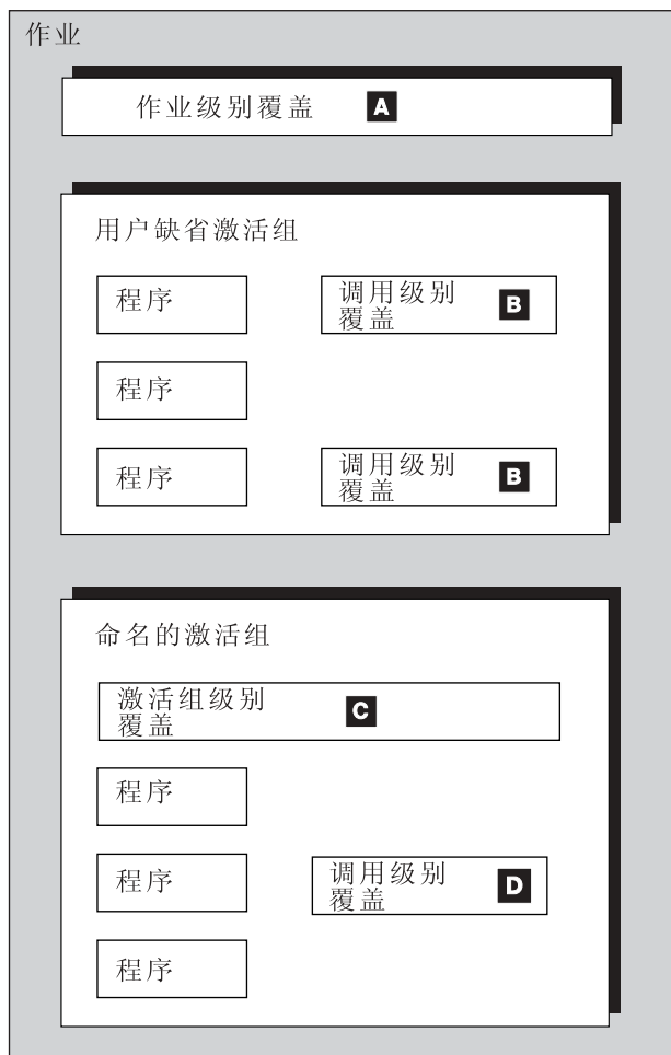
图 4. Integrated Language Environment 中的作业
