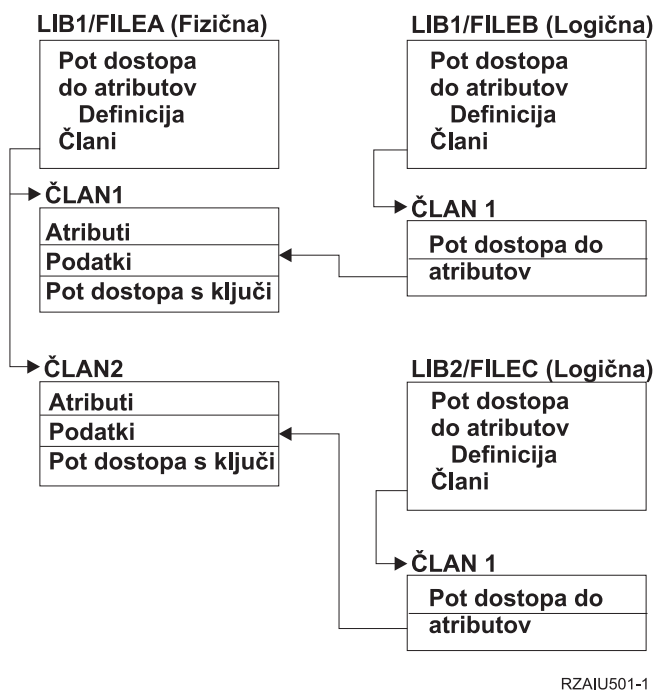
Slika 2. Shranjevanje poti dostopa
