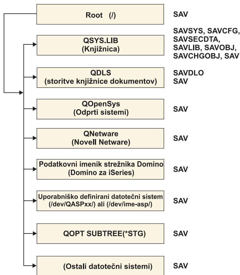
Slika 5. Datotečni sistemi - ukazi za shranjevanje
