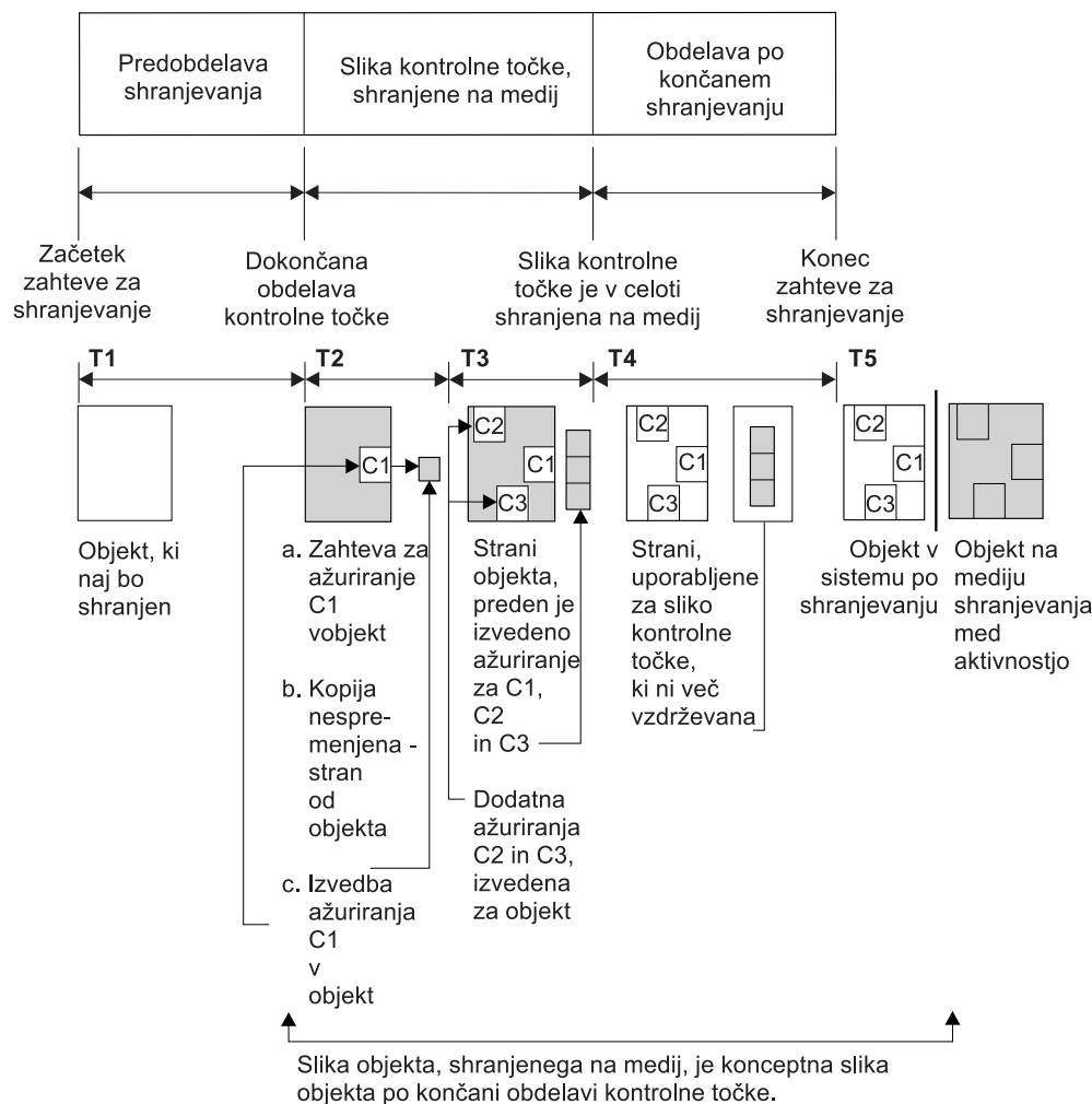
Slika 6. Strežnik je končal z upravljanjem popravkov v objektih po obdelavi kontrolne točke.
