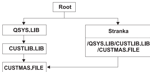
Slika 4. Zgled za objekt s simbolično povezavo
