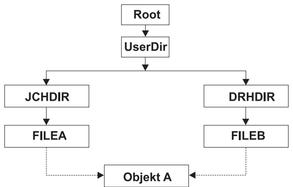
Slika 3. Zgled za objekt s trdimi povezavami
