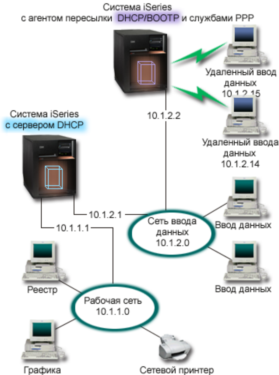
Рисунок 2. Профайлы DHCP и PPP на разных серверах iSeries
