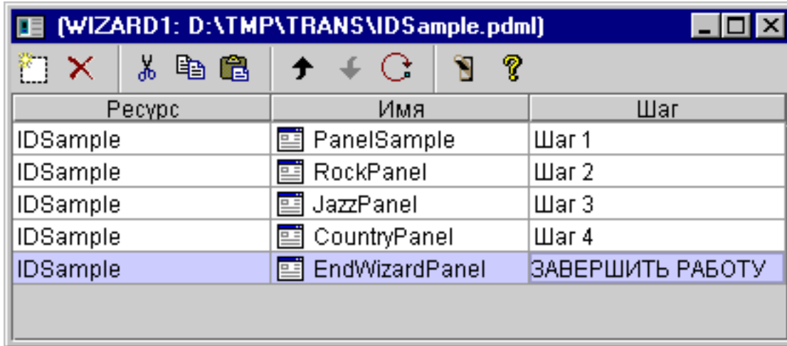
Рисунок 1: Создание мастера с помощью GUI Builder
