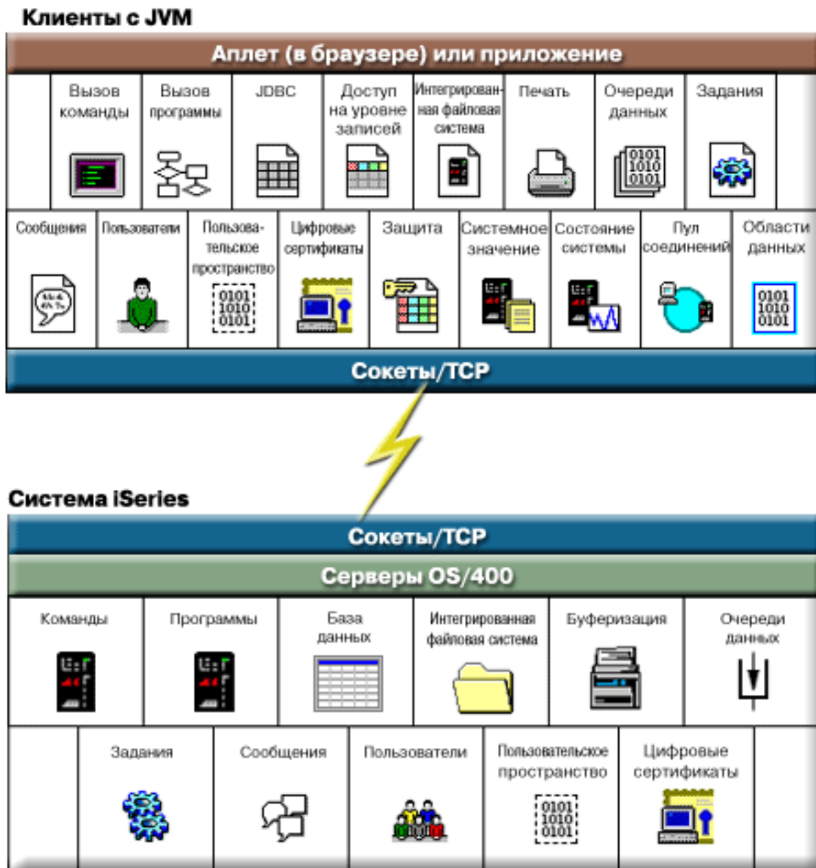
Рис. 1: Точки доступа сервера
