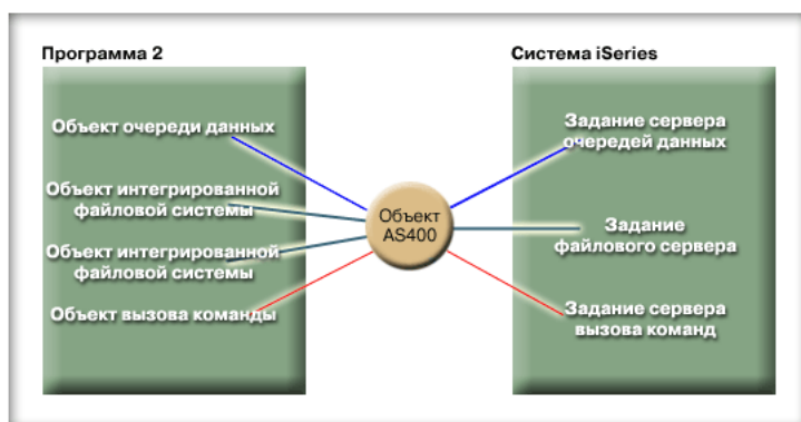
Рисунок 2: Создание одного объекта AS400 и одного соединения с сокетами iSeries в программе на Java
