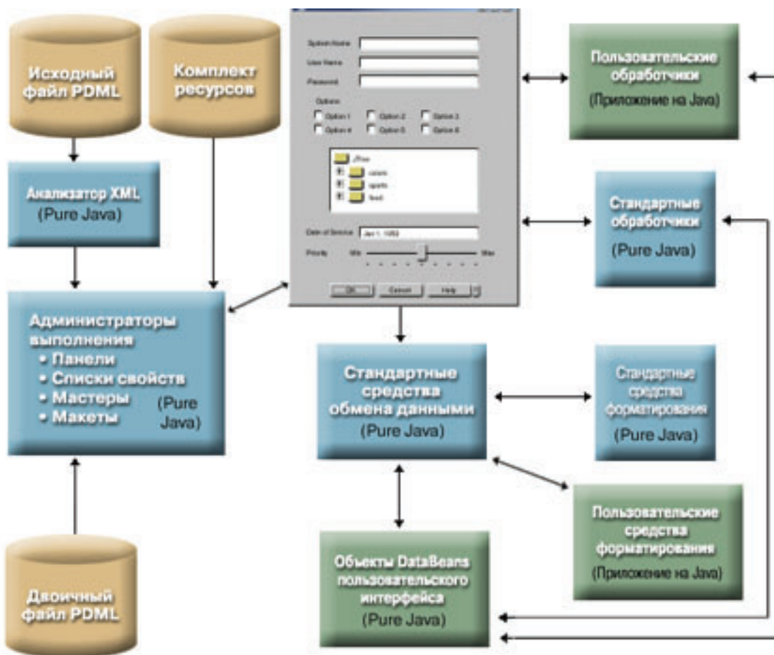
Рис. 1: Среда выполнения Graphical Toolbox
