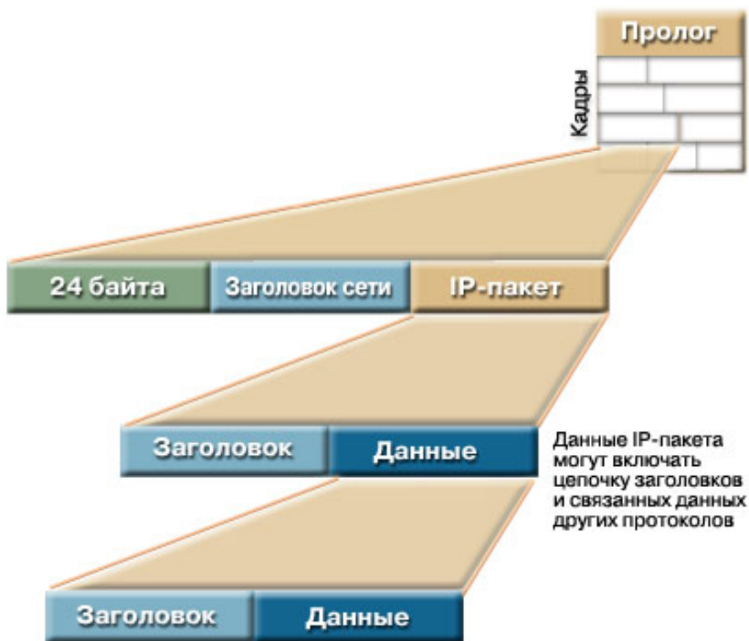
Рисунок 1: Модель Commtrace
