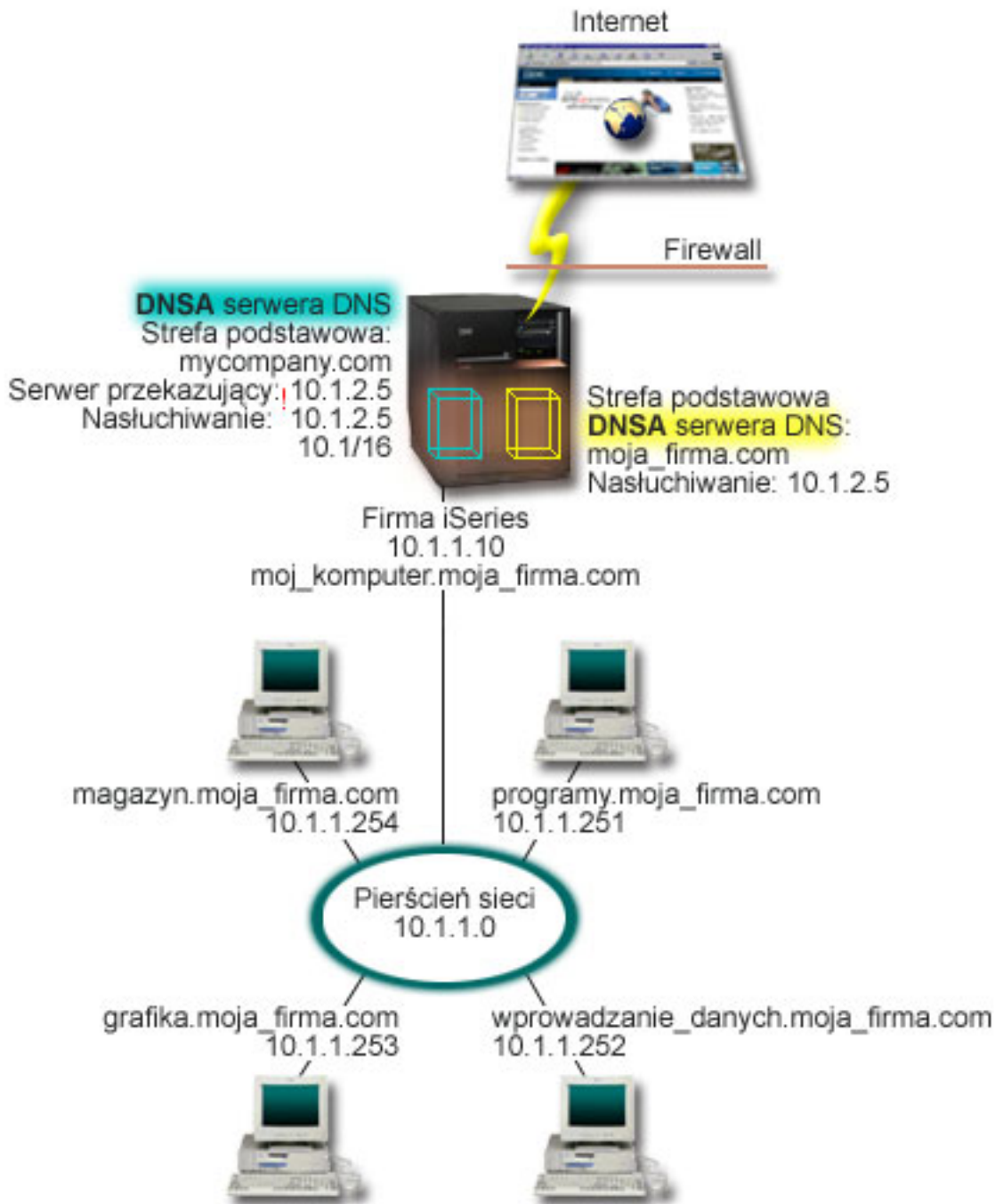
Rysunek 5. Dzielenie usług DNS poprzez firewall.
