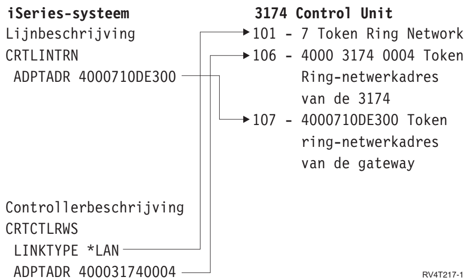
Figuur 9. Afbeelding met de iSeries-systeemparemeters en 3174-parameters die overeen moeten komen als u token-ring gebruikt
