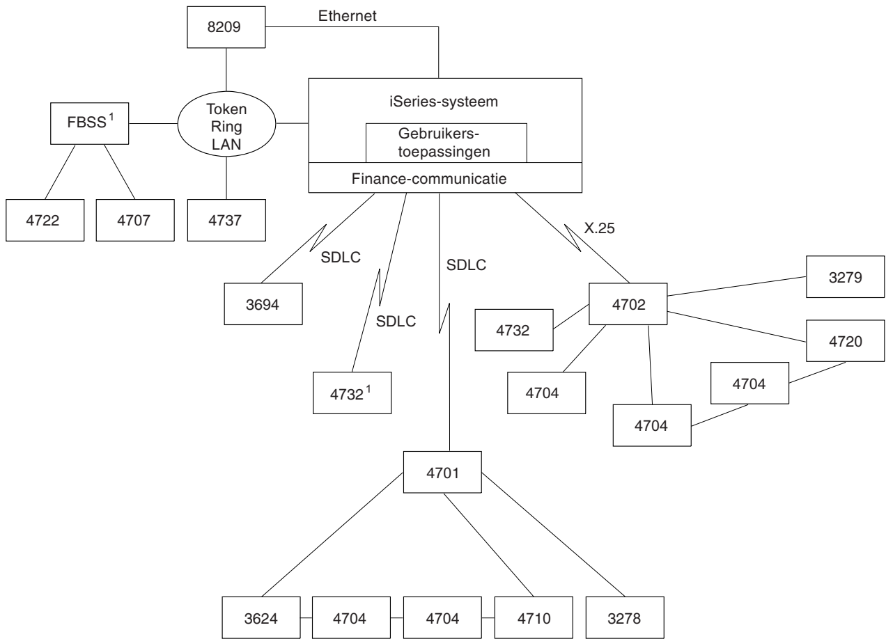
Figuur 10. Afbeelding van de communicatiestructuur tussen een iSeries-server en finance-controllers
