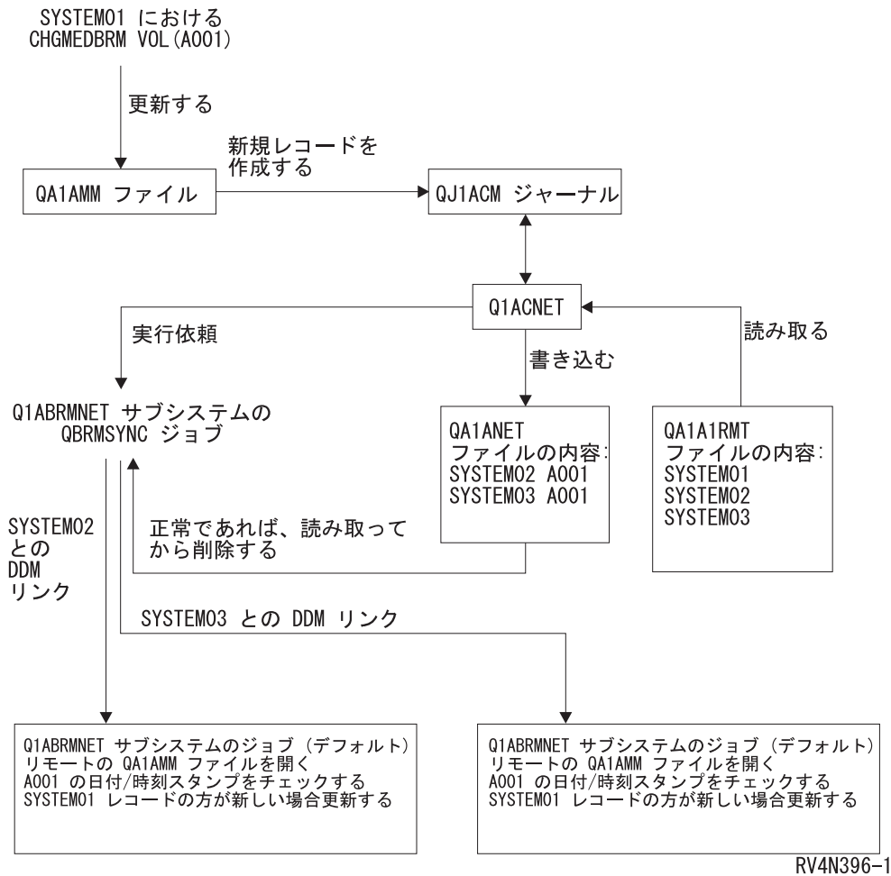
図 12. BRMS のネットワーク同期化処理
