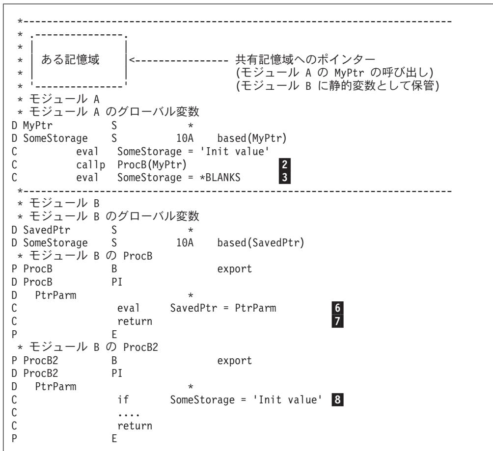
図 74. マルチスレッド環境でのデータの共用例
