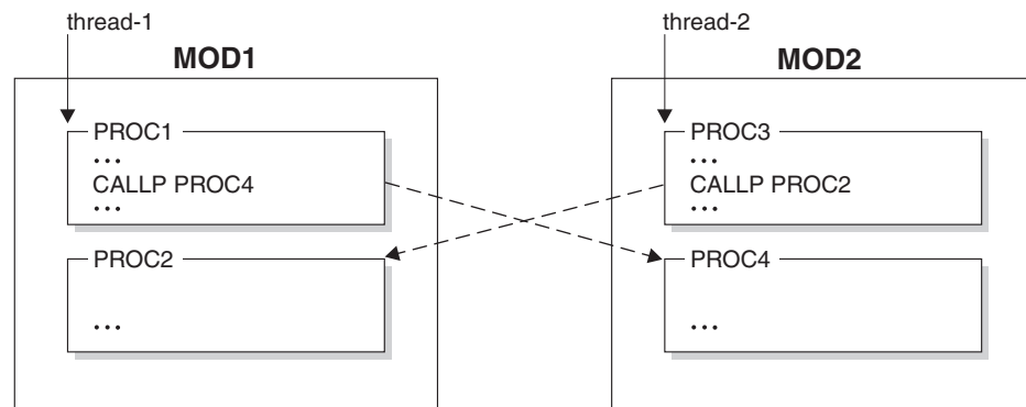
図 75. デッドロックの例
