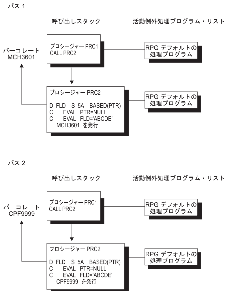
図 130. 処理不能の機能チェックのシナリオ
