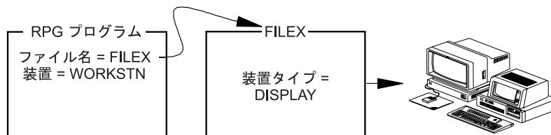
図 148. ファイル名と表示装置ファイル記述との関連付け
