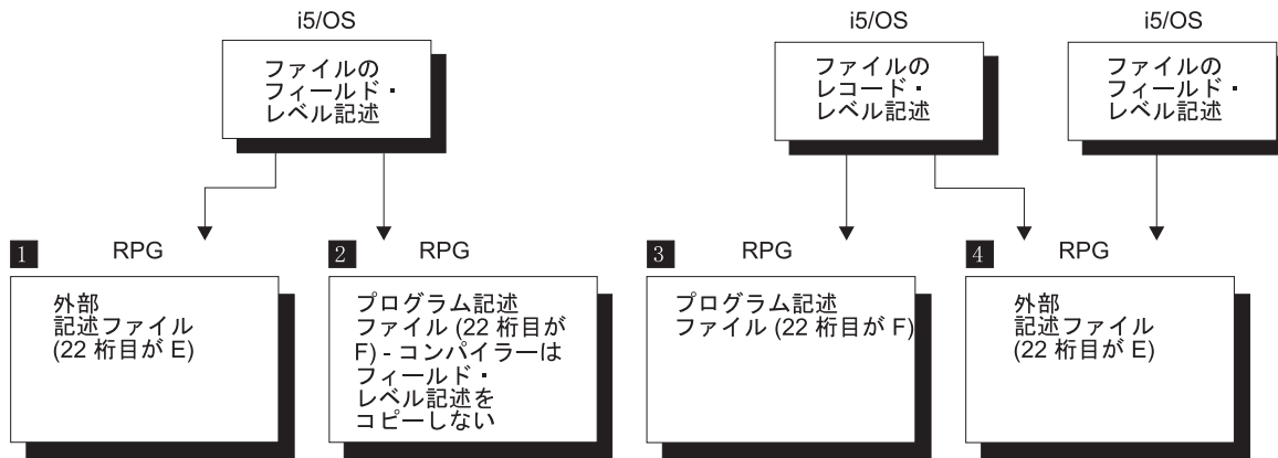
図 150. iSeries システムでの RPG プログラムとファイルの代表的な関係
