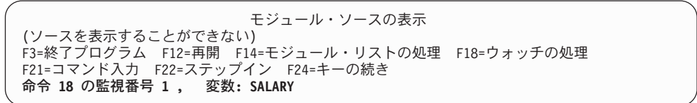
図 112. 「モジュール・ソース表示」パネルの例
