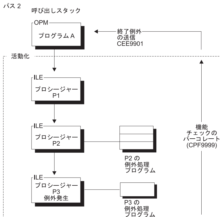
図 128. 呼び出しスタックおよび例外メッセージのパーコレーション
