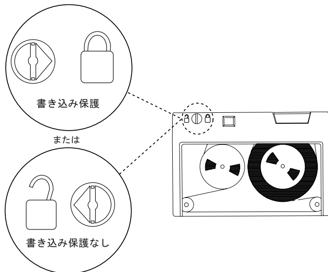
図4. 新しいスタイルの 1/4 インチ・テープ・カートリッジの書き込み保護位置
