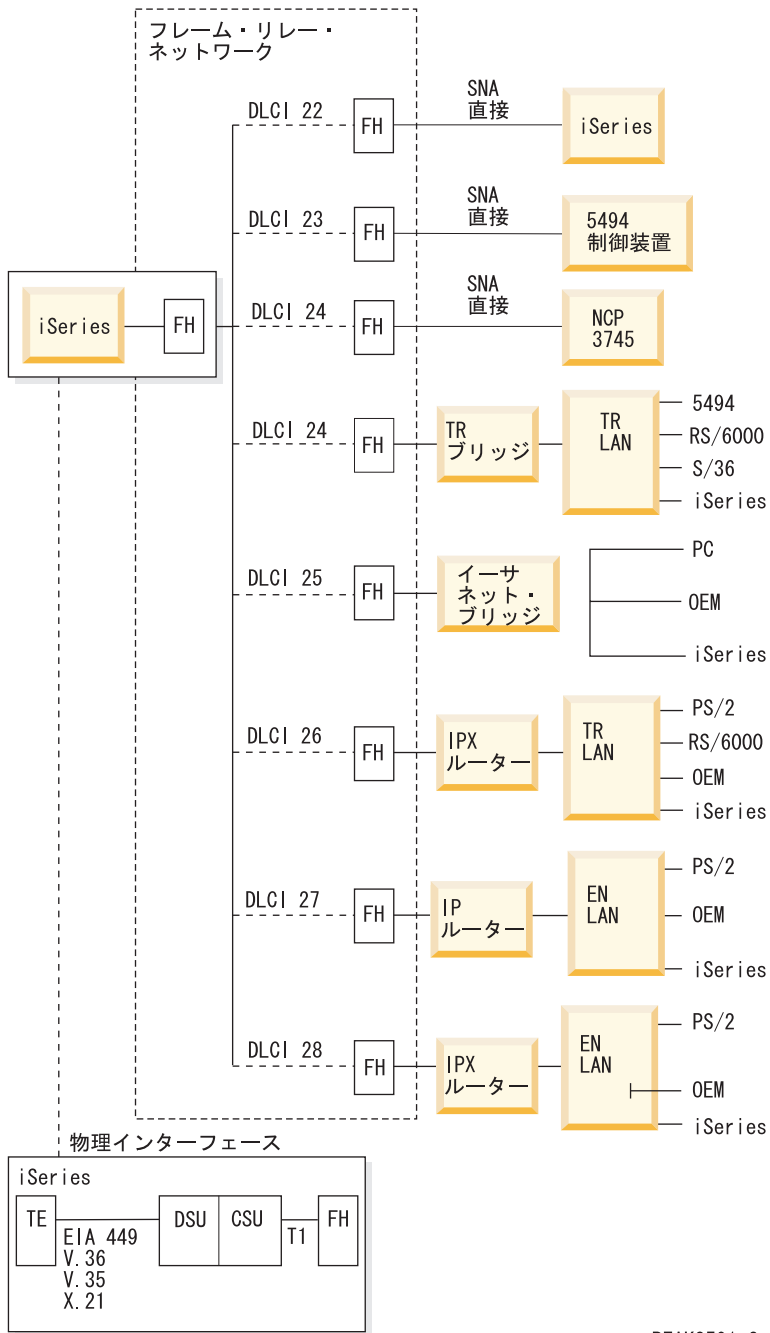
図4. フレーム・リレー・ネットワークの例
