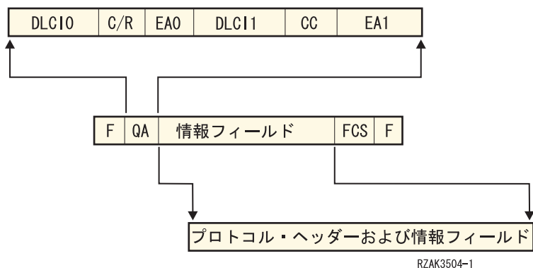
図 8. フレーム・リレー・コア・サービス (FRCS) のフレーム形式
