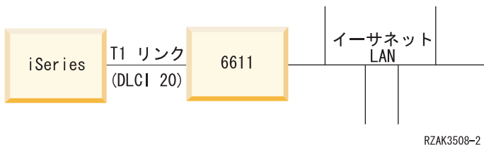
図 21. イーサネット・ネットワークへのブリッジによる構成
