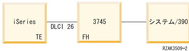
図 19. 3745 ホスト制御装置への SNA 直接接続
