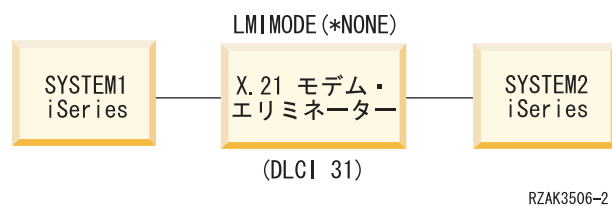
図 18. モデム・エリミネーター使用の SNA 直接接続
