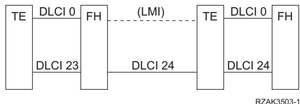
図 6. PVC 接続の DLCI 割り当ての例
