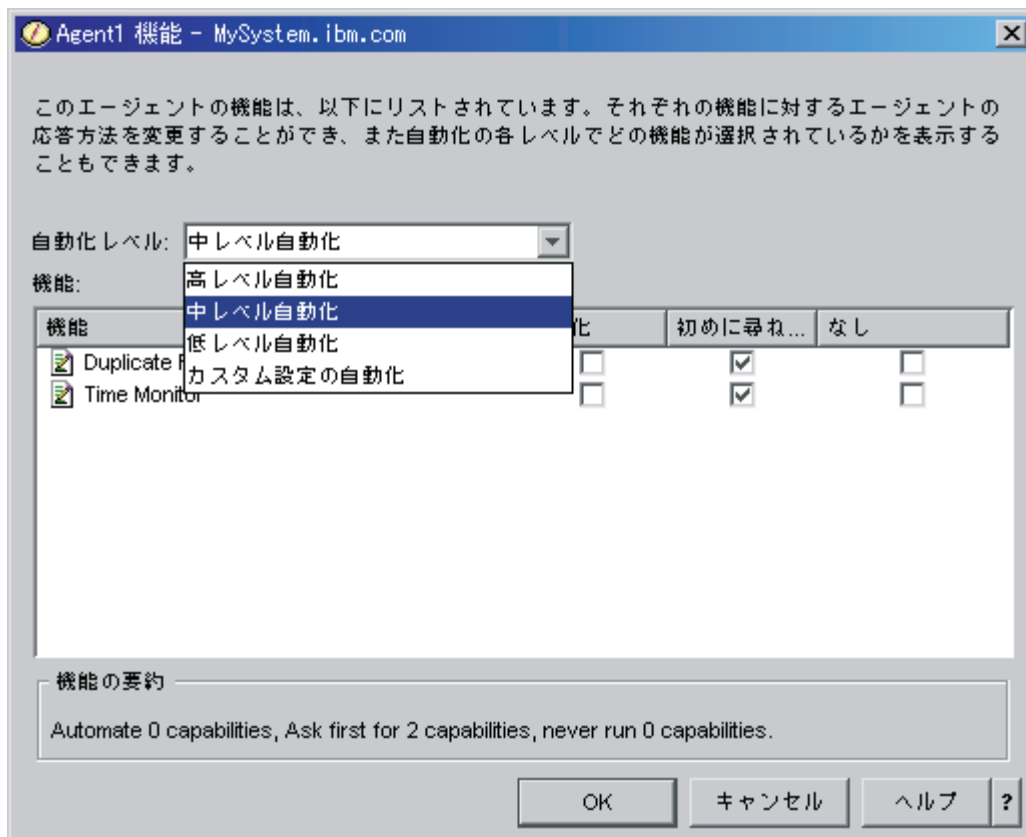
図4. TimeMonitor エージェントの機能に関連付けられた自動化レベルの表示
