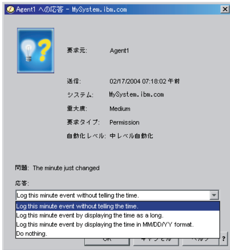
図 5. エージェントの要求に応答する
