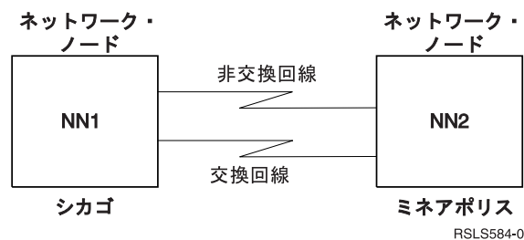
図 5. APPN の 2 つのシステム・ネットワーク
