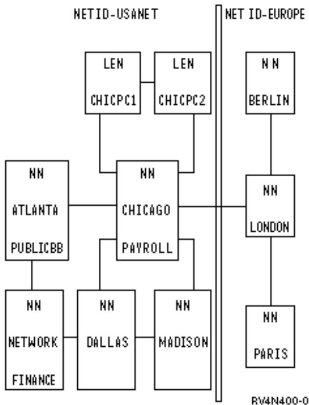
図 12. 2 つの接続された APPN ネットワーク
