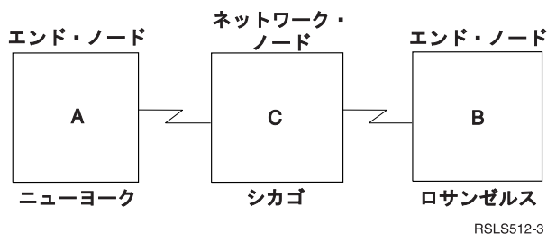
図 10. 3 つのシステムの HPR ネットワーク
