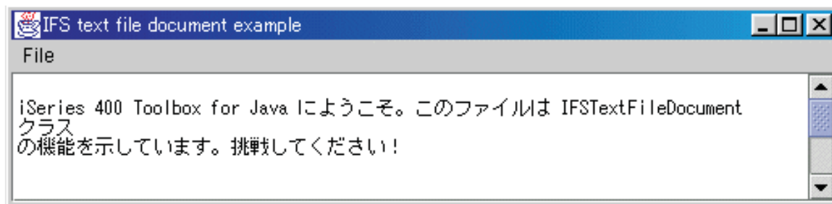
図 1: IFSTextFileDocument の例
