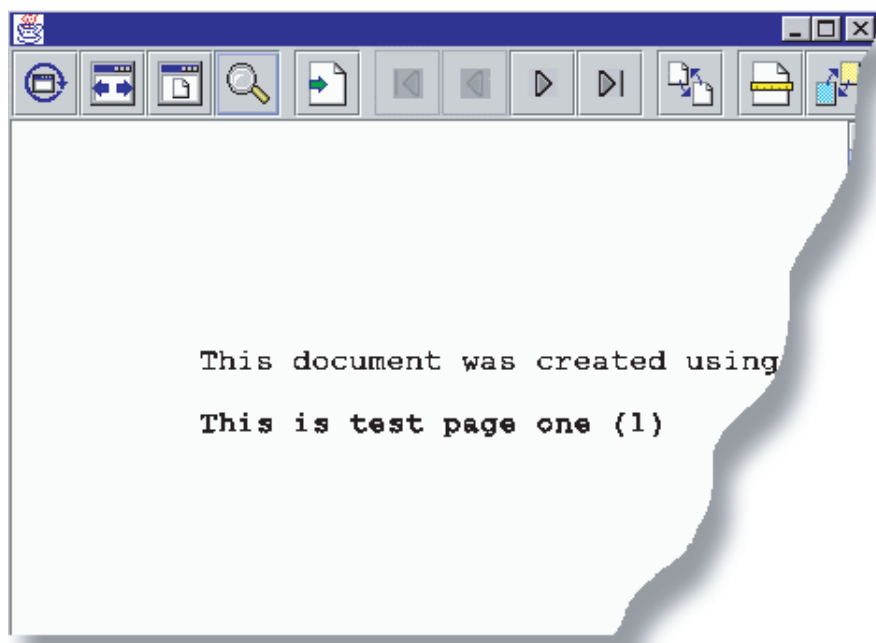
図 1: SpoiledFileViewer
