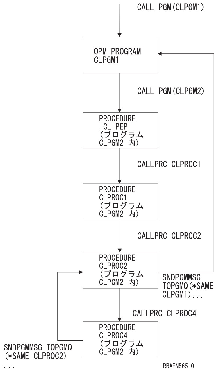
図 18. 基本項目としての単純名の使用例
