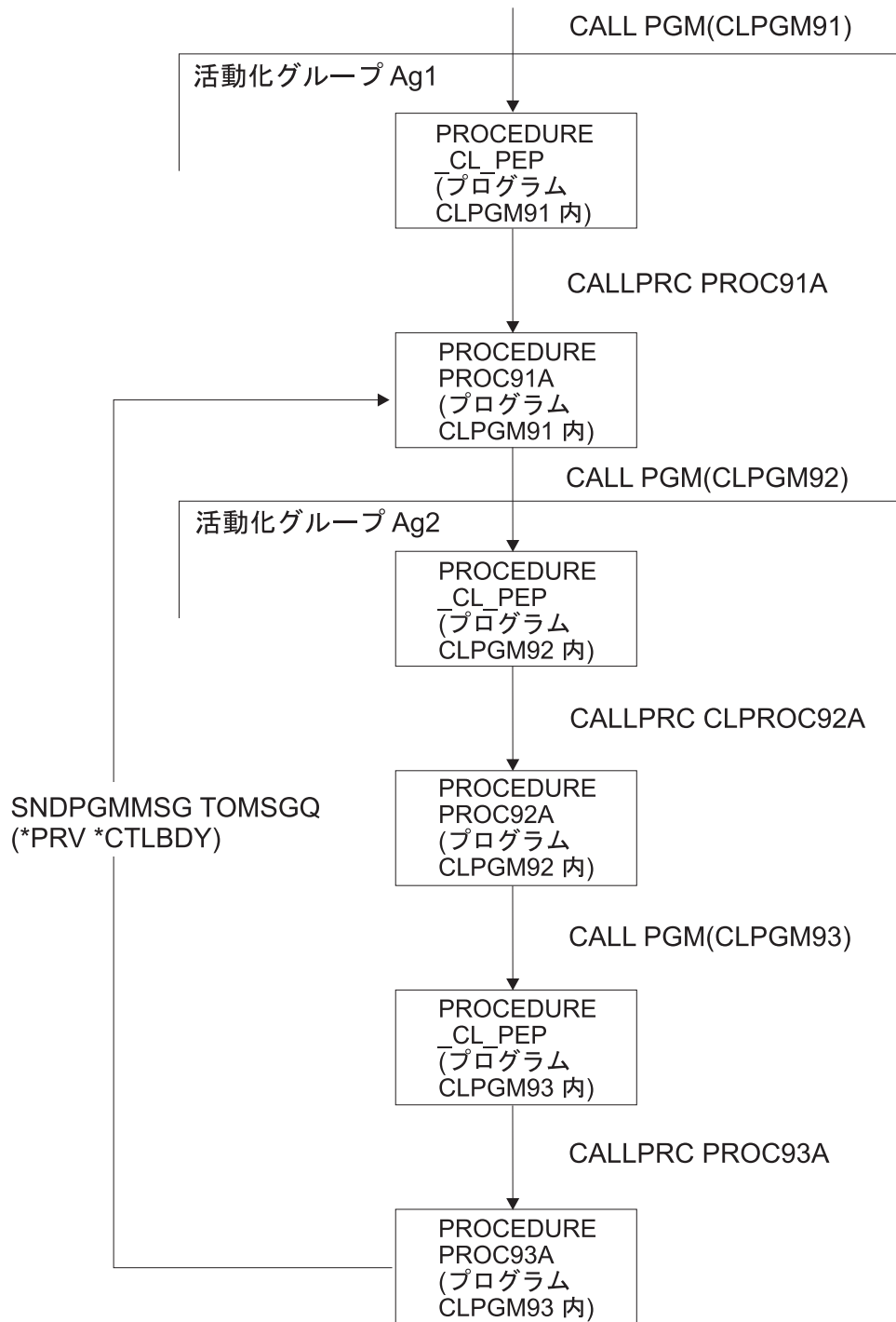
図 24. *CTLBDY の使用例
