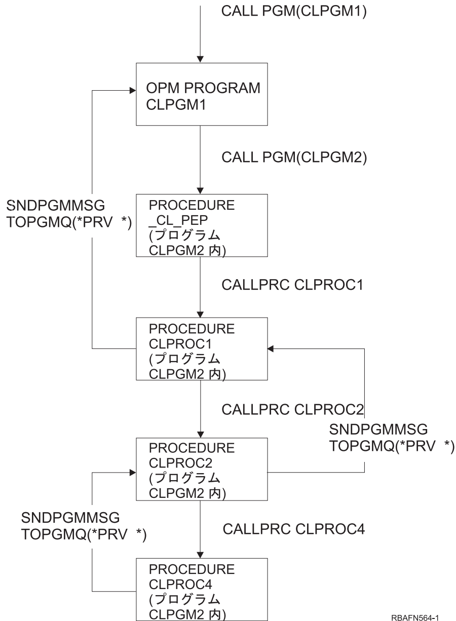
図 17. TOPGMQ(*PRV *) の例
