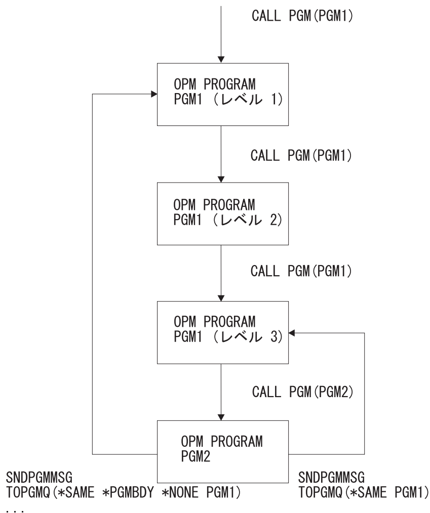
図 22. 再帰を伴った OPM 名を持つ *PGMBDY の使用例
