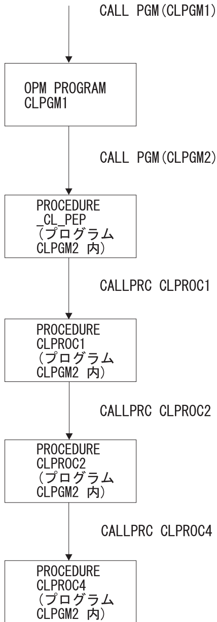
図 16. OPM プログラムを持つランタイム呼び出しスタックおよび複数プロシージャを持つ ILE プログラムの例
