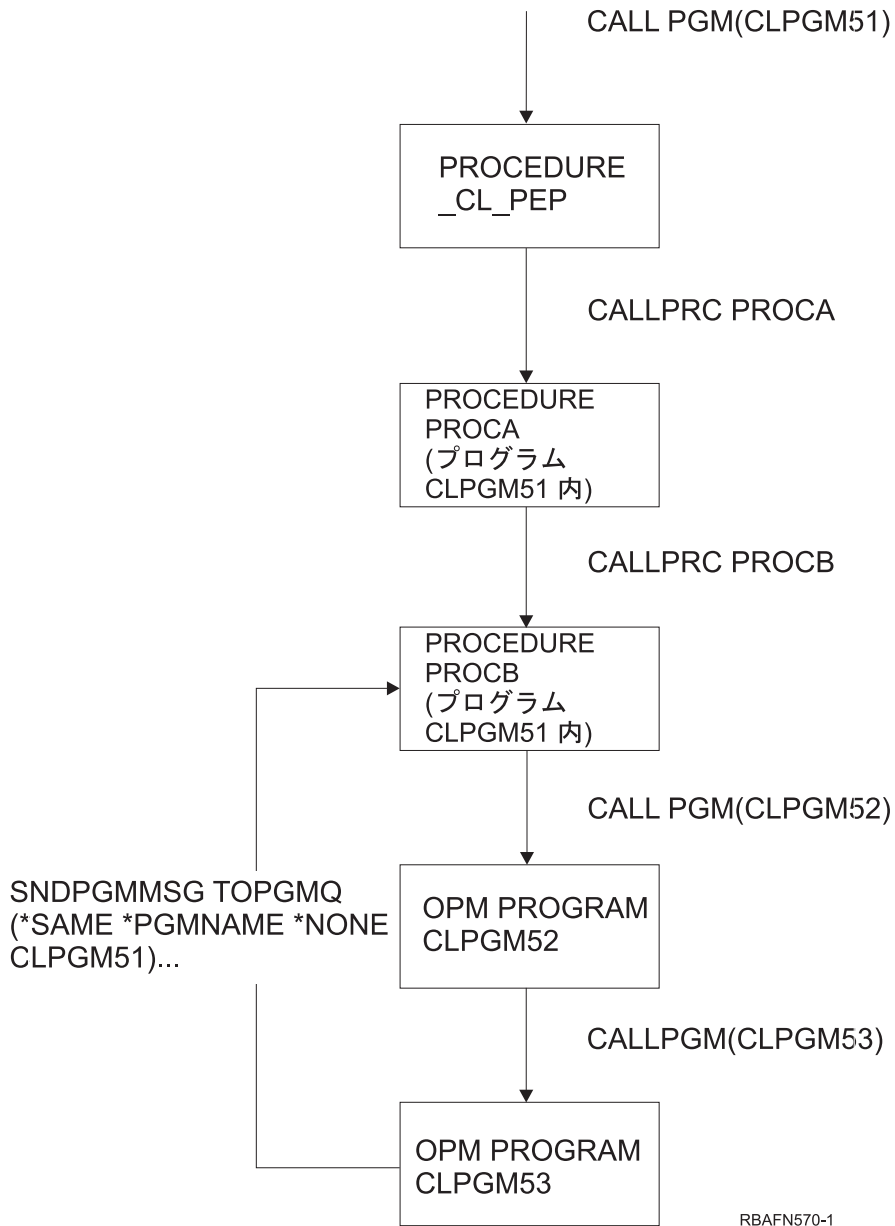
図 23. *PGMNAME の例
