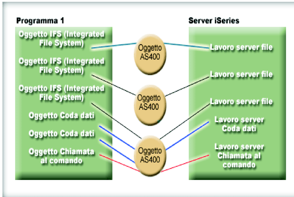
Figura 1: esempio di programma Java che crea più oggetti AS400 e collegamenti socket per lo stesso server iSeries
