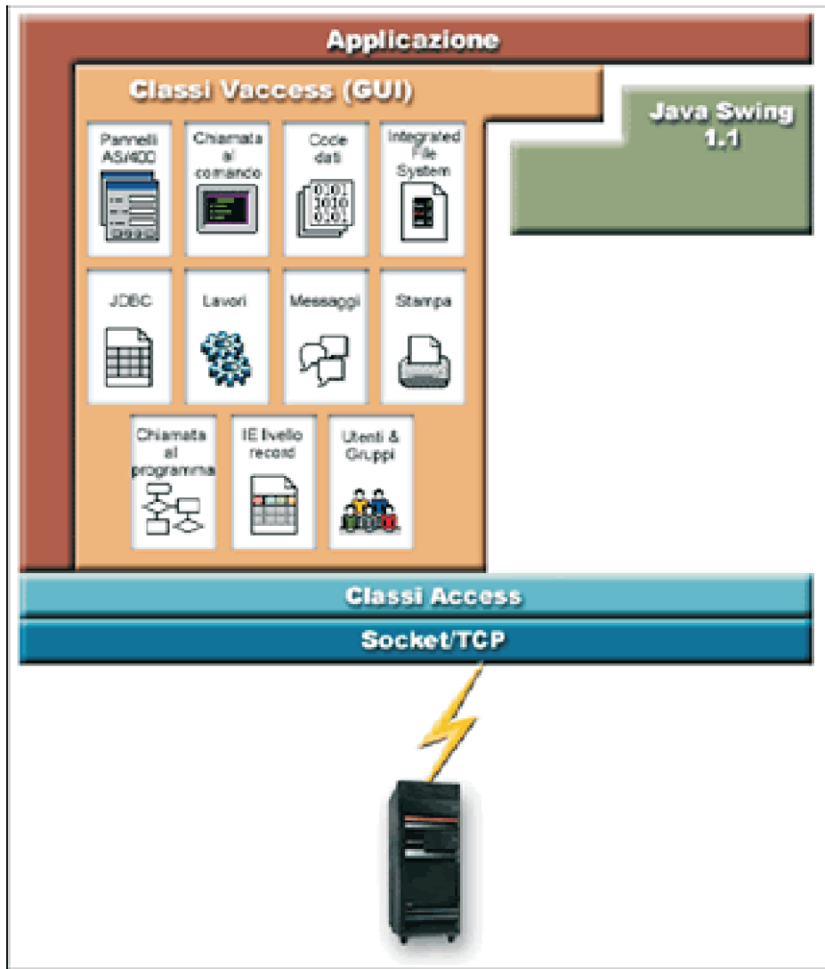
Figura 1: classi Vaccess (rzahh508.gif)”
