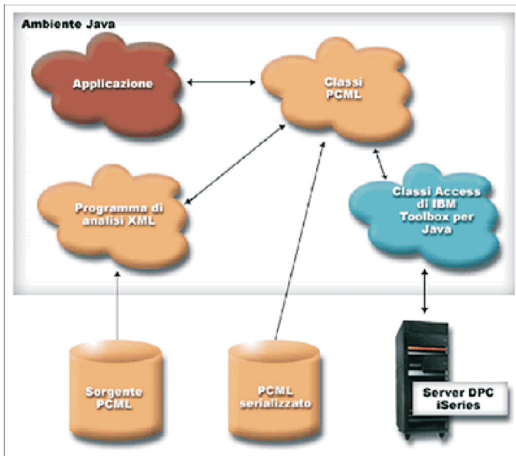
Figura 1. Esecuzione di chiamate al programma utilizzando PCML.
