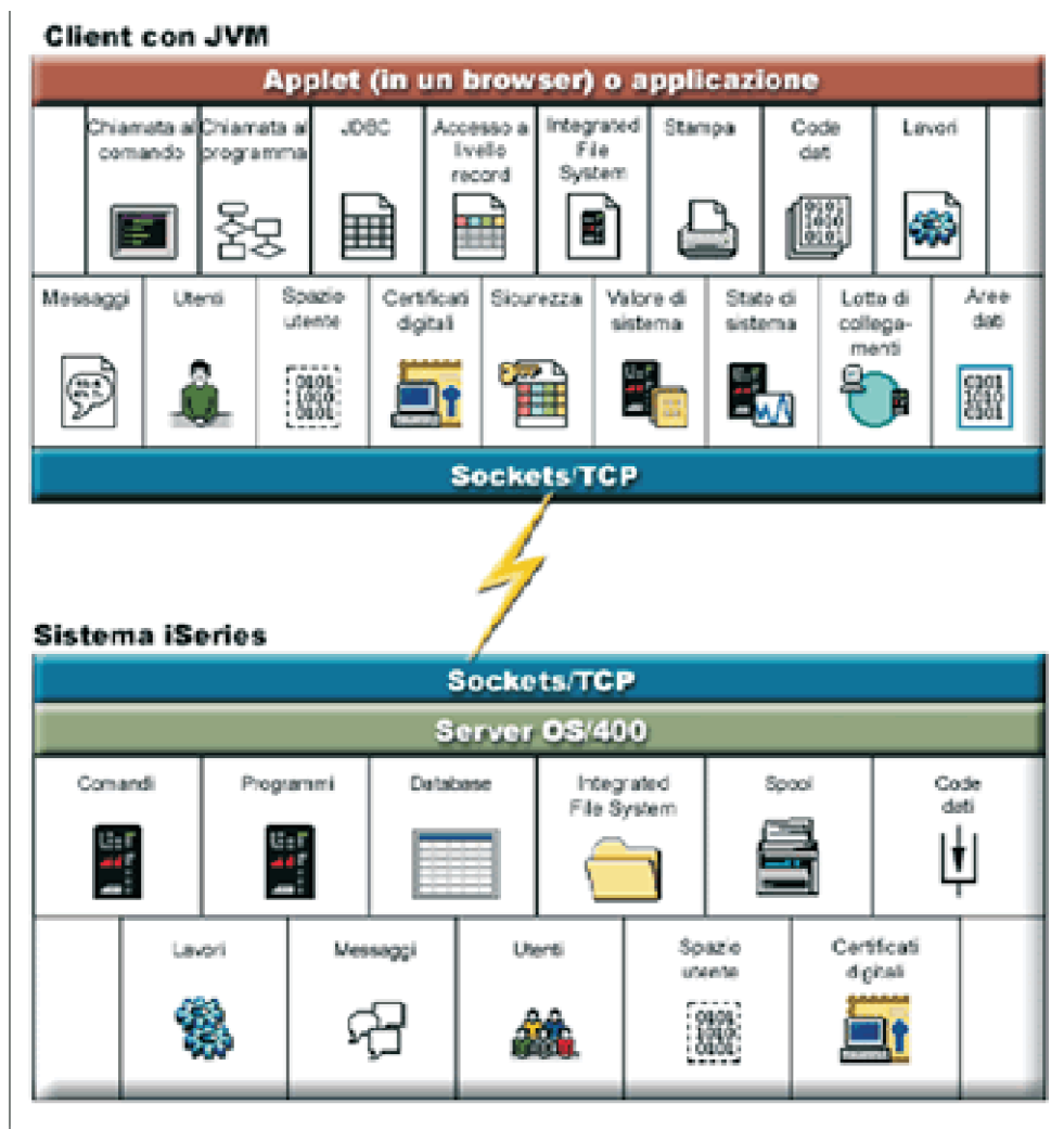
Figura 1: punti di accesso al server
