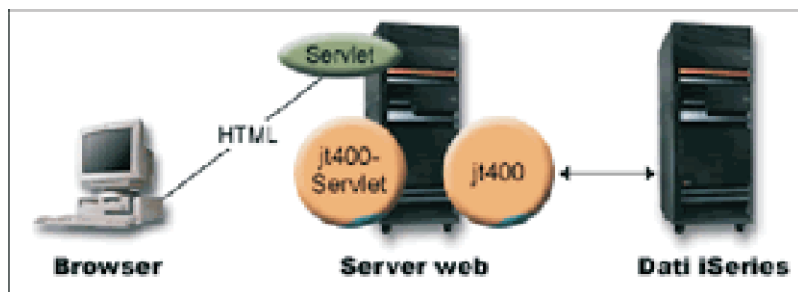
Figura 1: come funzionano i servlet
