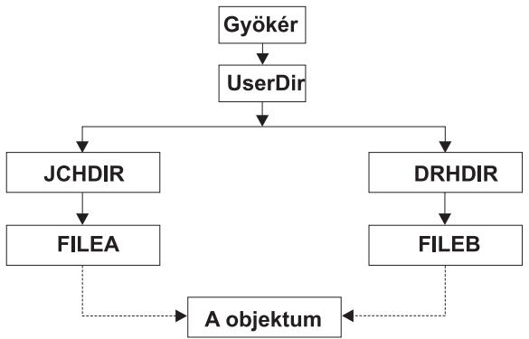
3. ábra: Objektumok közvetlen hivatkozásokkal - Példa
