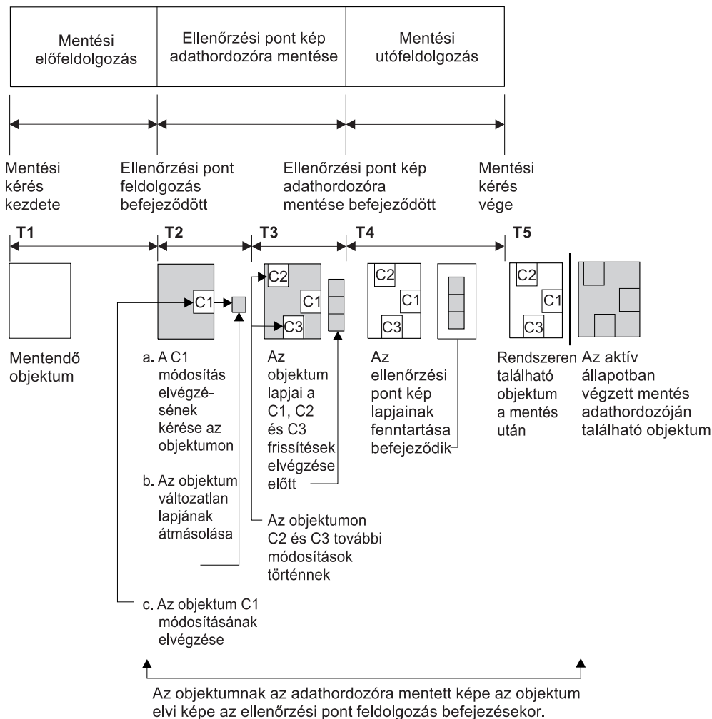
6. ábra: Az ellenőrzési pont feldolgozáson túljutott objektumok módosításainak szerverszintű kezelése
