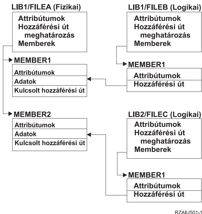
2. ábra: Hozzáférési utak mentése
