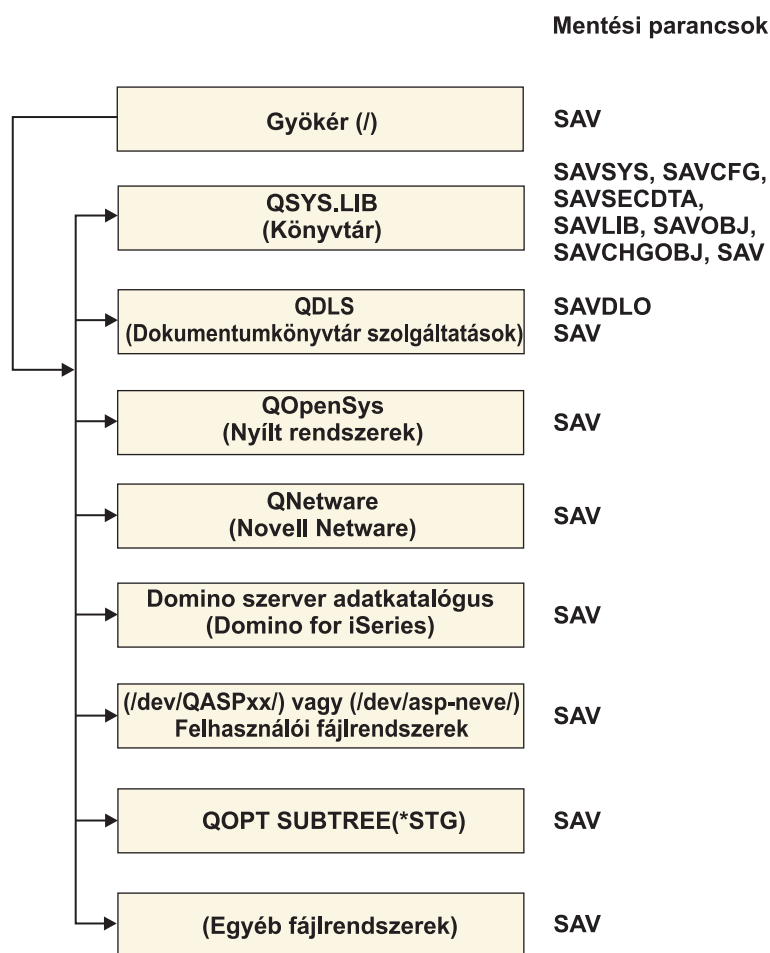
5. ábra: Fájlrendszerek - Mentési parancsok
