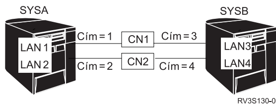
3. ábra: Hibátlan konfiguráció, két összeköttetési hálózat és két LAN vonal
