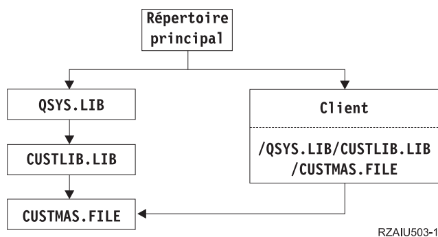
Figure 4. Objet avec un lien symbolique - Exemple
