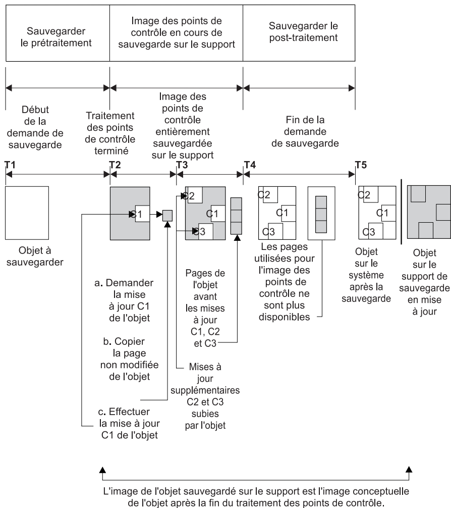
Figure 6. La gestion par le serveur des mises à jour des objets après traitement des points de contrôle est terminée
