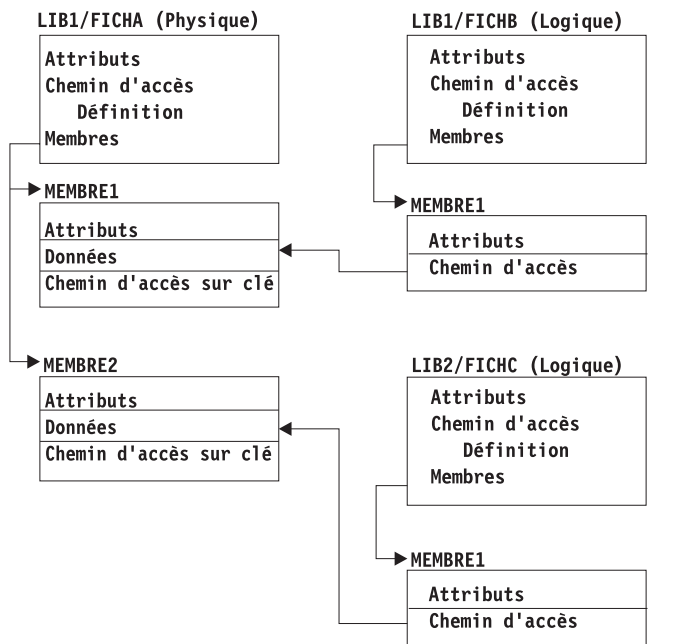
Figure 2. Sauvegarde des chemins d'accès
