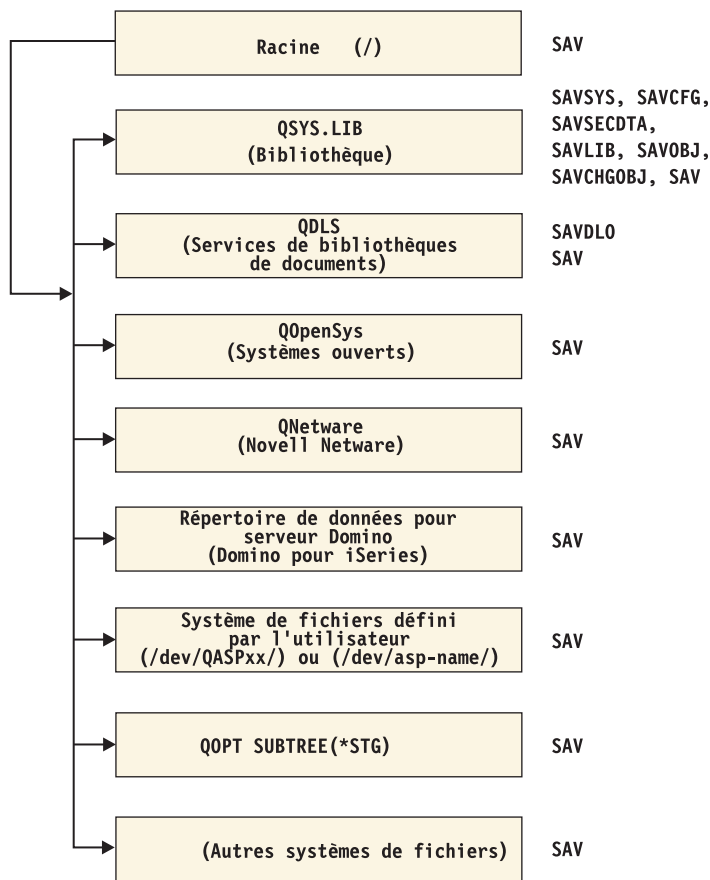
Figure 5. Systèmes de fichiers - Commandes de sauvegarde
