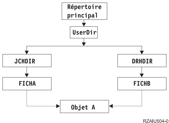
Figure 3. Objet avec des liens fixes - Exemple
