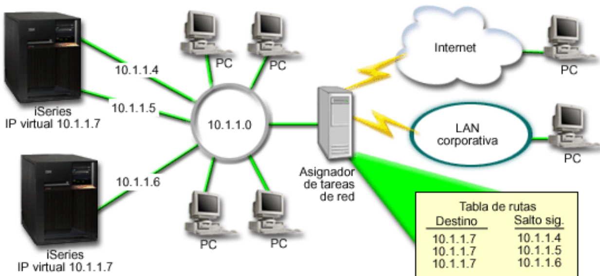
Figura 3. Conmutación por anomalía de adaptador con varios iSeries y clientes locales
