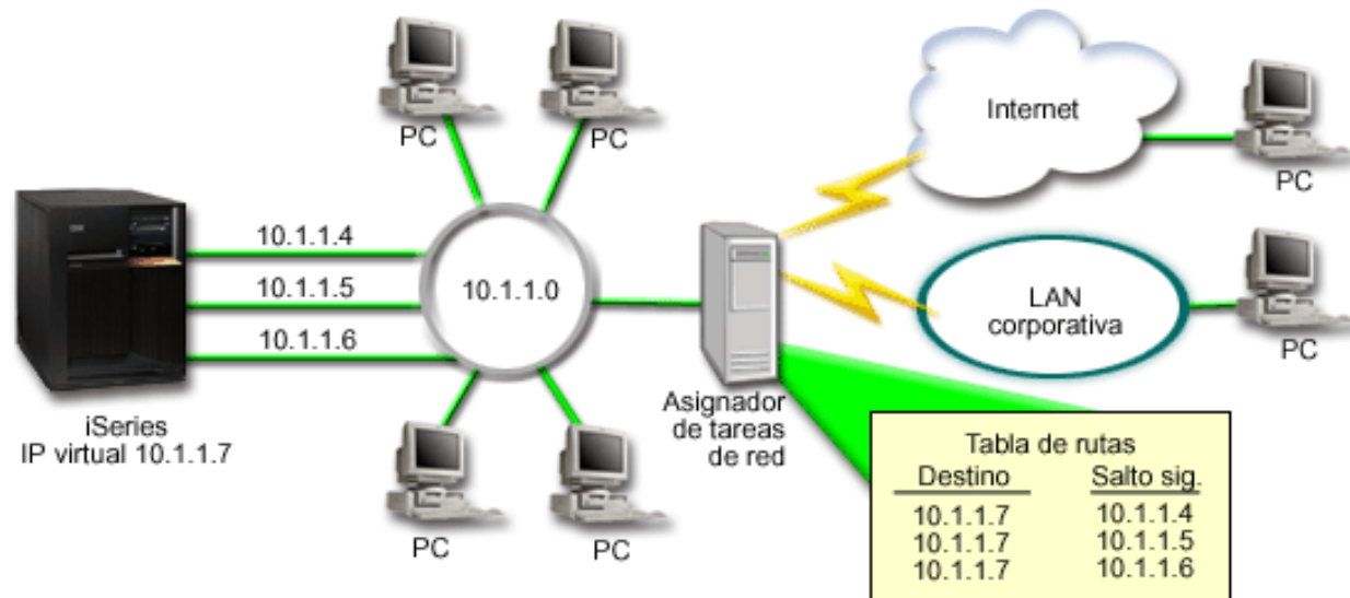
Figura 2. Conmutación por anomalía de adaptador con clientes locales
