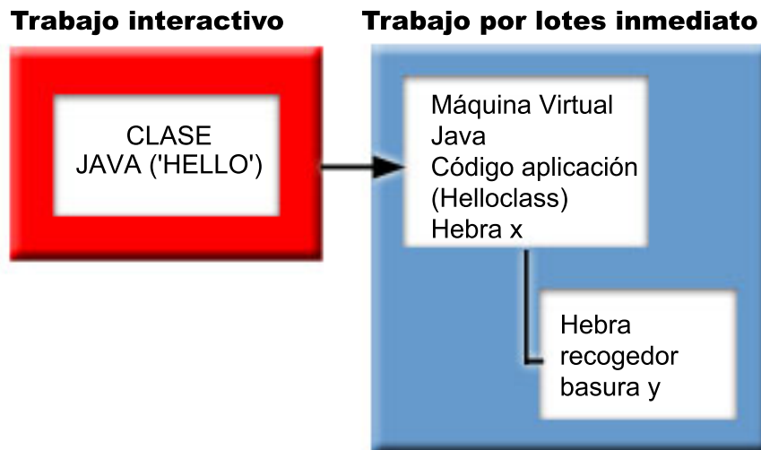
Figura 1: El entorno de Java típico cuando se utiliza el mandato CL RUNJVA or JAVA
