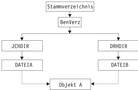
Abbildung 3. Objekt mit festen Verbindungen - Beispiel
