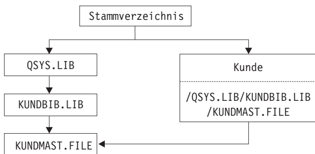
Abbildung 4. Objekt mit einer symbolischen Verbindung - Beispiel
