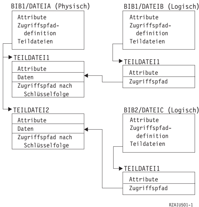
Abbildung 2. Zugriffspfade sichern
