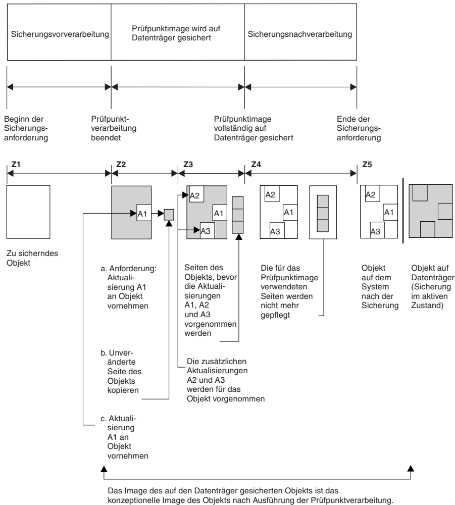
Abbildung 6. Verwaltung der Aktualisierungen an Objekten durch den Server nach der Beendigung der Prüfpunktverarbeitung
