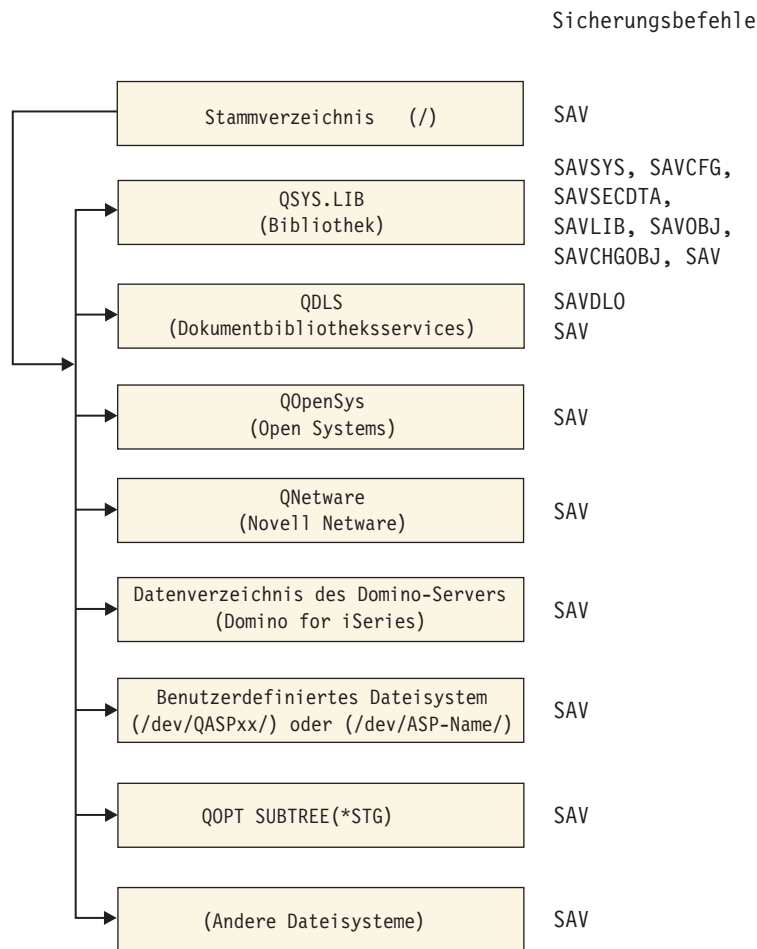
Abbildung 5. Dateisysteme - Sicherungsbefehle
