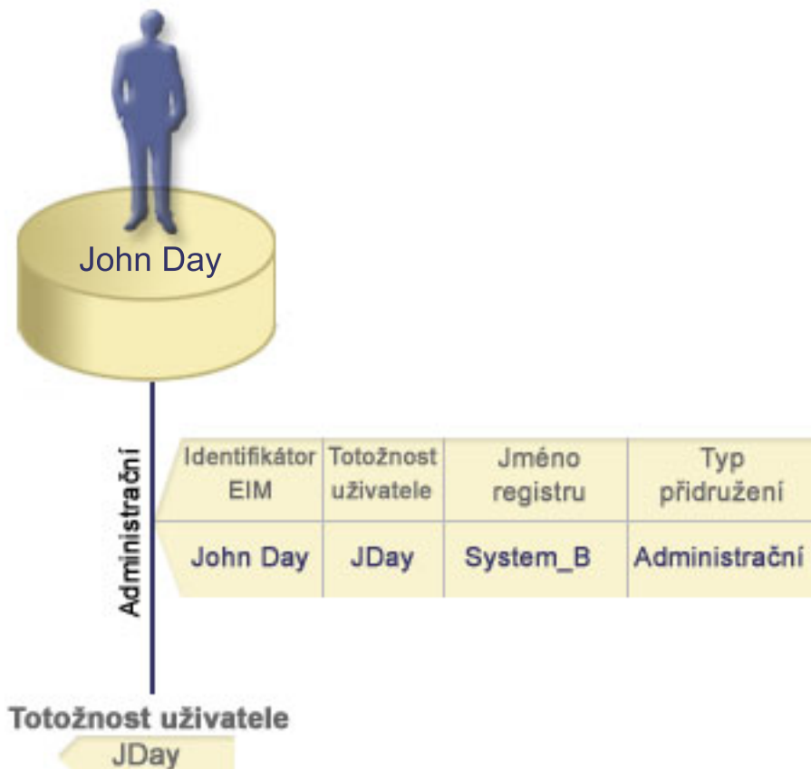
Obrázek č. 7: Administrační přiřazení EIM identifikátoru EIM John Day
