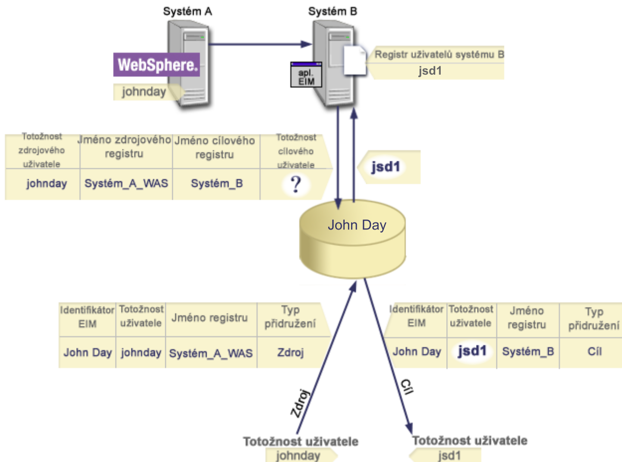
Obrázek č. 11: Vyhledávací operace vrací cílovou totožnost uživatele z daných přidružení identifikátorů na základě známé totožnosti uživatele johnday.
