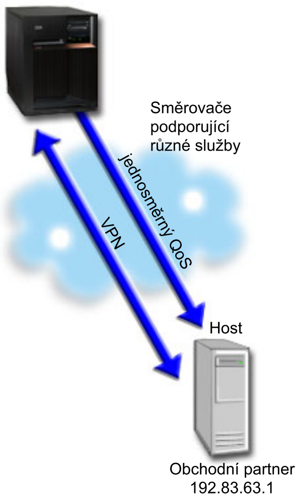
Obrázek 5. Spojení VPN typu host-to-host využívající zásadu odlišovaných služeb QoS.
