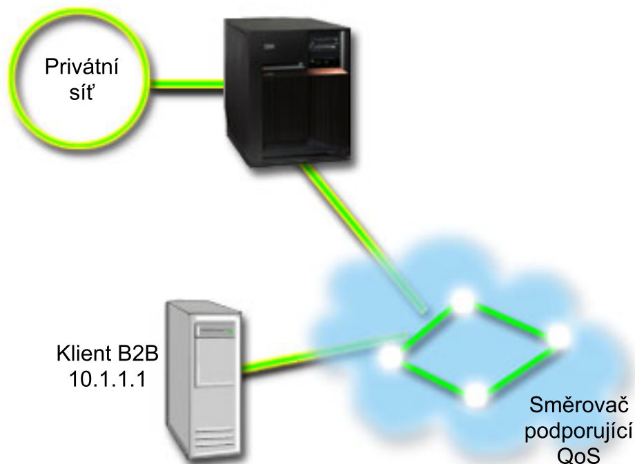
Obrázek 7. Zásada integrovaných služeb QoS pro klienta B2B využívající směrovače s podporou pro RSVP.
