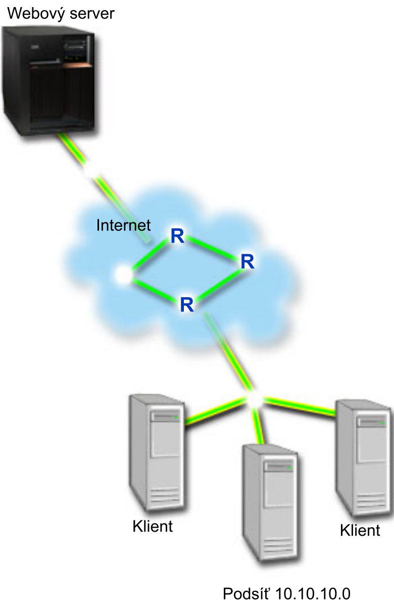
Obrázek 4. Webový server omezující přenos prohlížeče pro určitého klienta.
