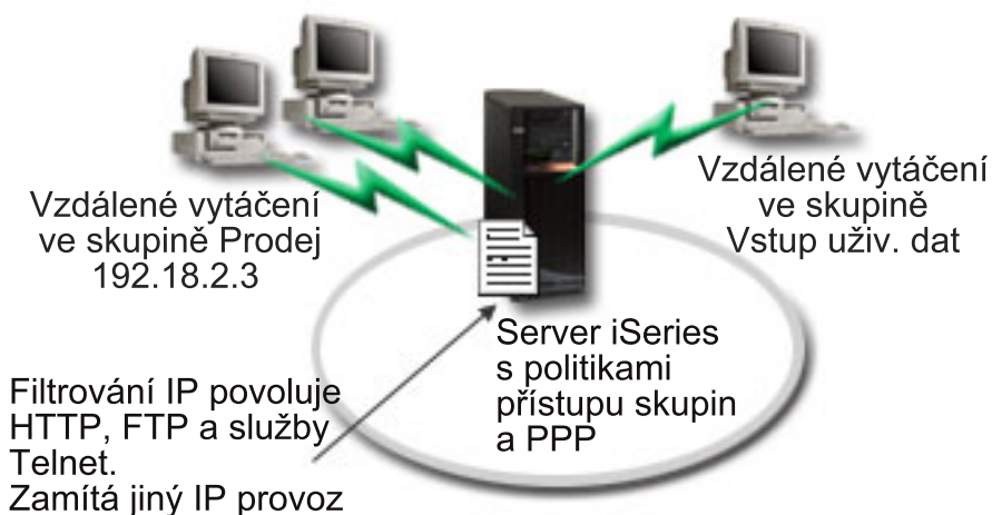
Obrázek 8. Nastavení vytáčených přípojení s uplatněním zásady skupinového nastavení
