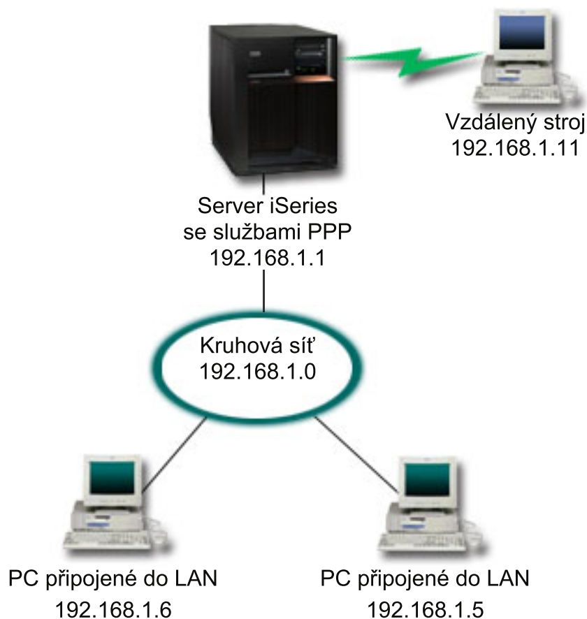
Obrázek 4. Připojení vzdálených klientů k serveru iSeries
