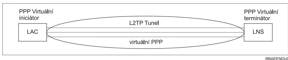
Obrázek 10. PPP virtuální iniciátor nebo PPP virtuální terminátor
