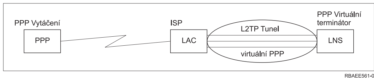
Obrázek 11. PPP iniciátor vytáčení nebo PPP virtuální terminátor
