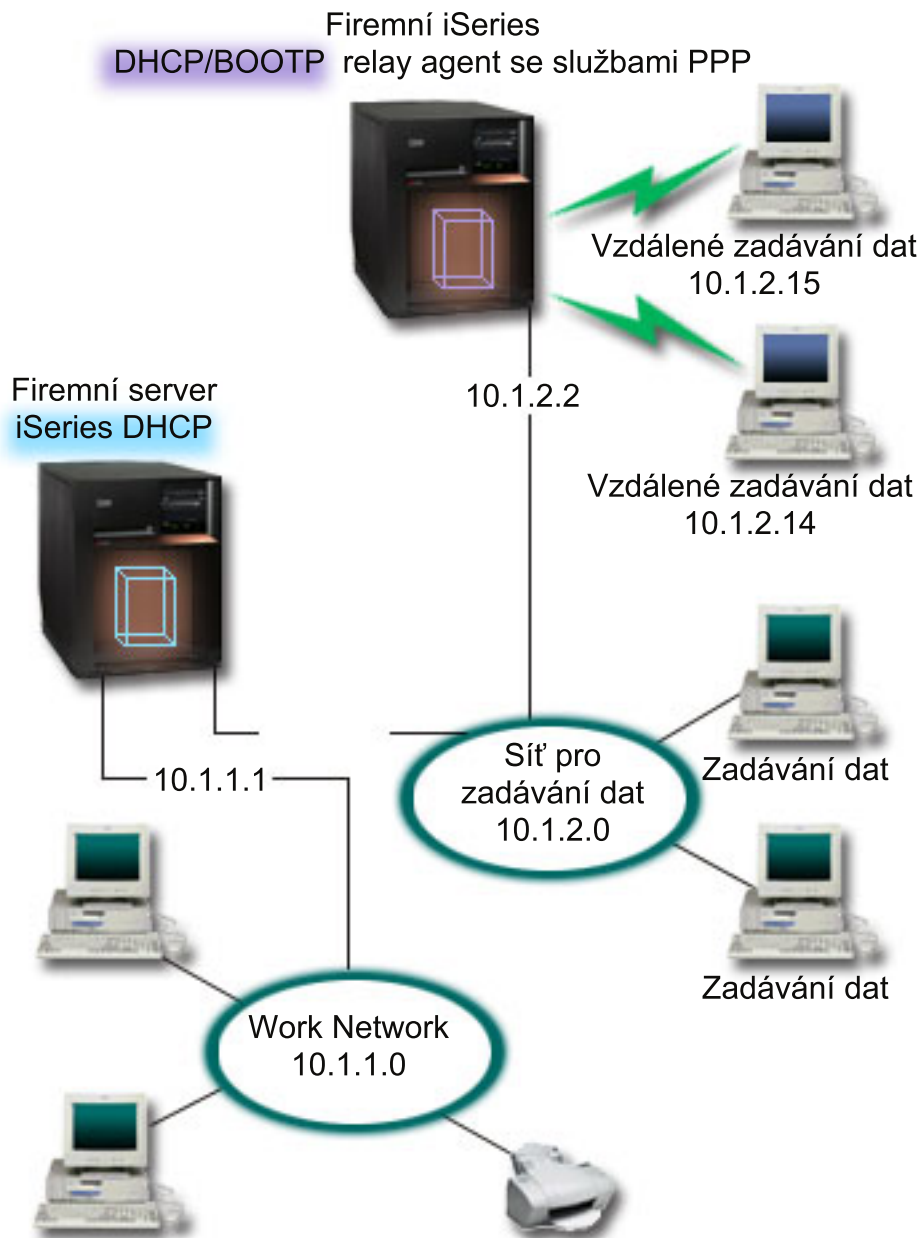
Obrázek 2. Profil DHCP a PPP na různých serverech iSeries
