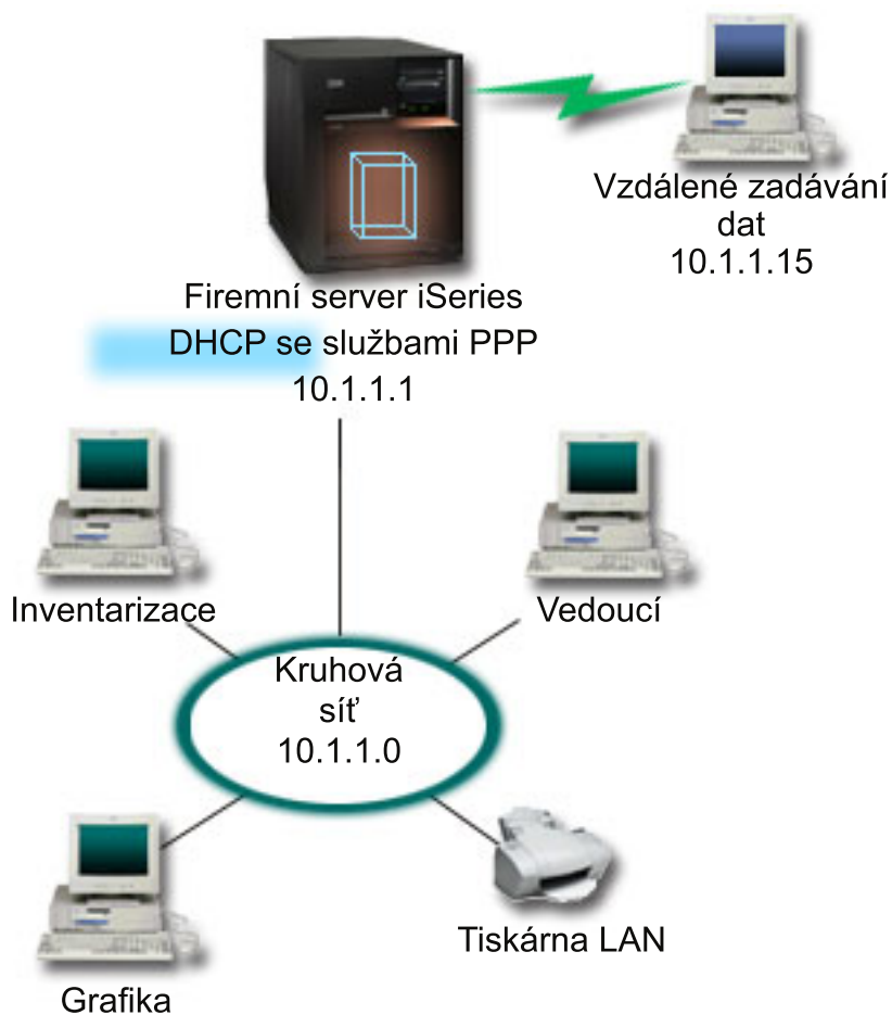
Obrázek 1. PPP a DHCP na jediném serveru iSeries
