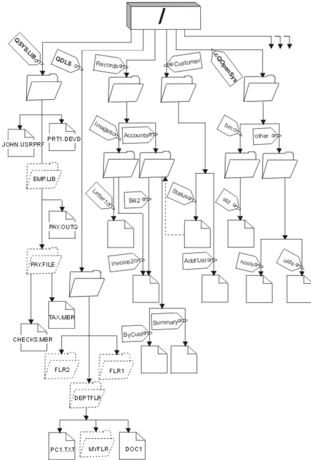
图 3. 文件系统和对象是集成文件系统目录树上的分支
