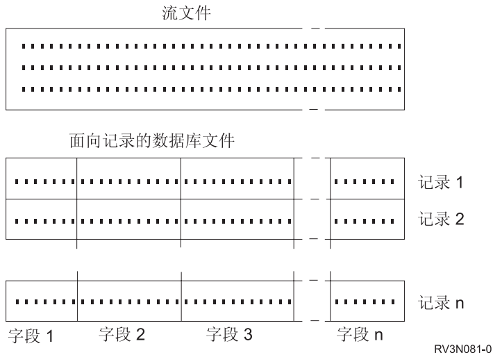
图 7. 比较流文件和面向记录的文件
