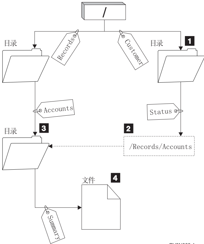
图 5. 使用符号链接的示例
