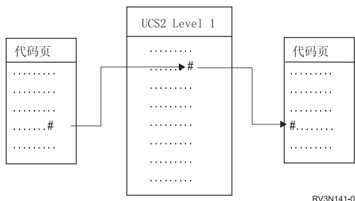
图 8. 使字符在各种编码方案中都相同
