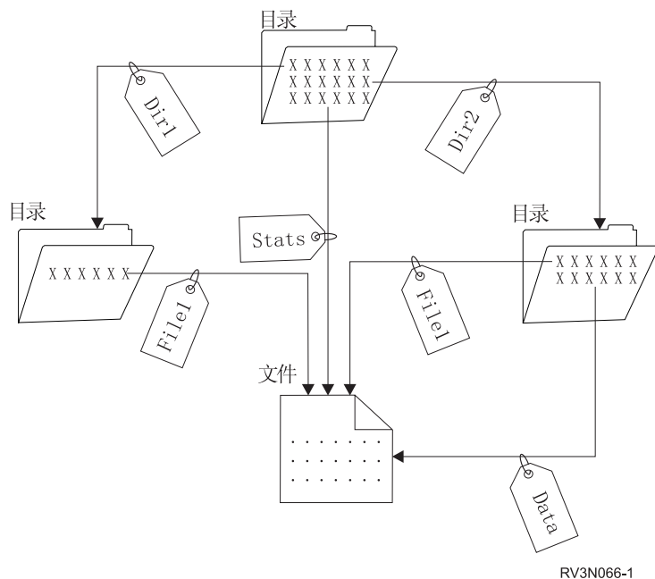
图 4. 目录项定义每个硬链接。
