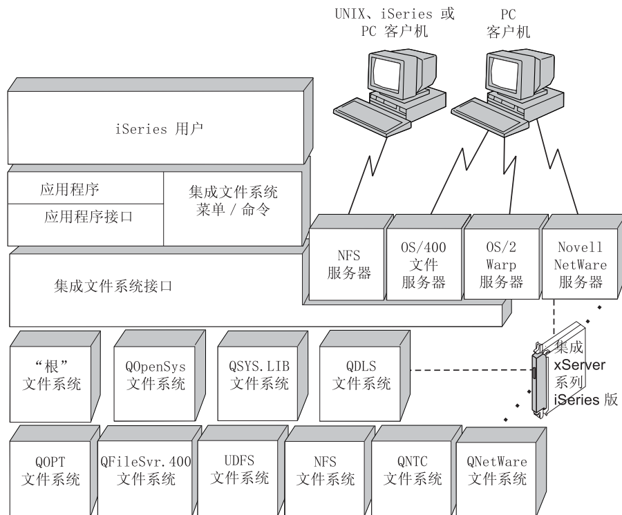
图 9. 文件系统、文件服务器和集成文件系统接口
