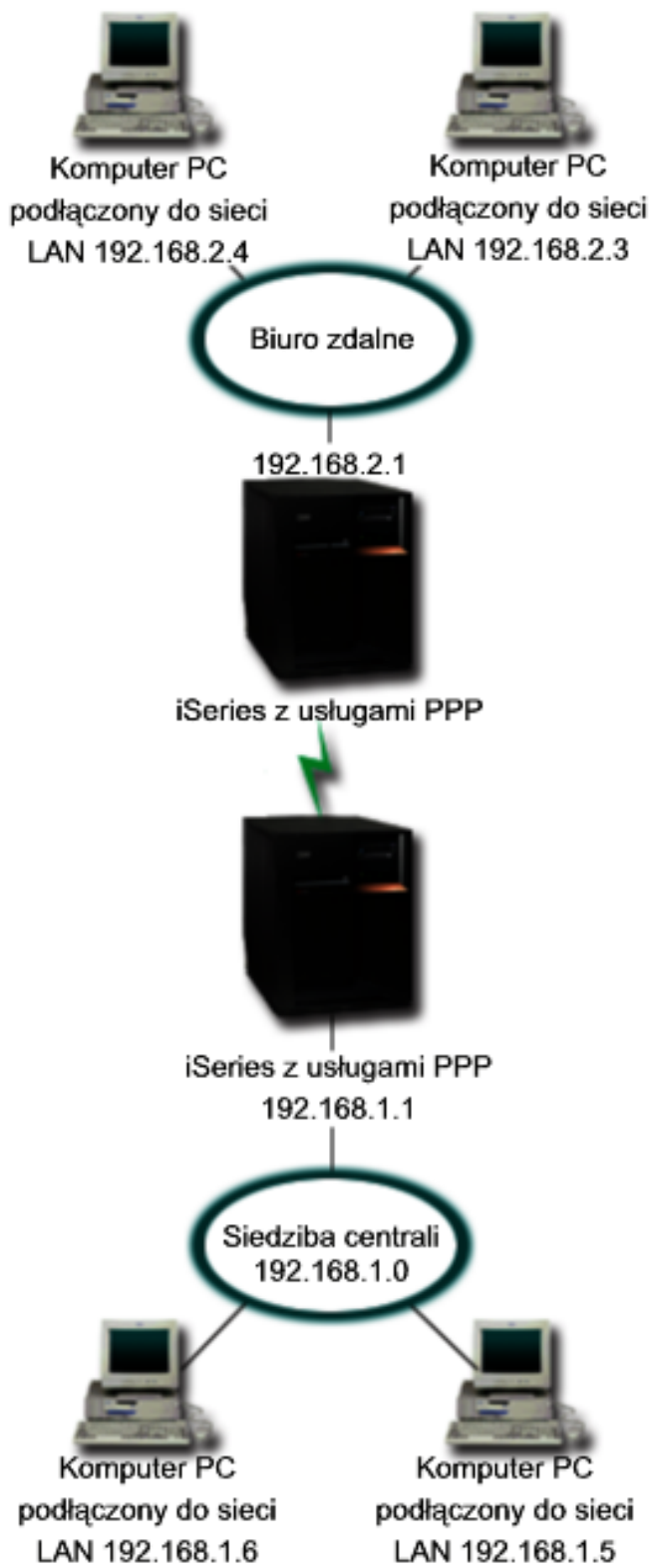
Rysunek 4. Łączenie sieci LAN z sieciami zdalnymi za pomocą modemu
