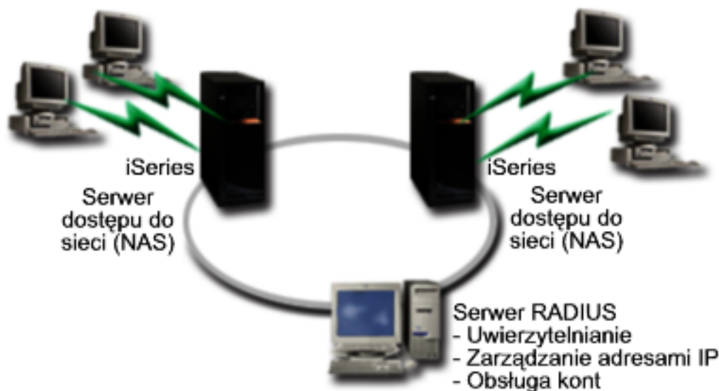
Rysunek 5. Uwierzytelnianie połączeń modemowych za pomocą serwera RADIUS
