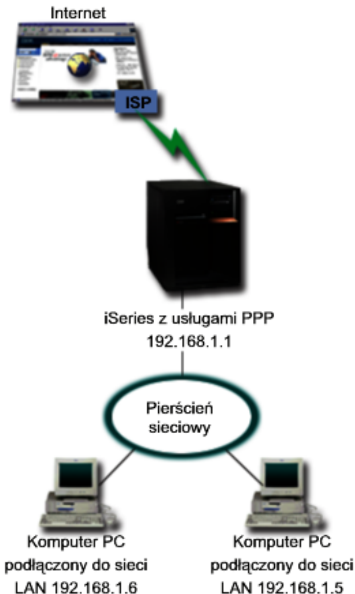
Rysunek 3. Łączenie sieci LAN z Internetem przy pomocy modemu
