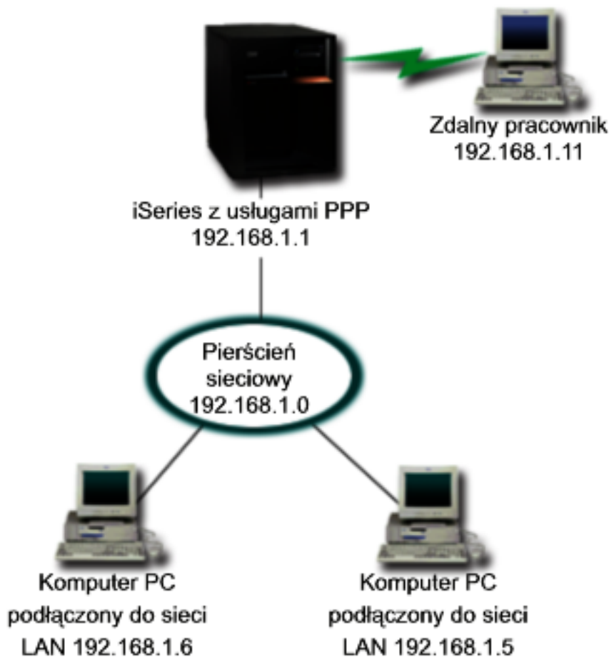
Rysunek 2. Łączenie zdalnych klientów z serwerem iSeries
