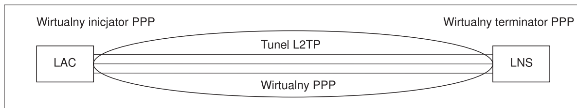
Rysunek 7. Wirtualny inicjator PPP lub wirtualny terminator PPP
