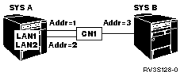
Rysunek 1. Niepoprawna konfiguracja, równoległe grupy TG w sieci połączeń
