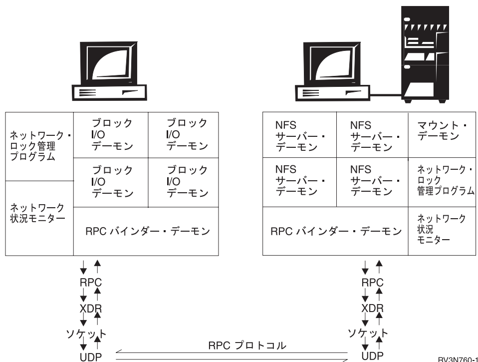
図7. NFS クライアント / サーバー・プロトコルの内訳
