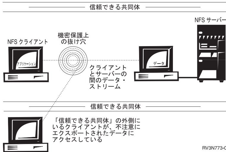
図 57. 信頼できる共同体の外側にいるクライアントが機密保護上の抜け穴を作る
