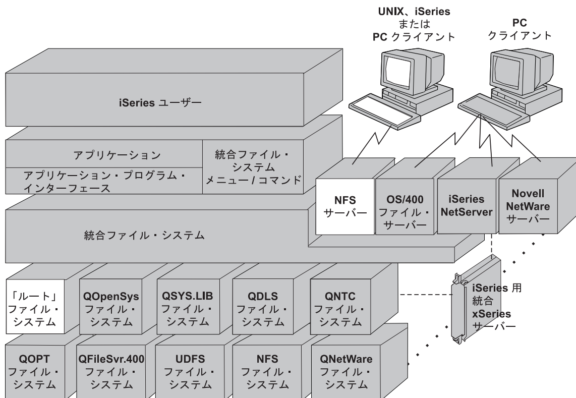
図 46. NFS サーバー経由でアクセスされる「ルート」(I) ファイル・システム
