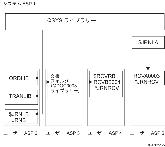
図 9. 独立ジャーナル・レシーバー回復後のユーザー ASP 構成
