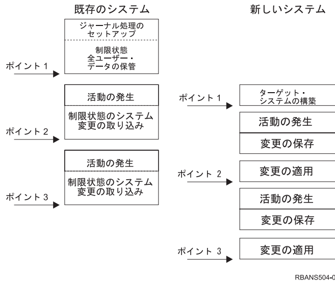
図 30. 同期化処理の概要
