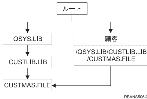
図 24. シンボリック・リンクをもつオブジェクトの例
