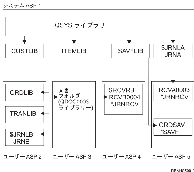
図 6. 障害前のユーザー ASP 構成
