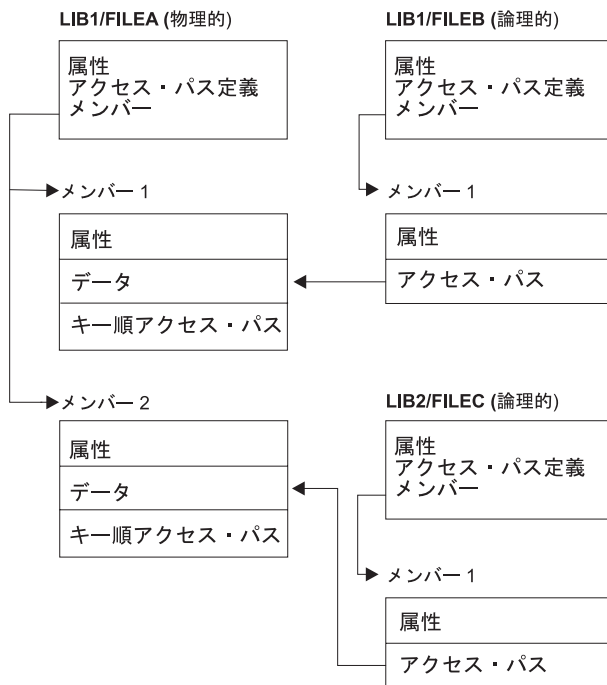
図 21. アクセス・パスの復元
