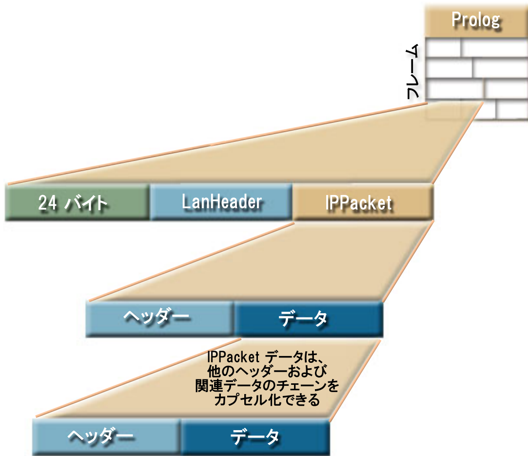
図 1: Commtrace モデル
