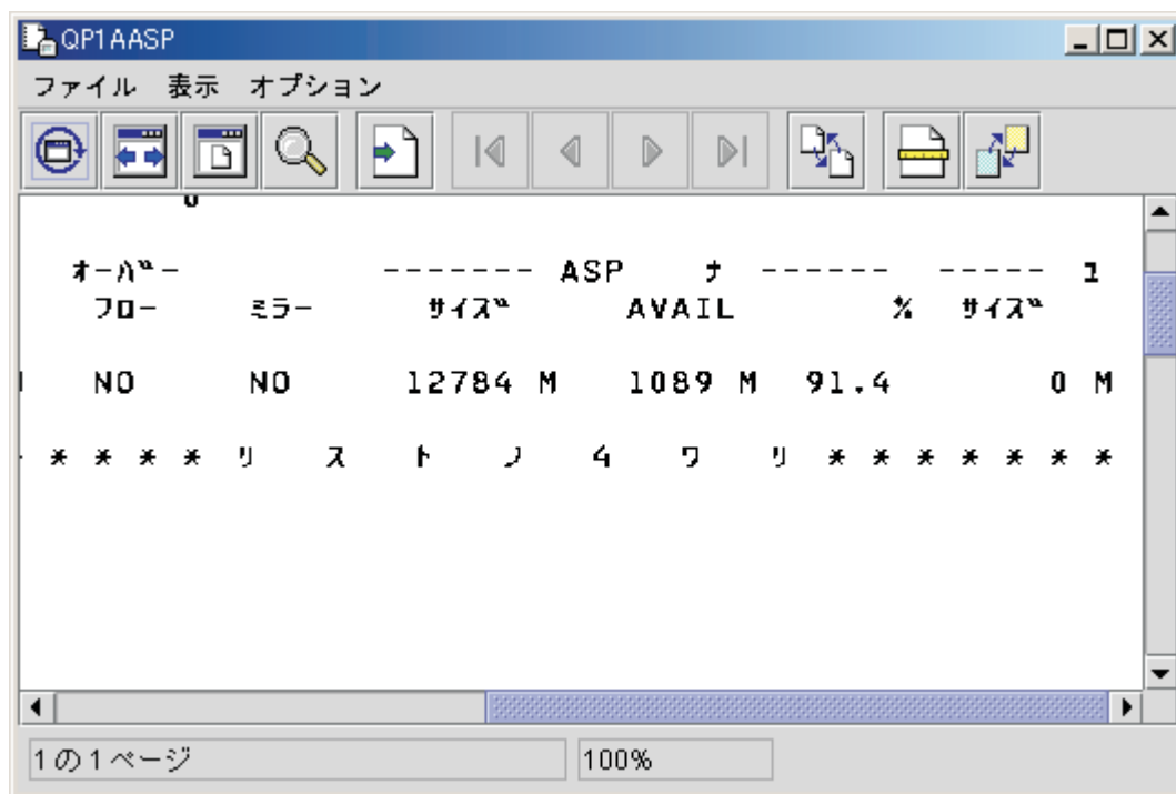
図 1: SpooledFileViewer
