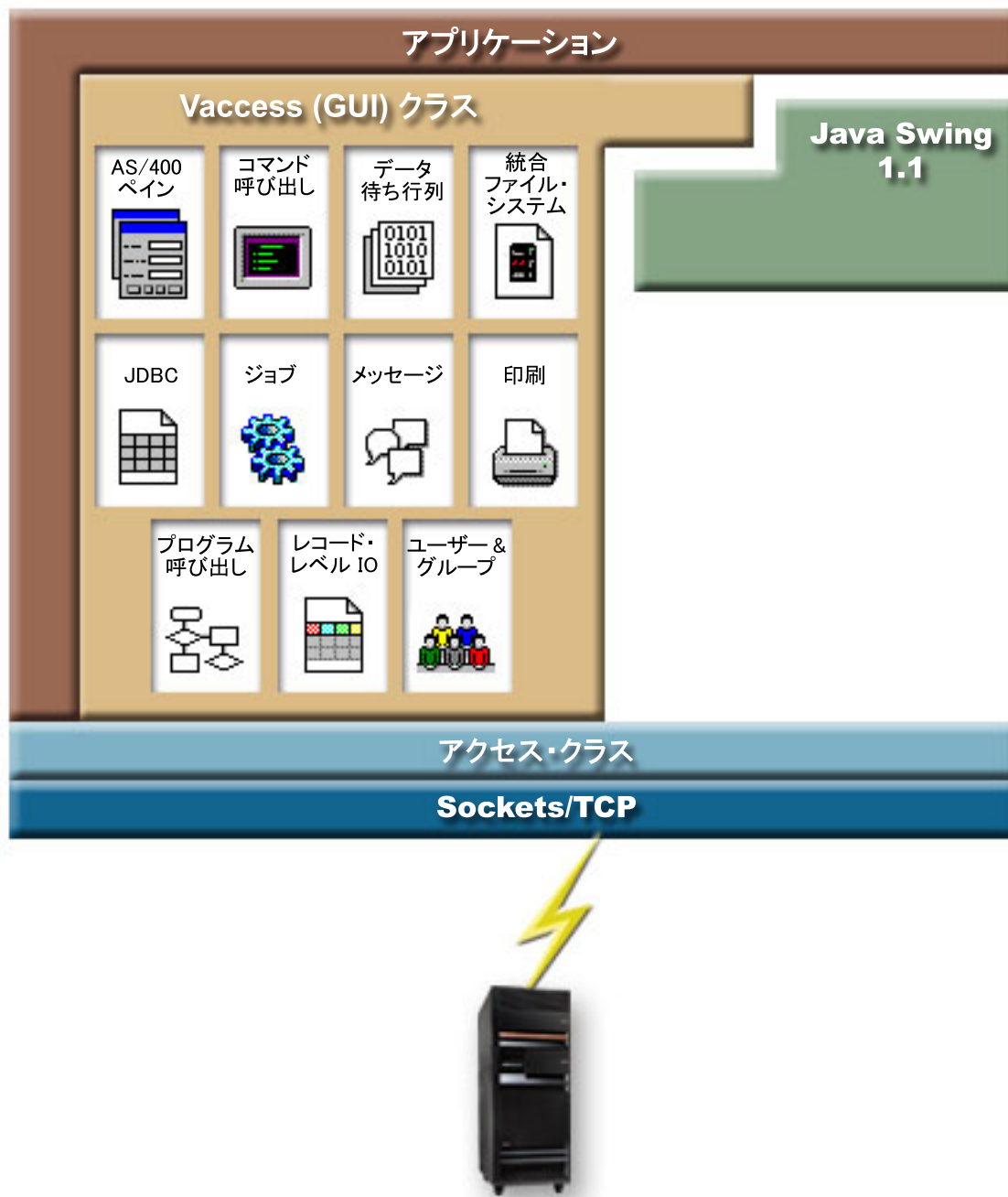
図 1: Vaccess クラス
