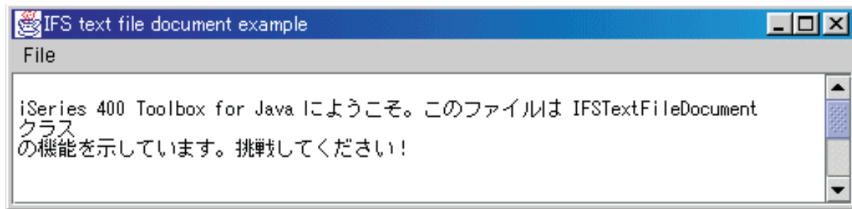
図 1: IFSTextFileDocument の例
