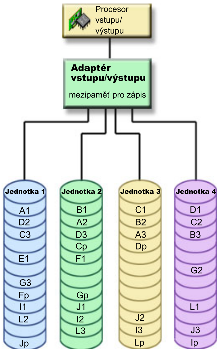
Obrázek 2. Příklad distribuce paritních dat při použití adaptérů IOA verze vyšší než V5R2 a ochrany pomocí RAID
