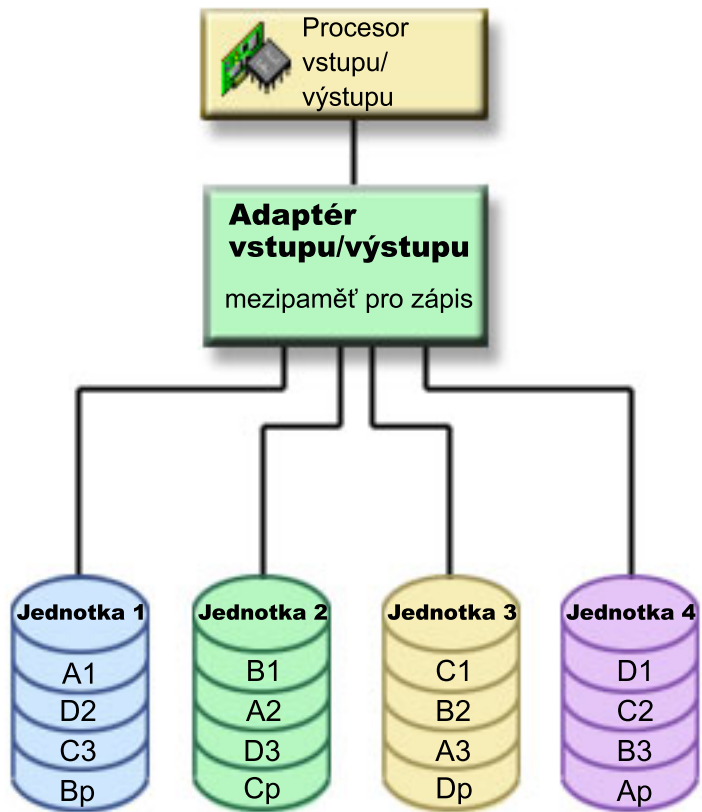
Obrázek 1. Příklad distribuce paritních dat při použití adaptérů IOA verze nižší než V5R2 a ochrany pomocí RAID
