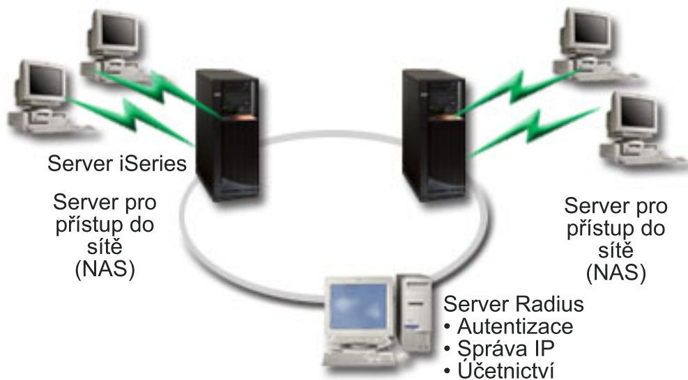
Obrázek 5. Autentizace vytáčených připojení pomocí serveru RADIUS
