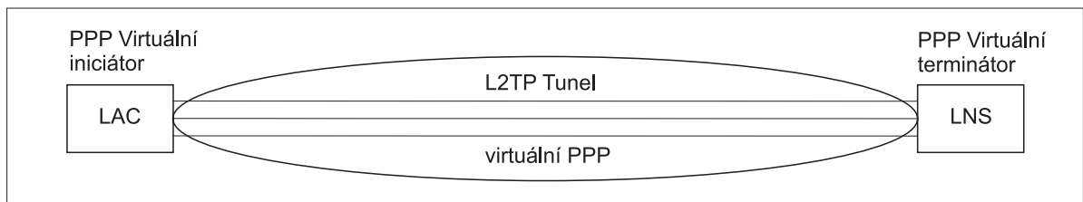
Obrázek 7. PPP virtuální iniciátor nebo PPP virtuální terminátor
