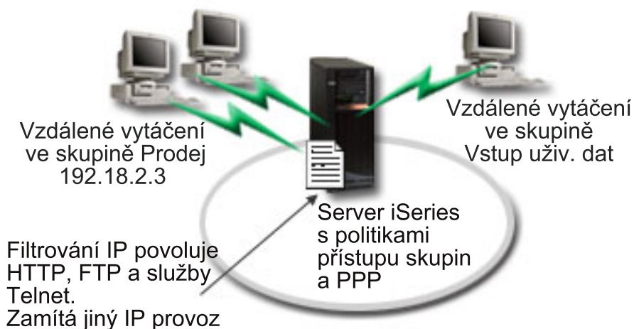
Obrázek 6. Nastavení vytáčených připojení s uplatněním zásady skupinového nastavení
