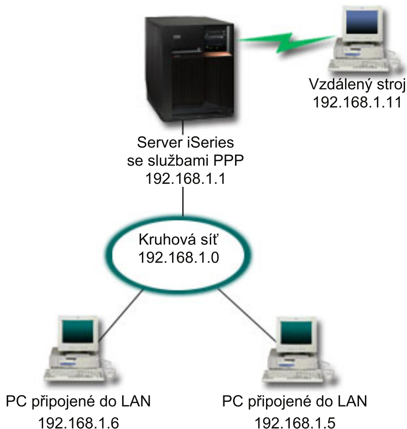
Obrázek 2. Připojení vzdálených klientů k serveru iSeries
