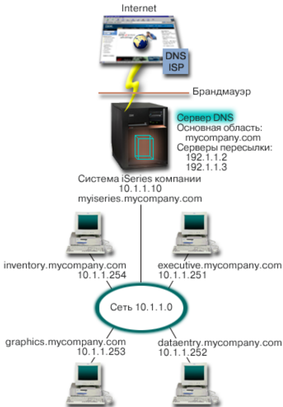
Рисунок 5. Сервер DNS, подключенный к Internet.
