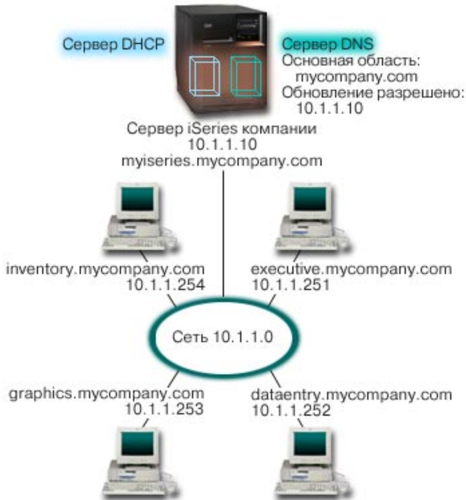
Рисунок 3. Серверы DNS и DHCP, расположенные в одной системе iSeries.
