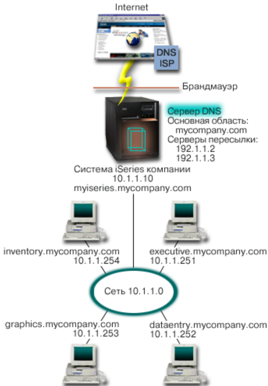
Рисунок 2. Сервер DNS, подключенный к Internet.
