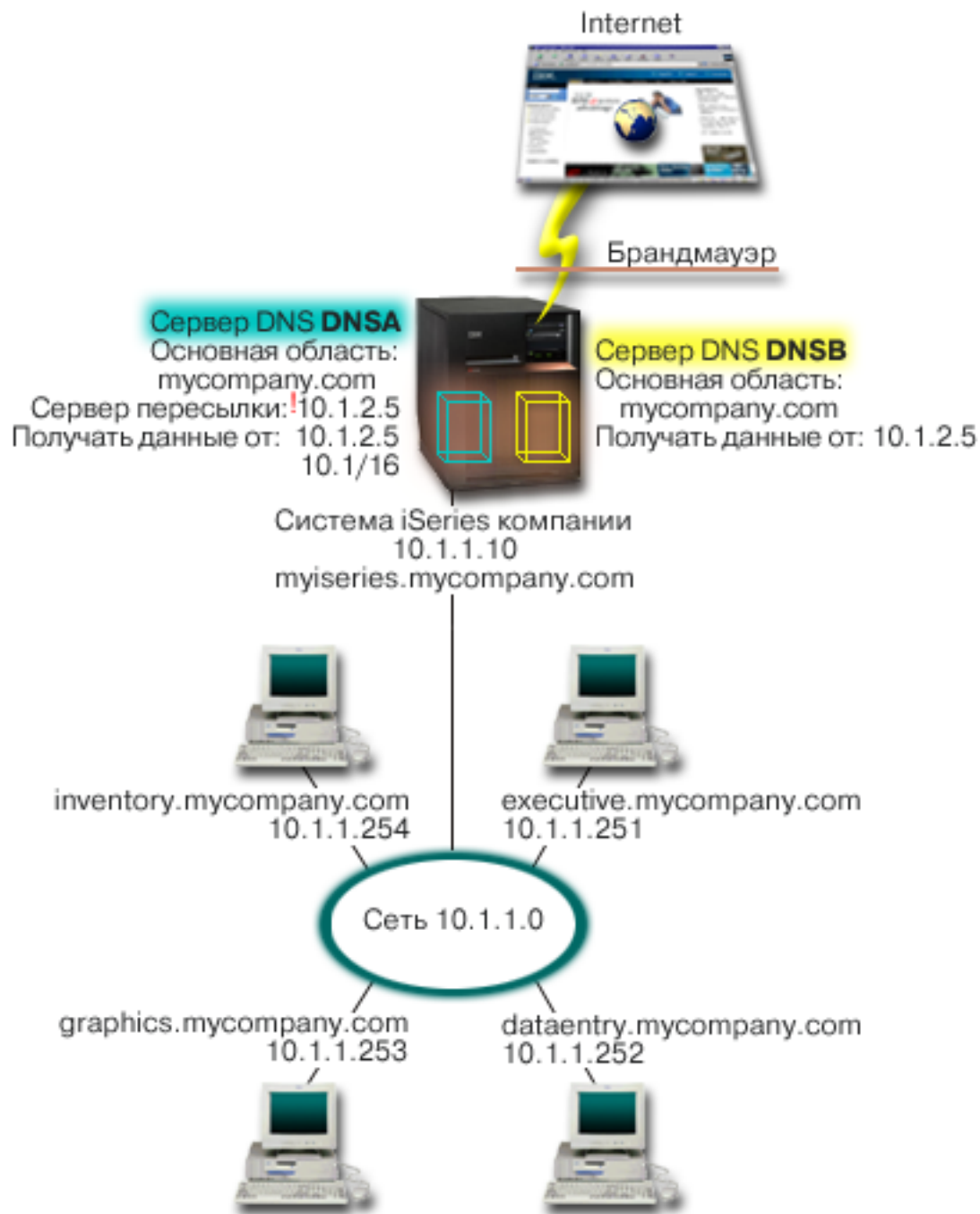
Рисунок 4. DNS с разделенной областью ответственности в сети с брандмауэром.
