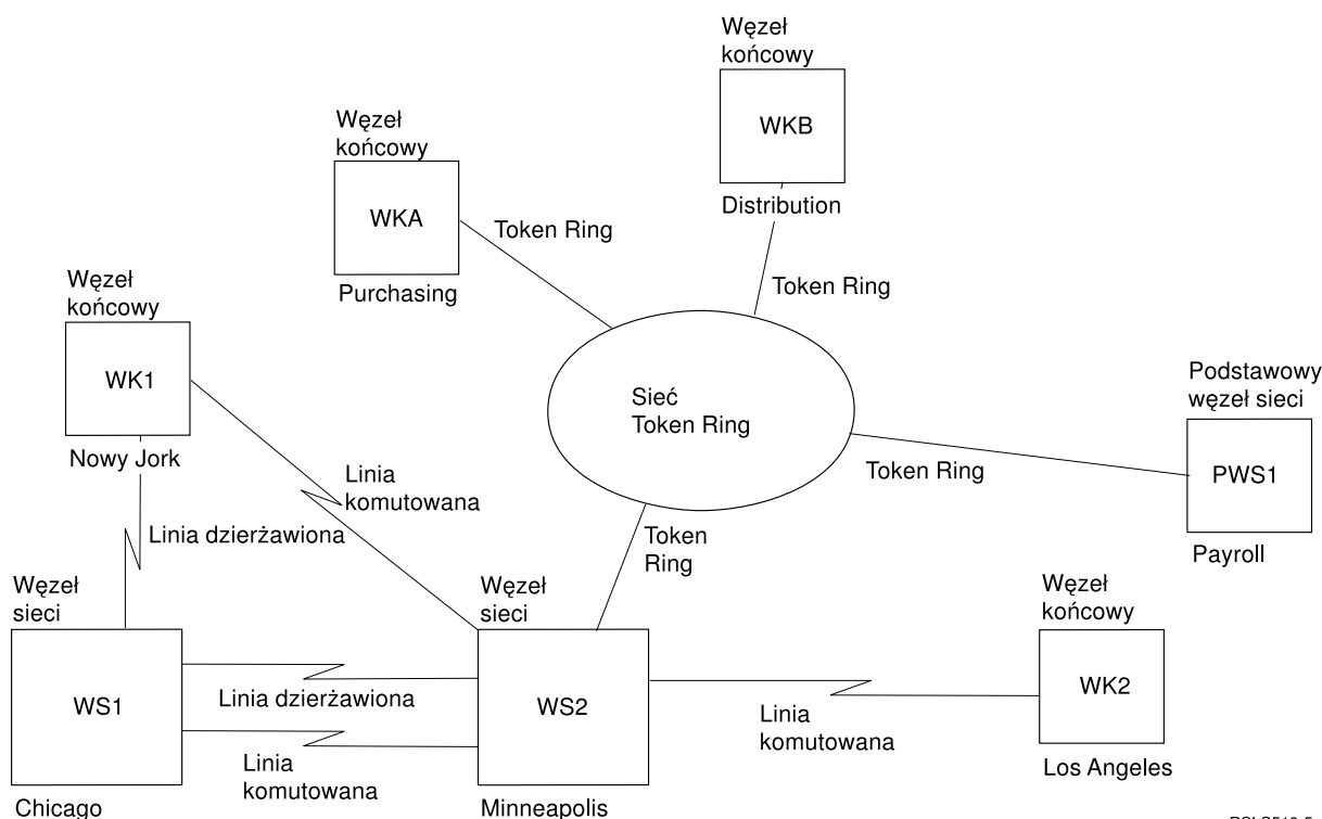
Rysunek 8. Kilka systemów iSeries używających komunikacji APPN
