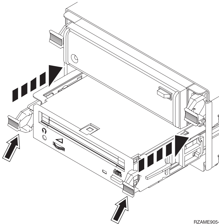
Figuur 4. Het CD-ROM- of bandstation installeren.
