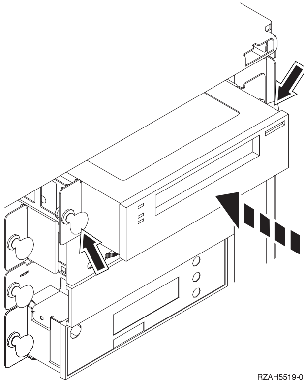
Figuur 2. Verwisselbare media installeren
