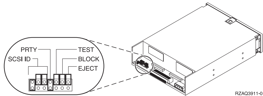
Figuur 1. Locaties van de jumpers van het optische medium
