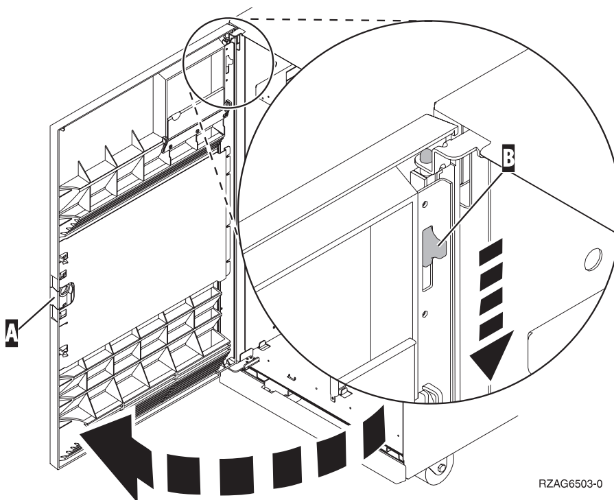
Figuur 1. Het voorpaneel openen (5074, 5094, 5095, 830, 840, 870, 890)
