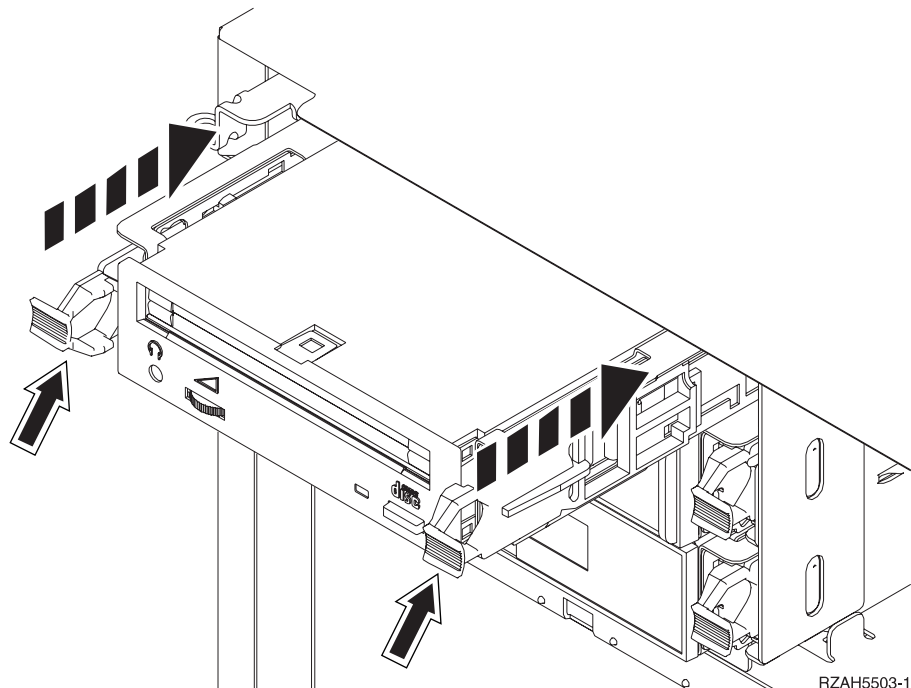
Figuur 3. Het CD-ROM- of bandstation installeren.
