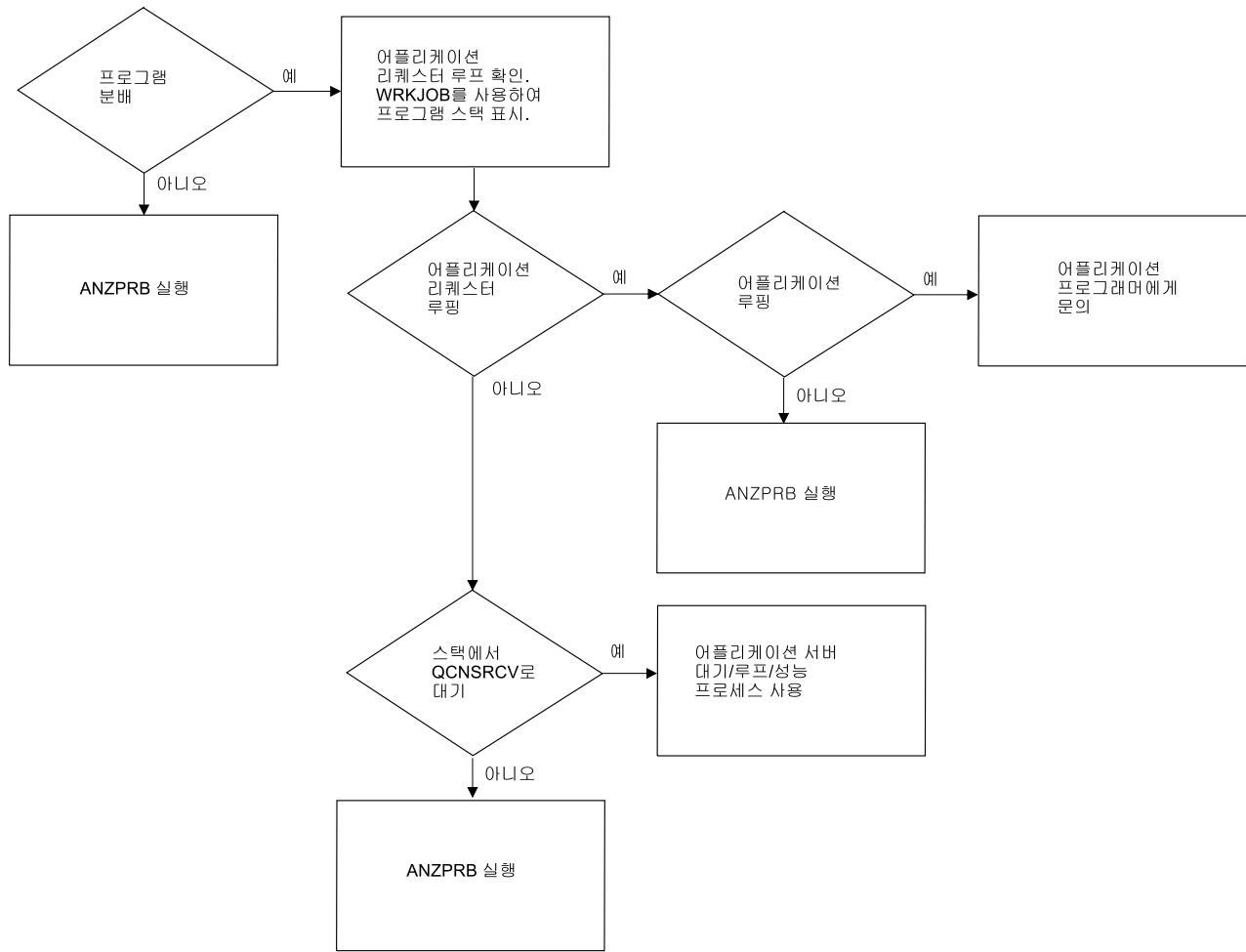
그림 16. 어플리케이션 리퀘스터 상의 대기, 루프 또는 성능 문제점 해결
