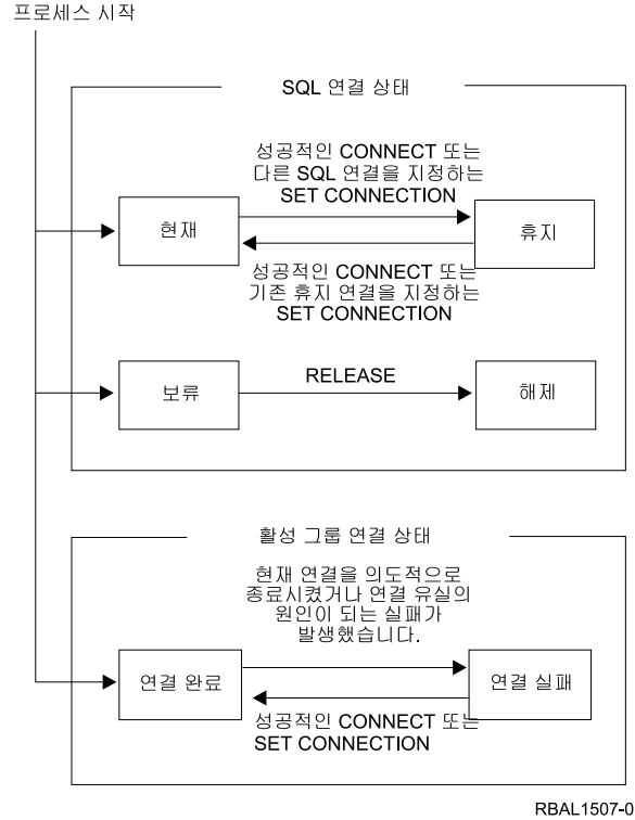
그림 21. 어플리케이션 지향의 분산 작업 단위 연결 및 활성 그룹 연결 상태 트랜지션
