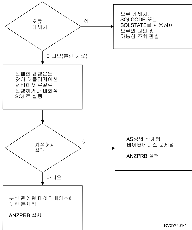
그림 15. 부정확한 출력 문제점 해결
