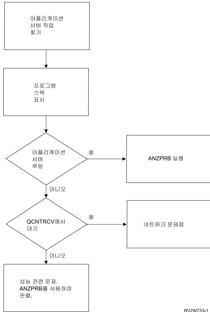
그림 17. 어플리케이션 서버 상의 대기, 루프 또는 성능 문제점 해결.
