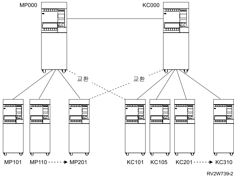
그림 12. 대체 네트워크 경로
