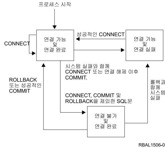
그림 20. 리모트 작업 단위 활성화 그룹 연결 상태 트랜지션
