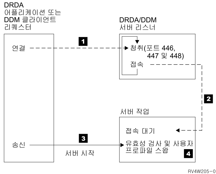
그림 11. DRDA/DDM TCP/IP 서버
