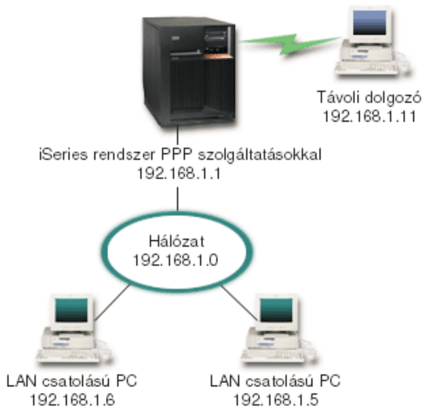
Ábra: 2. A távoli kliensek kapcsolódása az iSeries szerverhez
