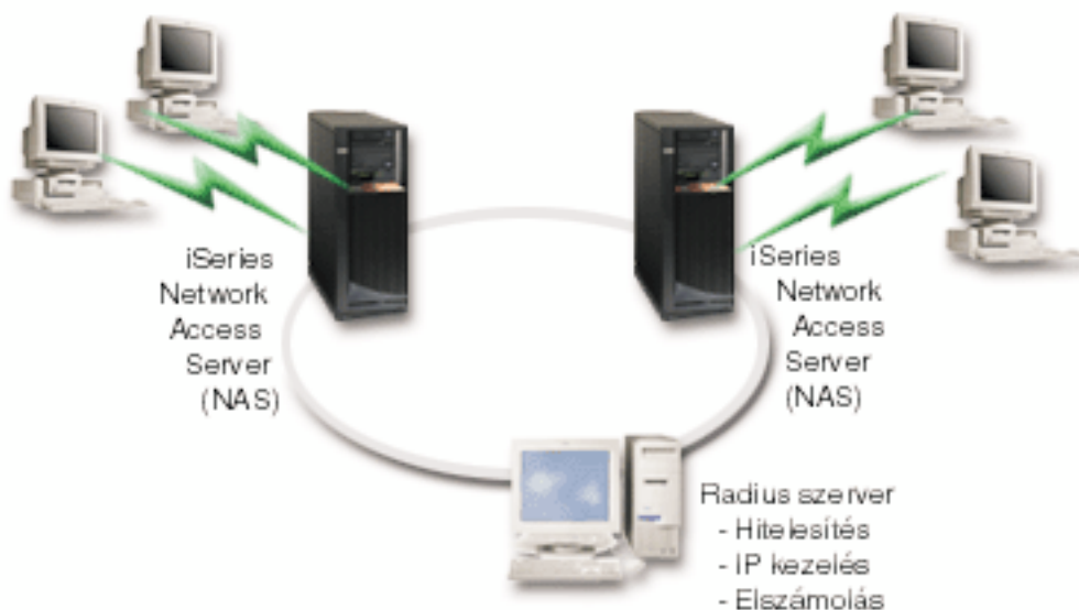
Ábra: 5. Telefonos kapcsolatok hitelesítése RADIUS szerverrel
