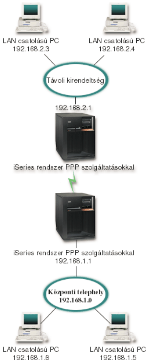
Ábra: 4. A vállalati és a távoli hálózatok összekapcsolása modemmel
